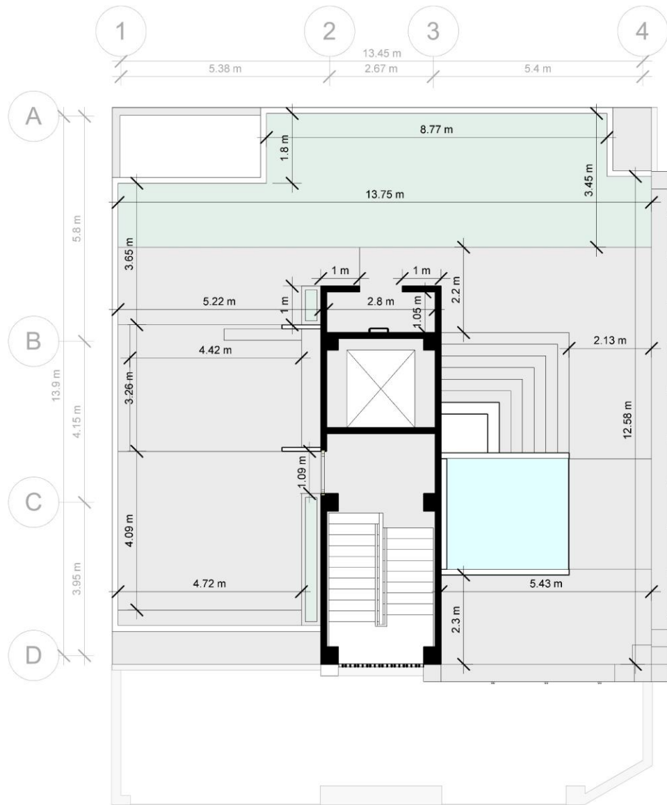
پلان مبلمان و اندازه گذاری بام
