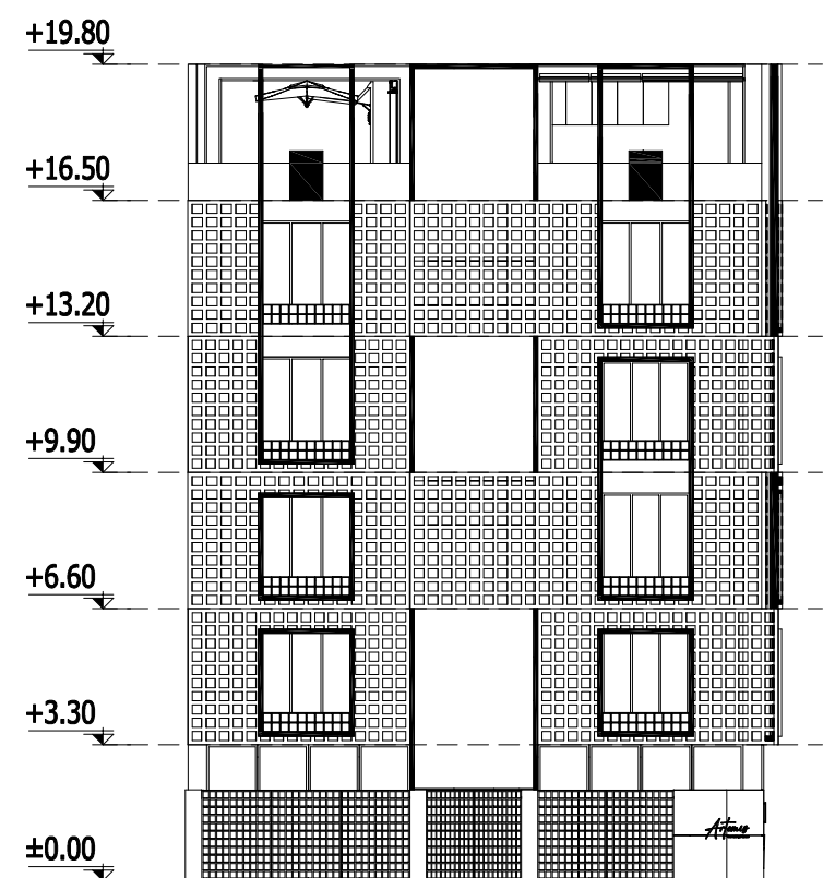
نمای شمالی
