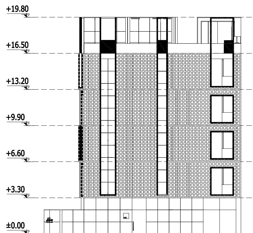
نمای شرقی
