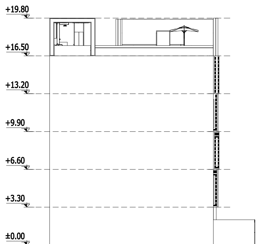
نمای غربی
