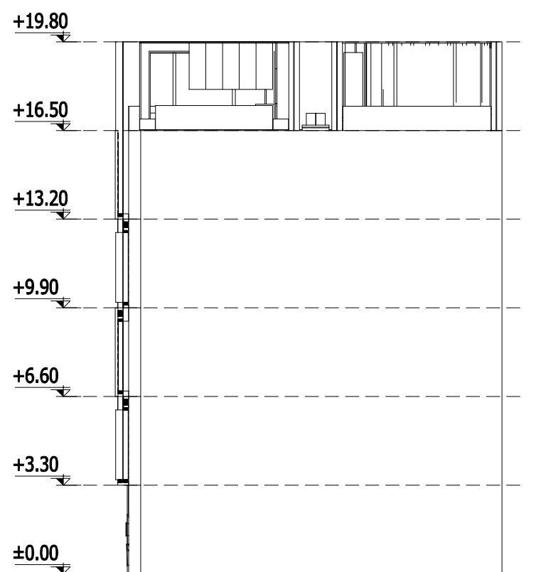
نمای جنوبی
