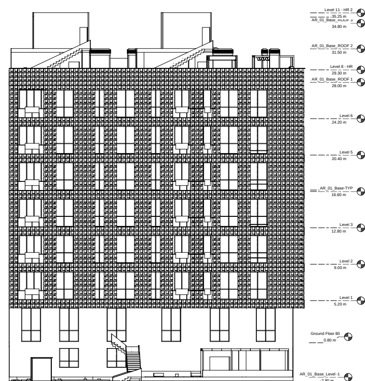
طراحی نما (جنوبی)
