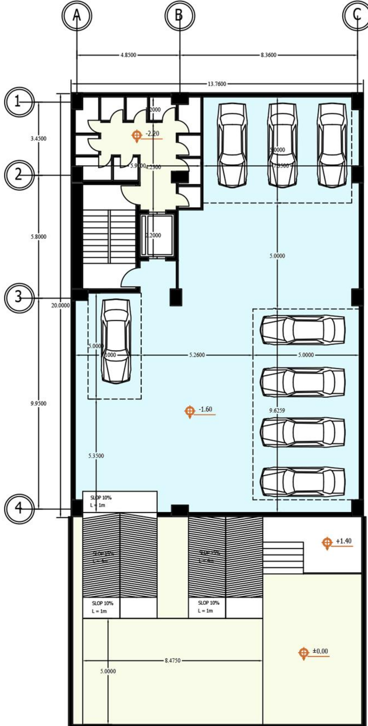
پلان اندازه گذاری طبقه زیرزمین
