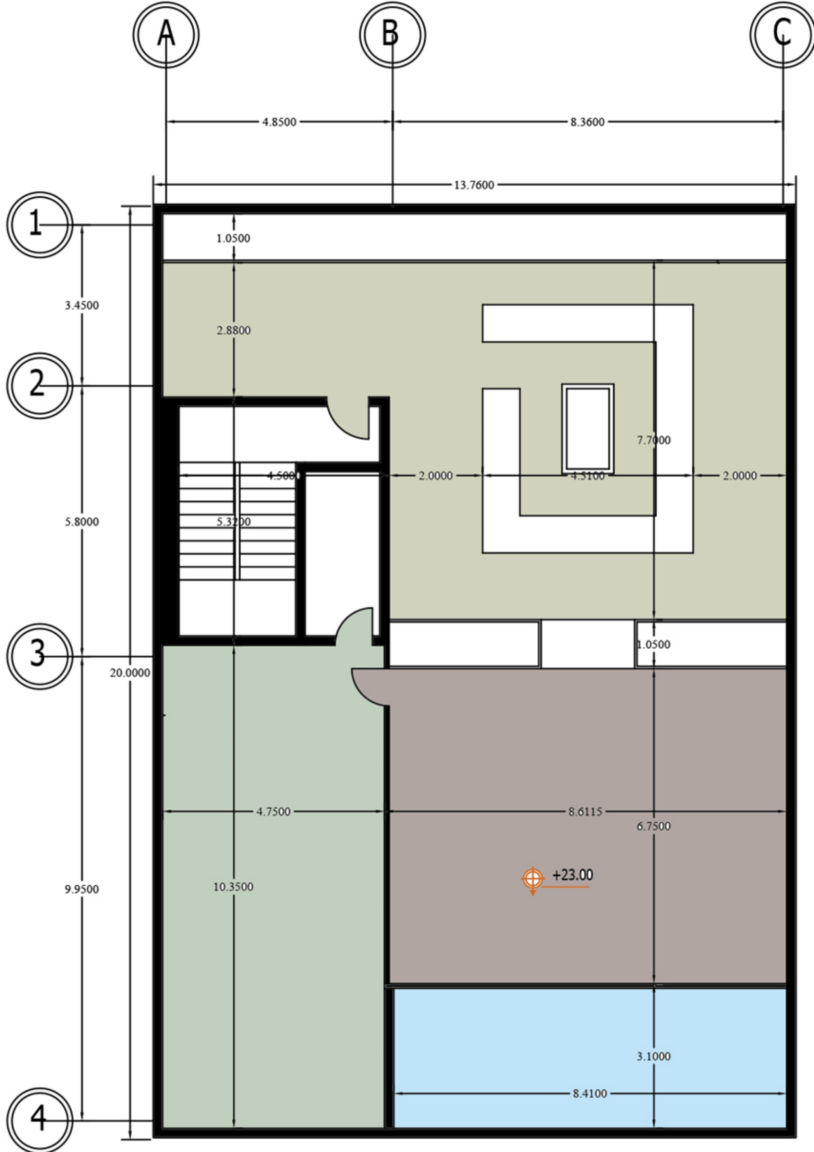
پلان اندازه گذاری طبقه بام
