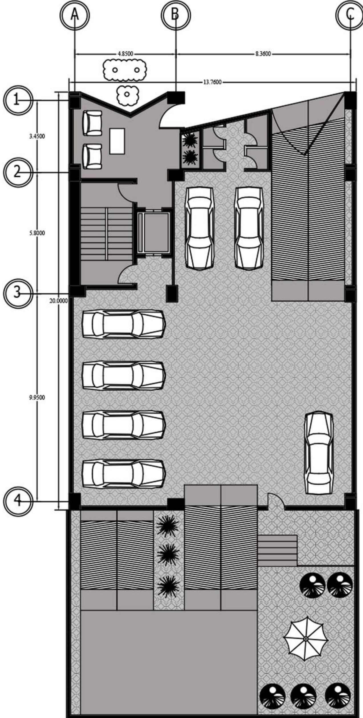
پلان مبلمان طبقه همکف
