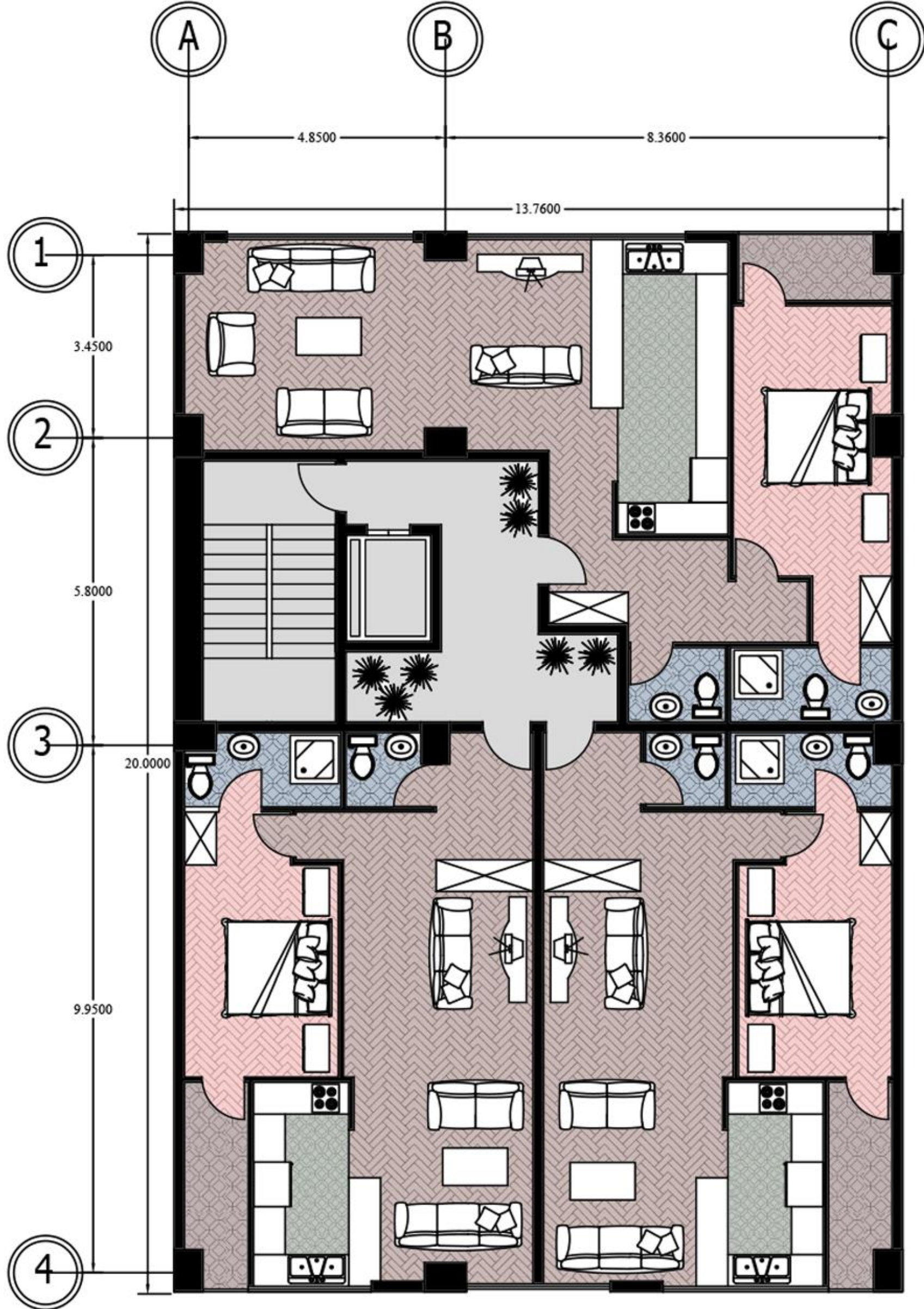
پلان مبلمان تیپ طبقات
