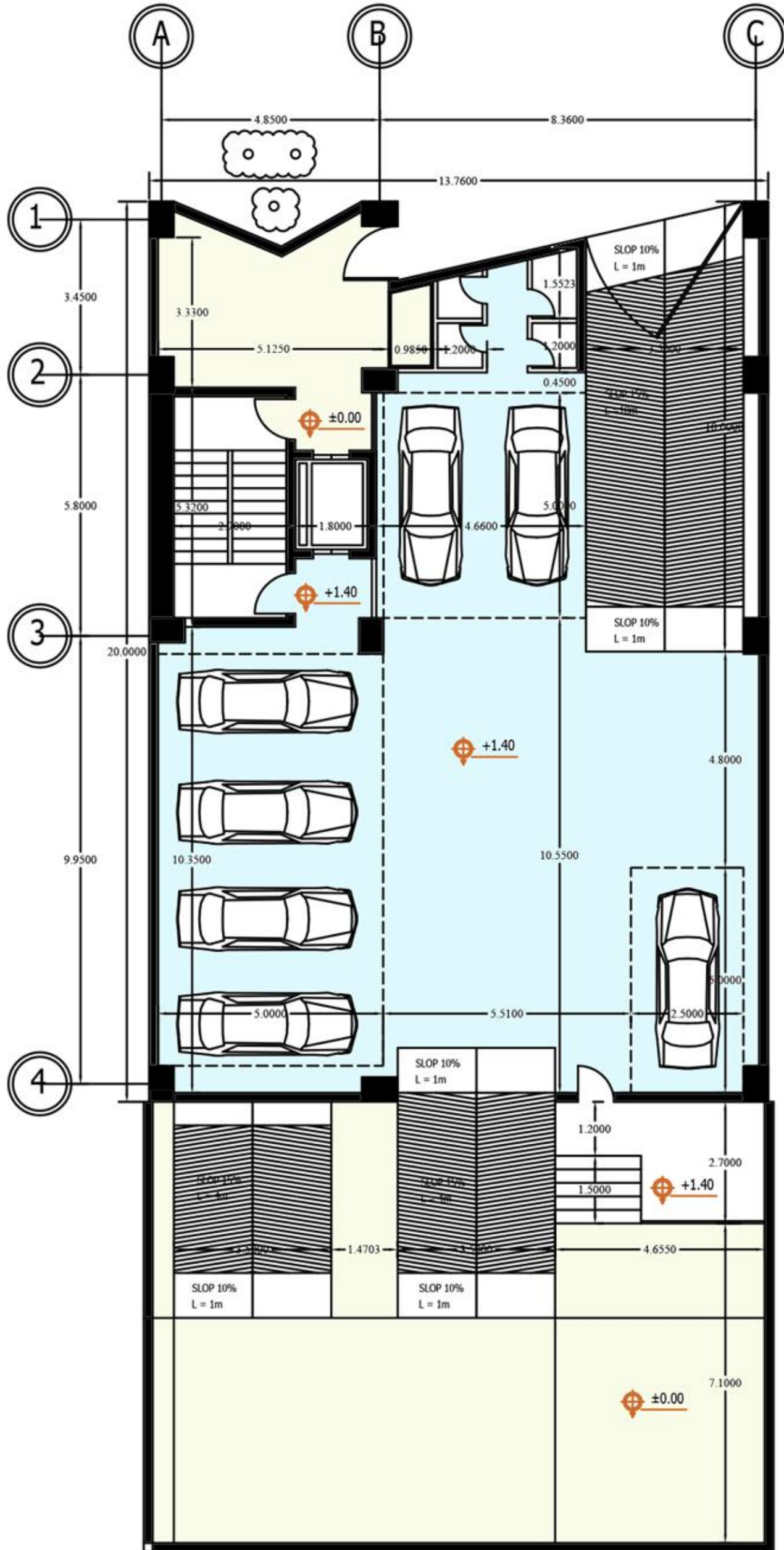
پلان اندازه گذاری طبقه همکف
