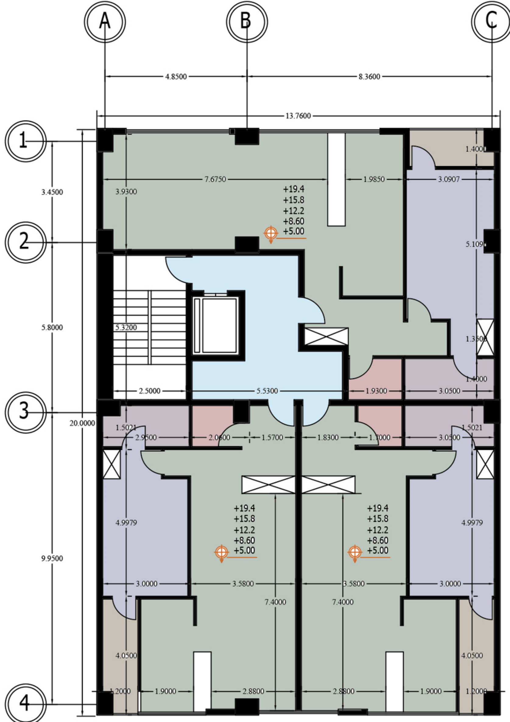
پلان اندازه گذاری تپ طبقات
