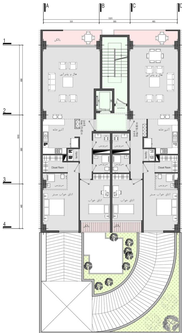
پلان تیپ طبقات پلان میلمان
