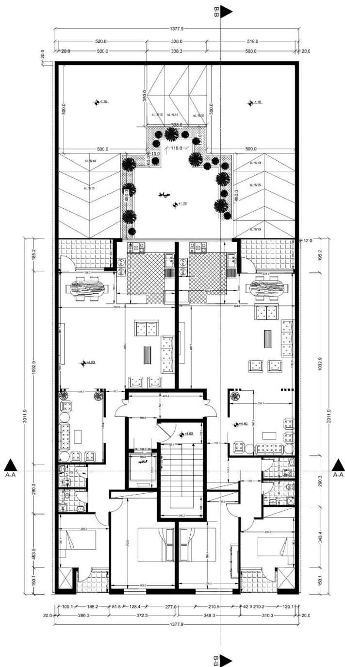
پلان طبقه اول sc:1.100
