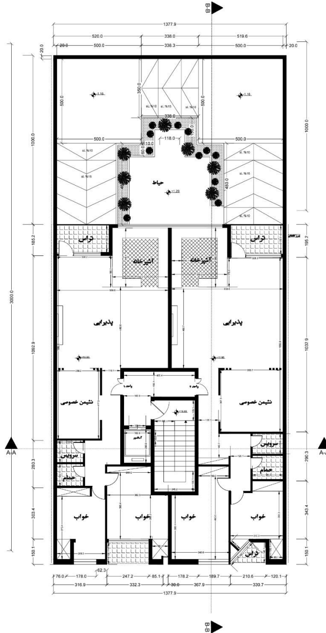
پلان طبقه پنجم sc:1.100
