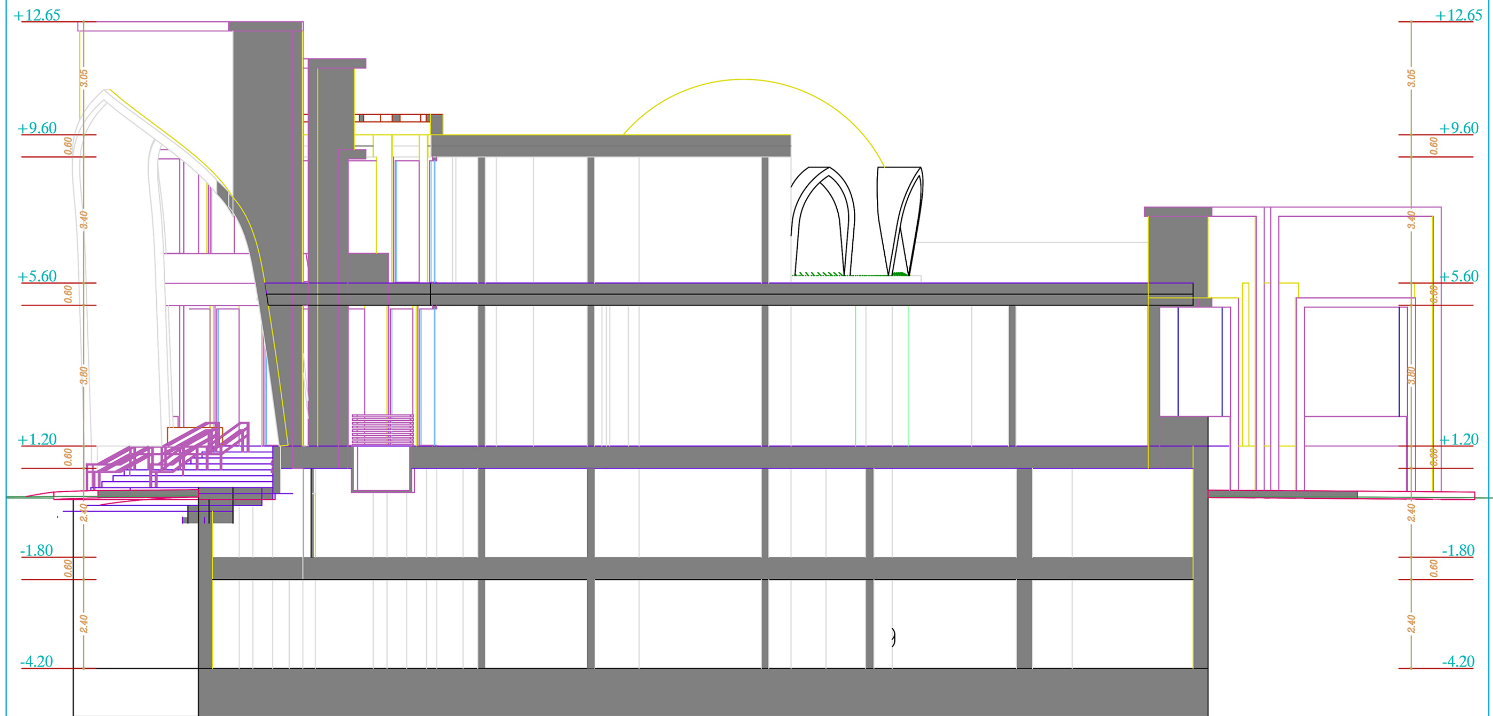
برش از شمال بنا
