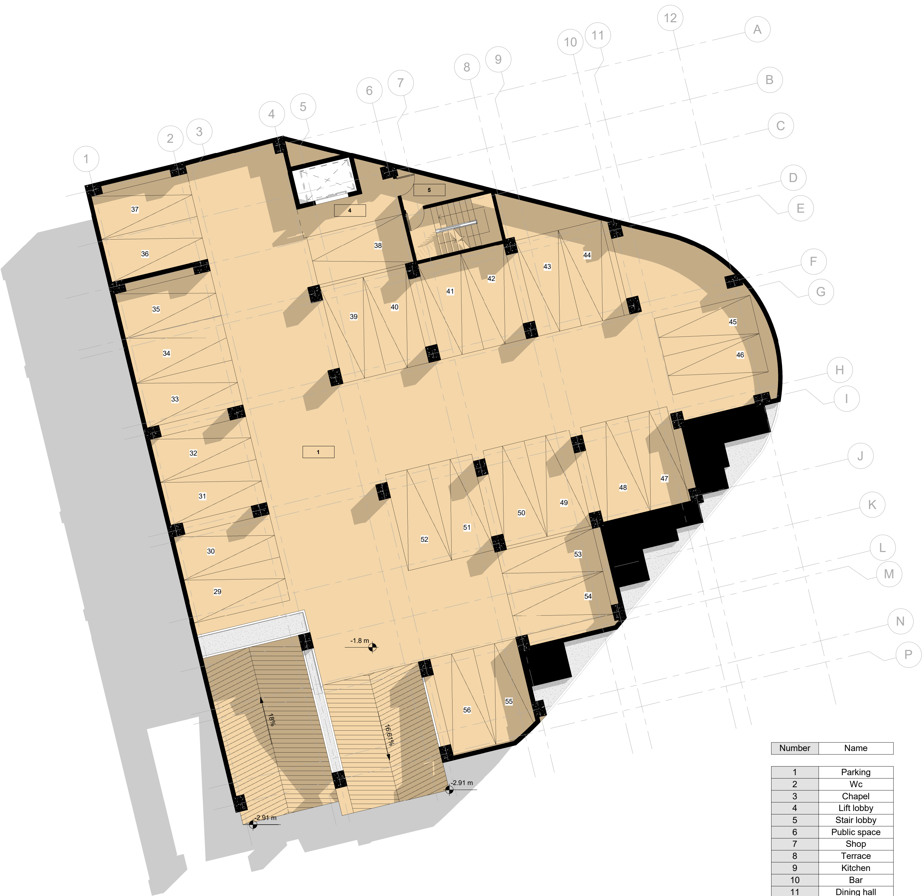
1 Basement 1 : 100
