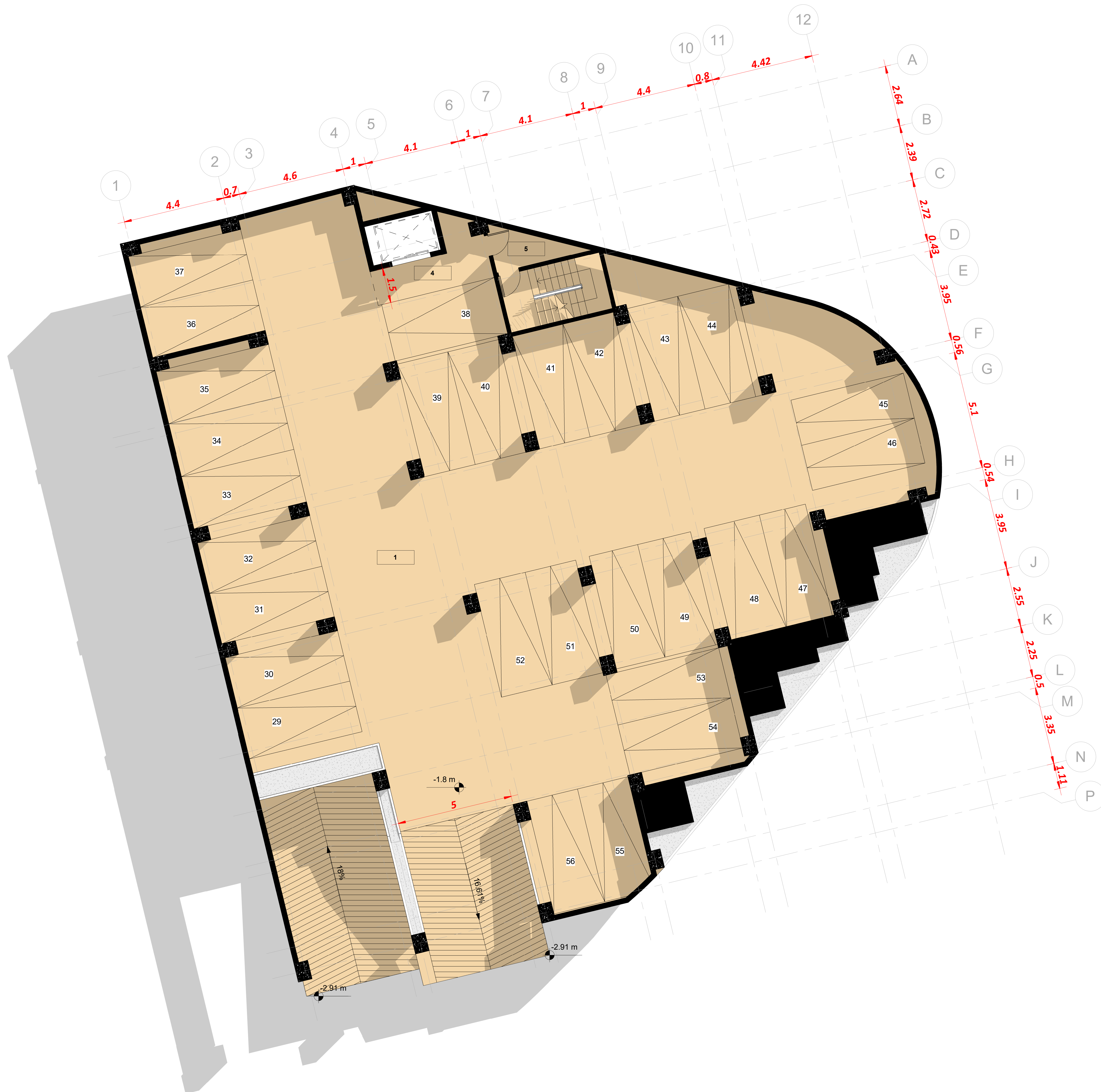
1 Annotation basement 1 : 100
