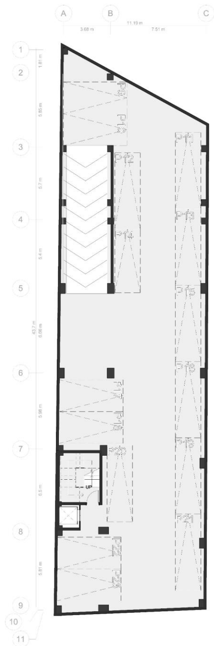
پلان مبلمان و اندازه گذاری طبقه منفی ۲
