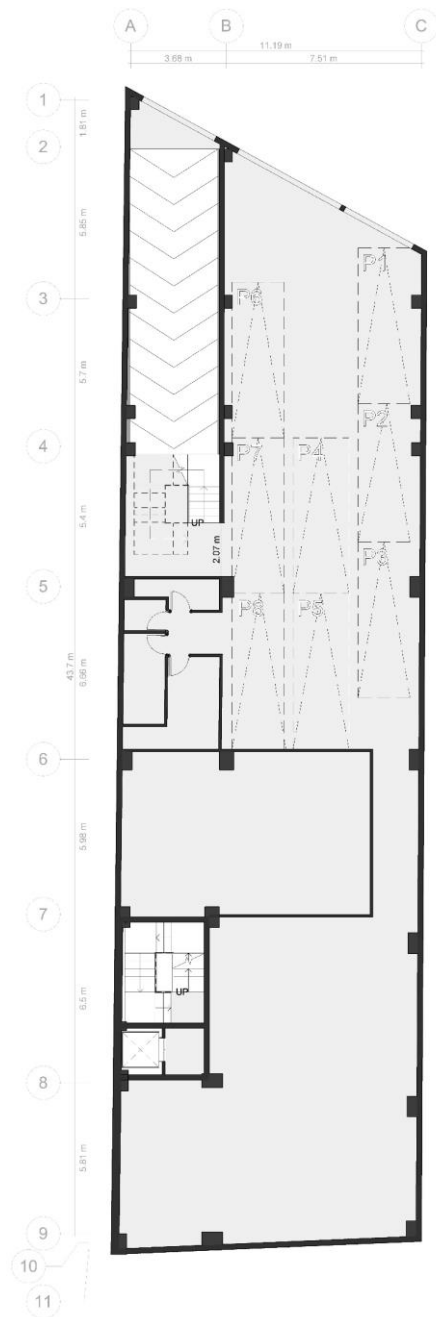
پلان مبلمان و اندازه گذاری طبقه منفی ۱
