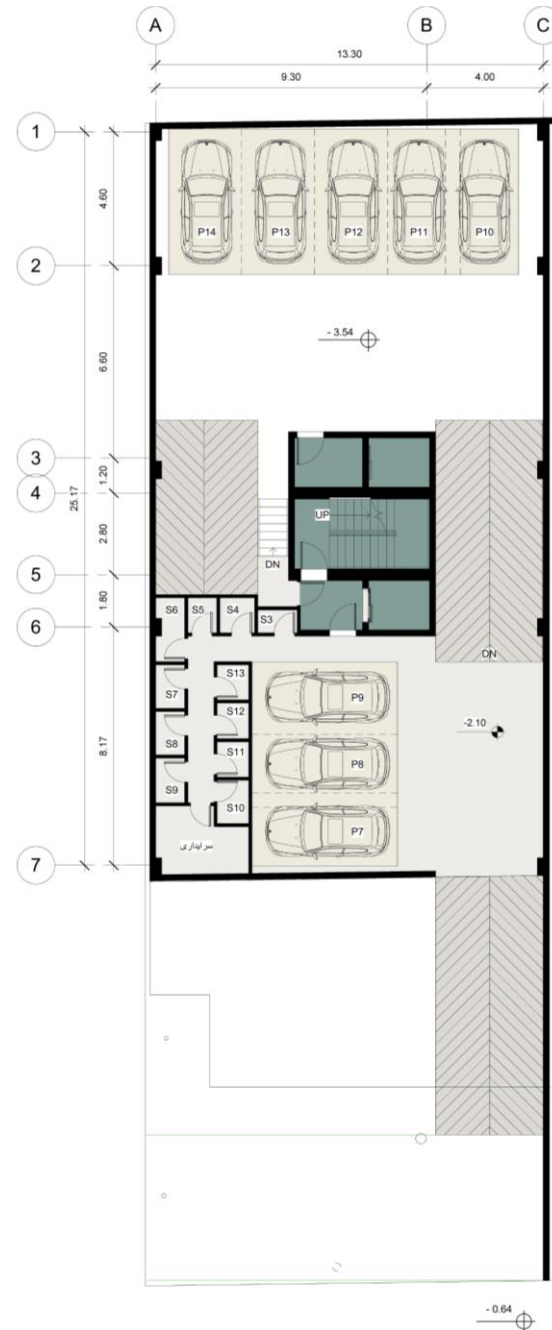
پلان ۱- (۸/۲۶)
