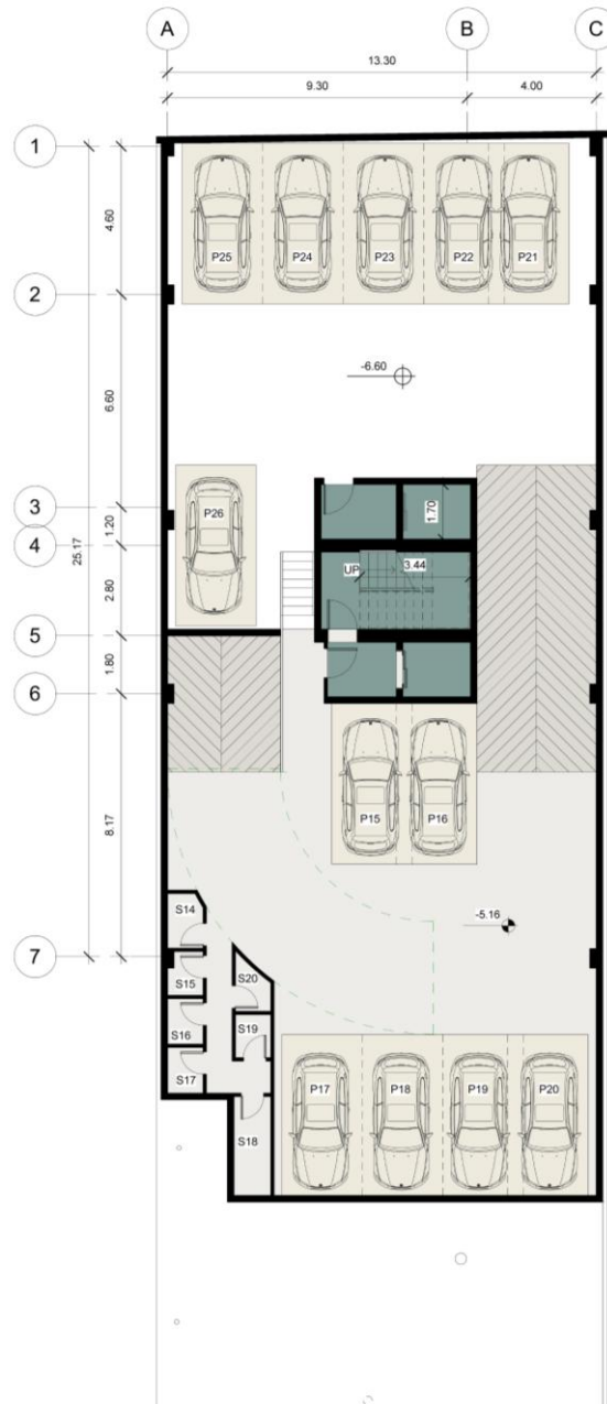
پلان ۲- (۱۲/۲۶)
