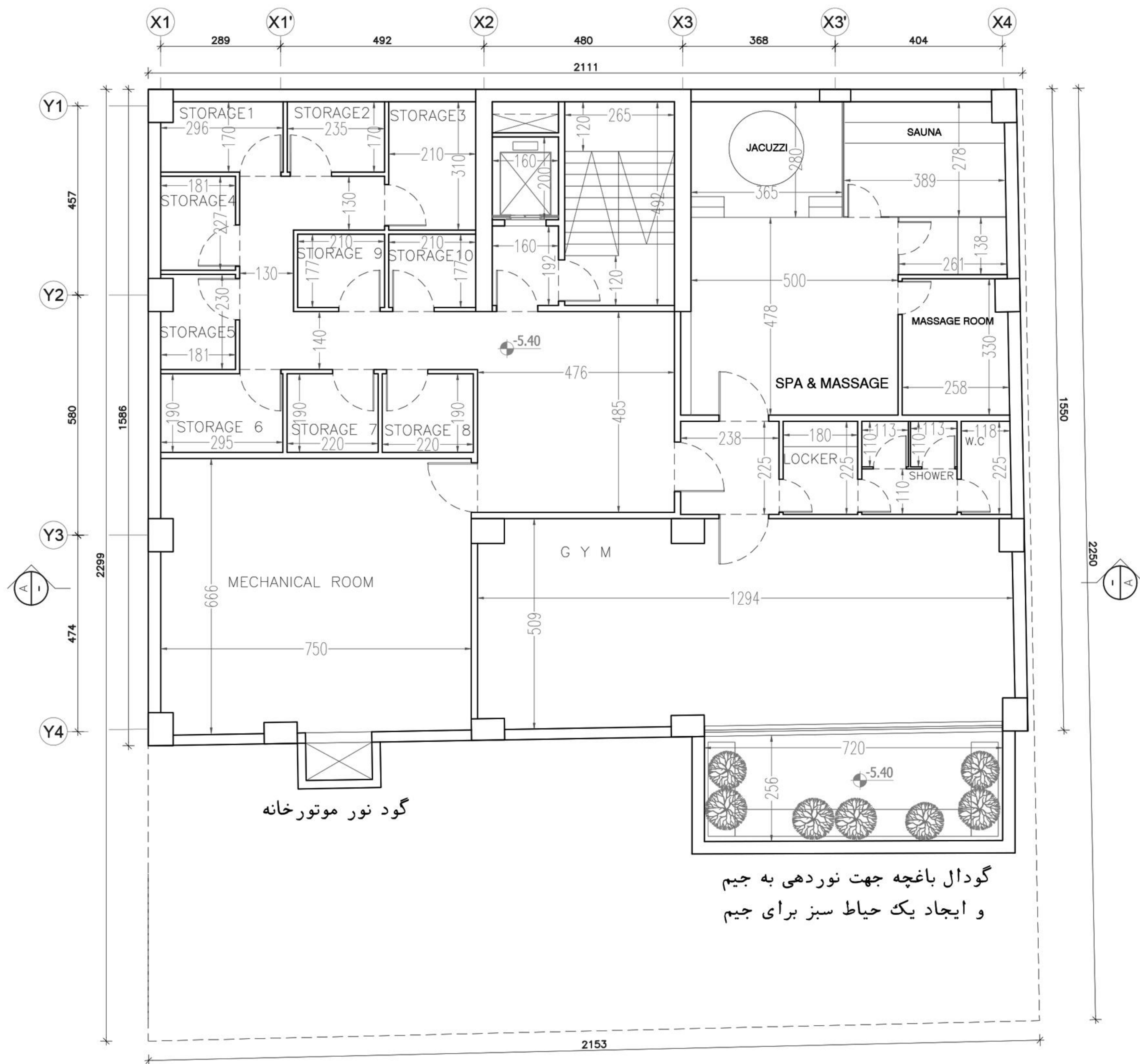
پلان اندازه گذاری طبقه منفی دو آلترناتیو اول
