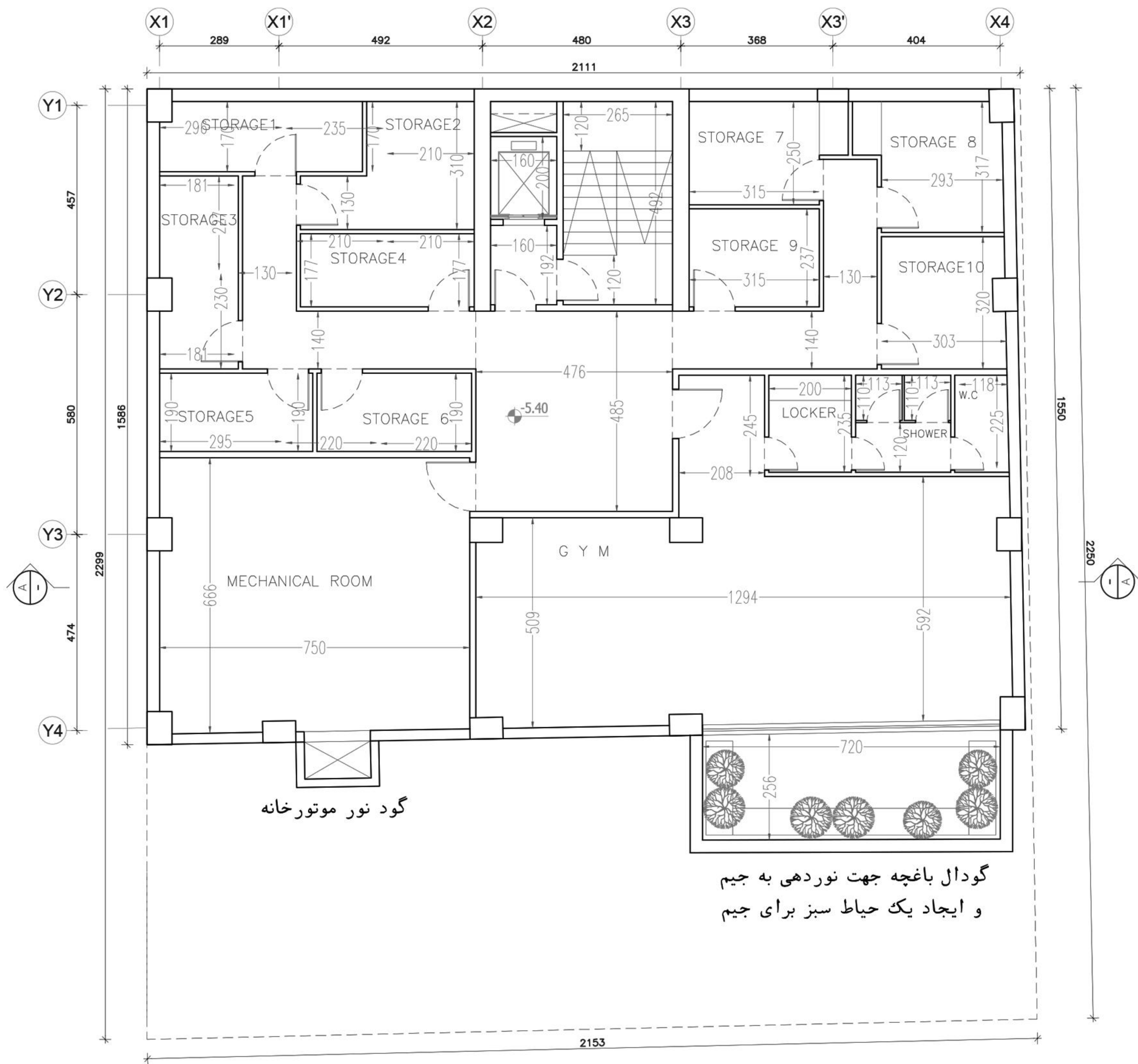
پلان اندازه گذاری طبقه منفی دو آلترناتیو سوم
