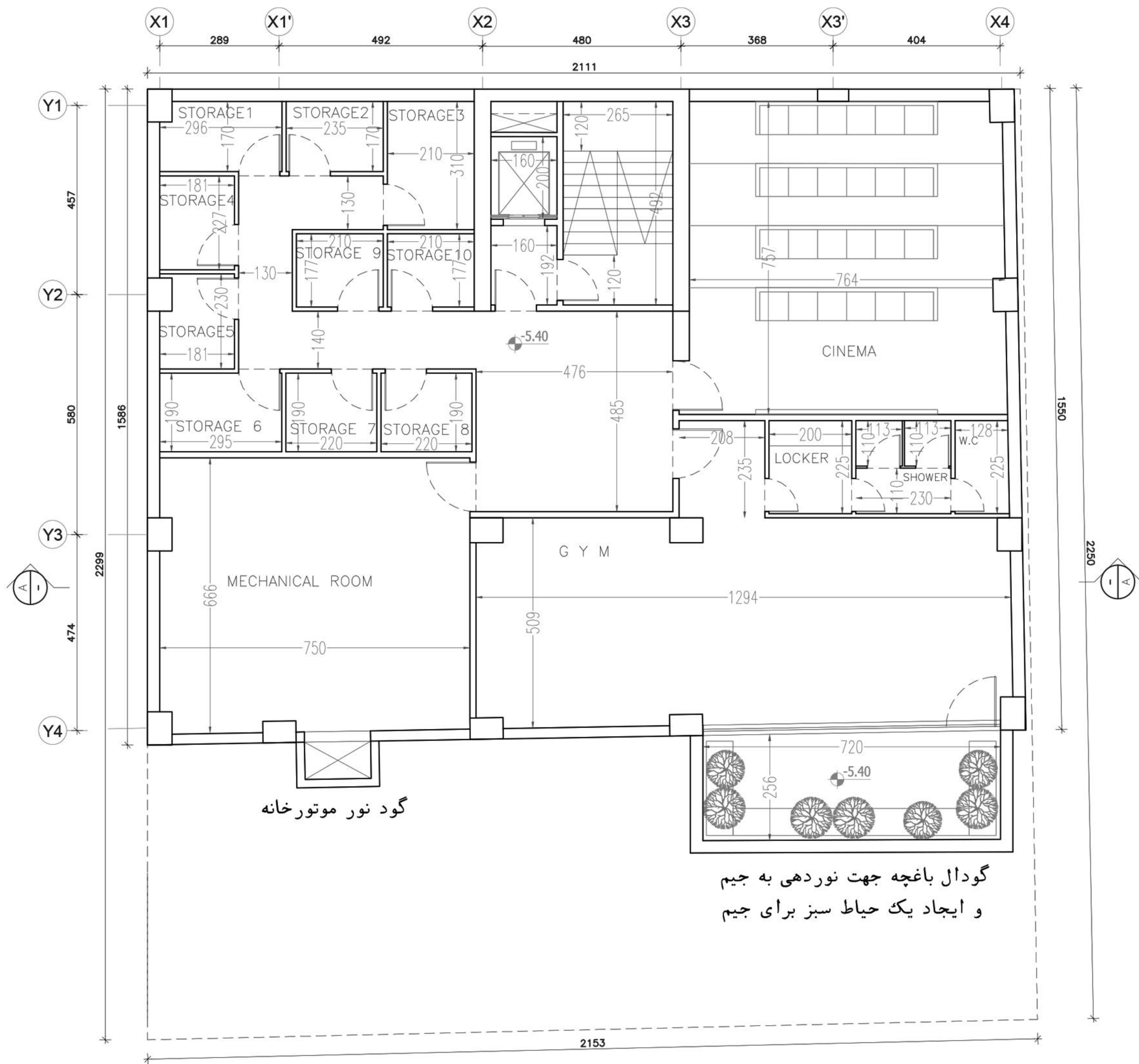
پلان اندازه گذاری طبقه منفی دو آلترناتیو دوم
