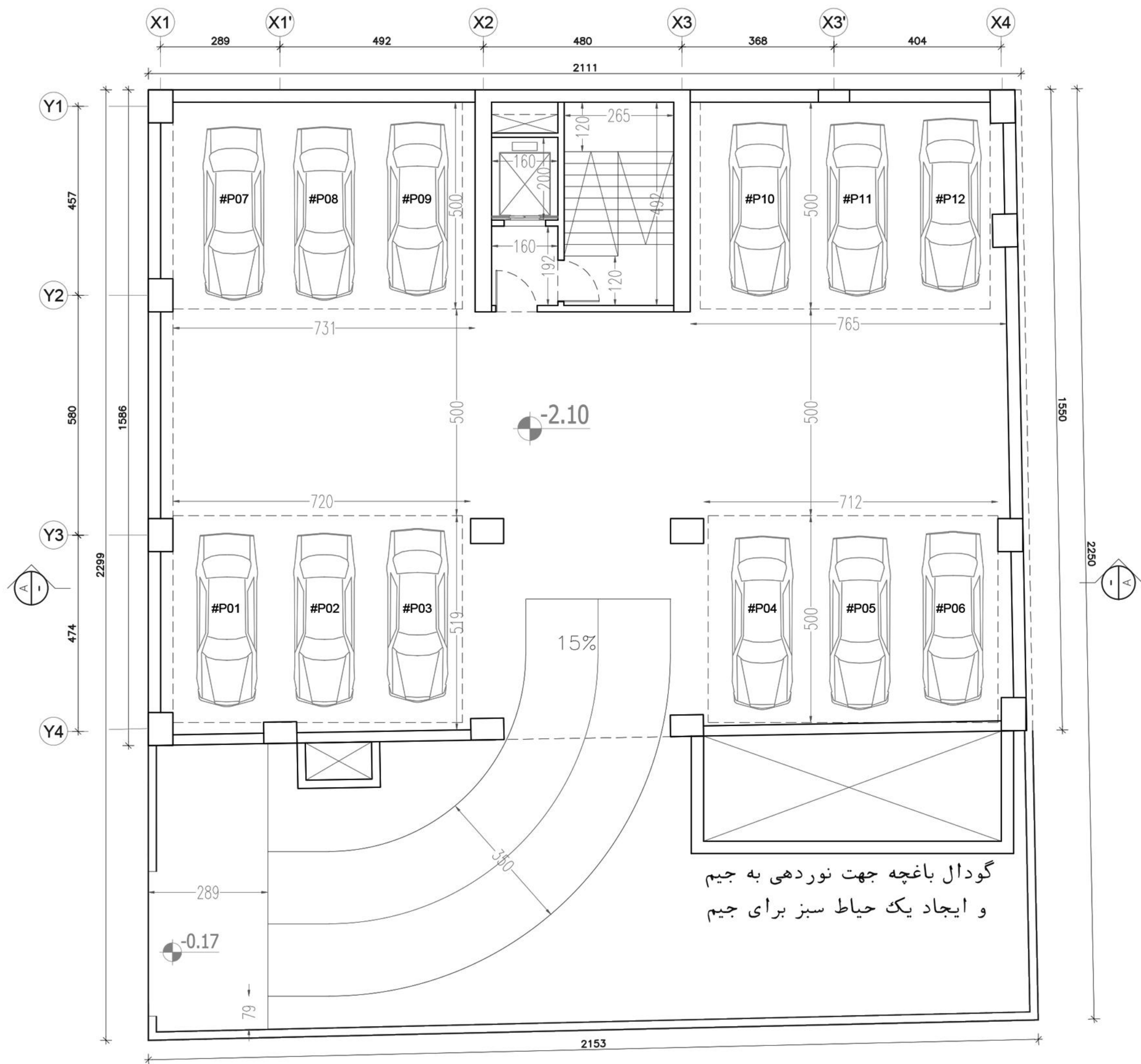
پلان اندازه گذاری طبقه منفی یک
