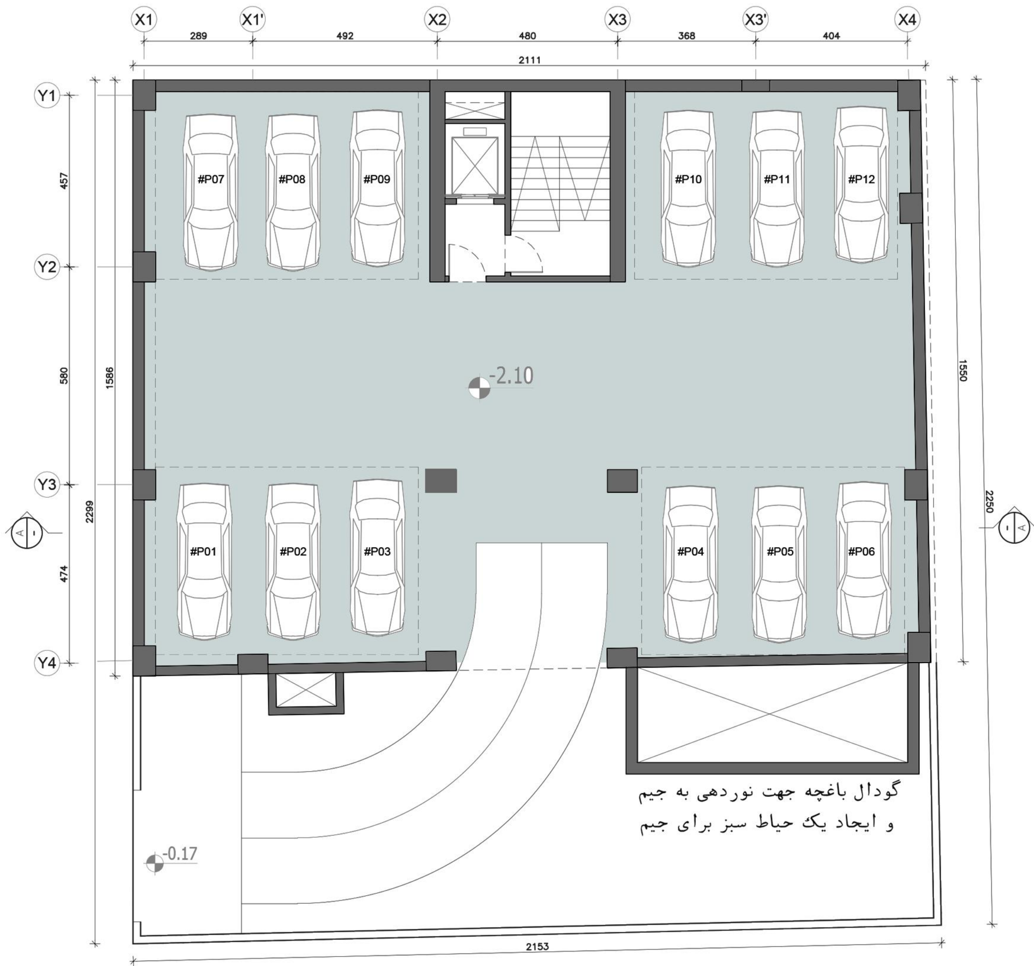
پلان مبلمان طبقه منفی یک
