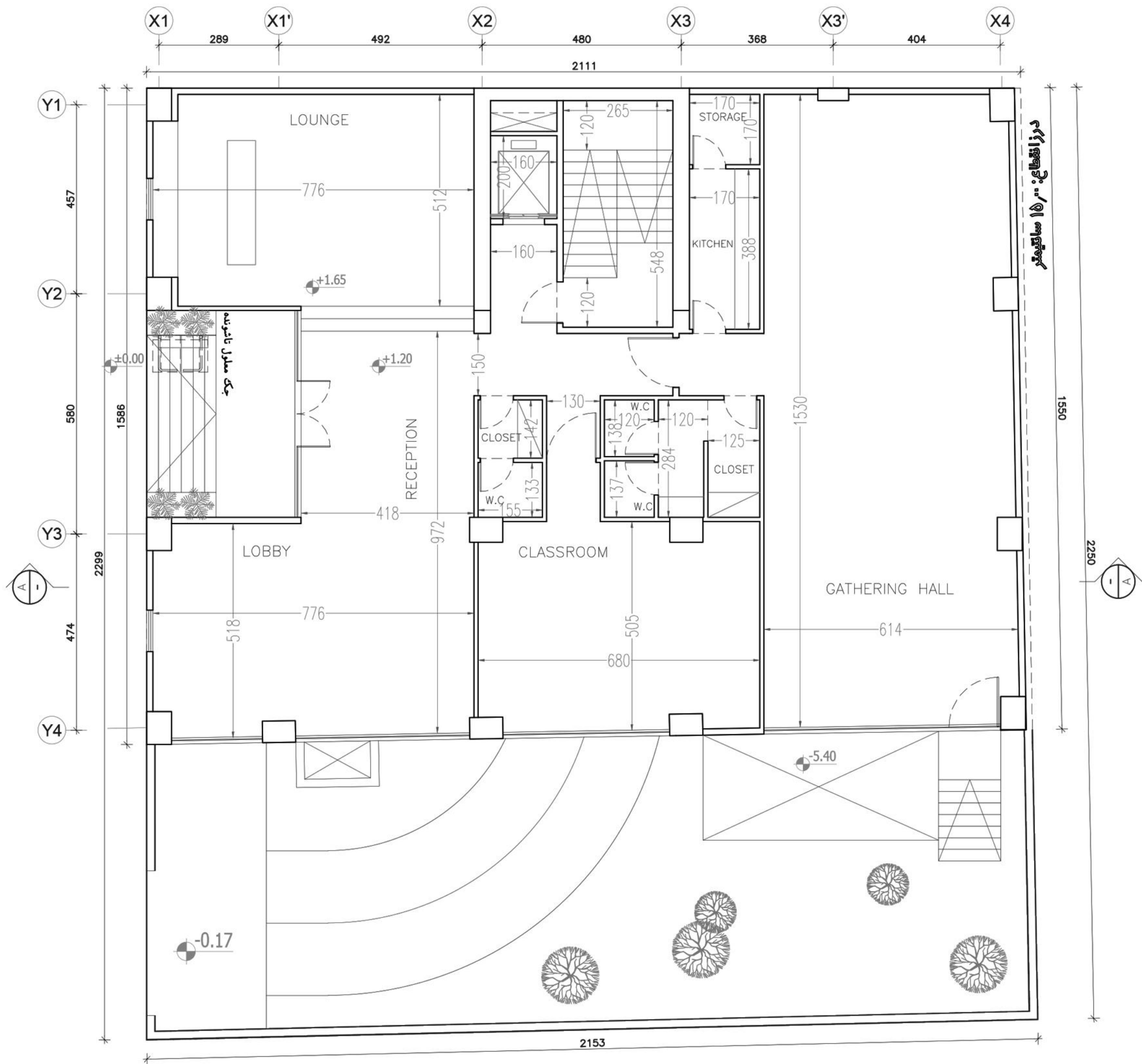
پلان اندازه گذاری طبقه همکف
