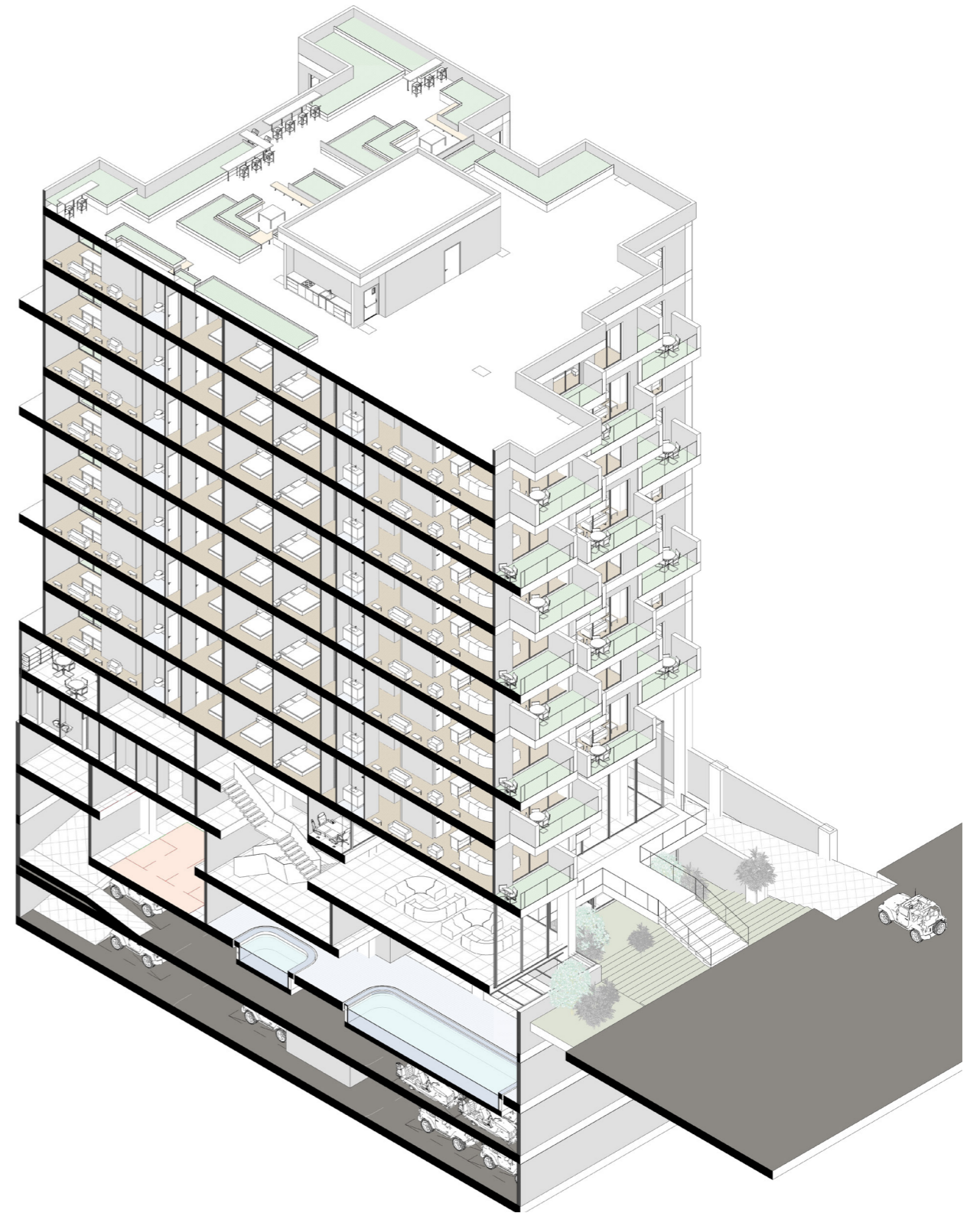
Section D-D
