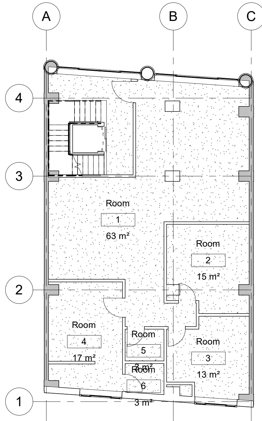
3 Level 1,4,5 Area 1 : 100
