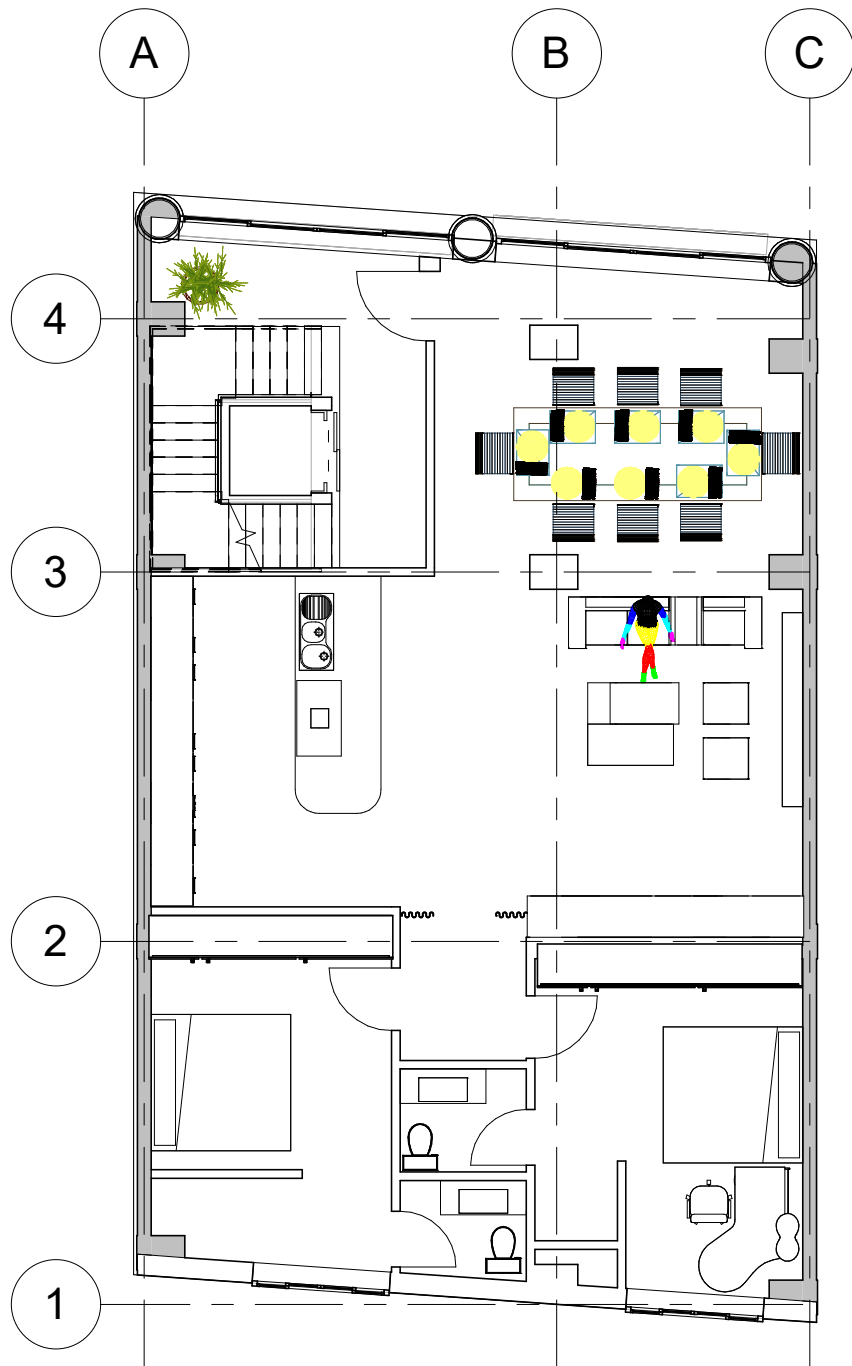
Level 2,3
