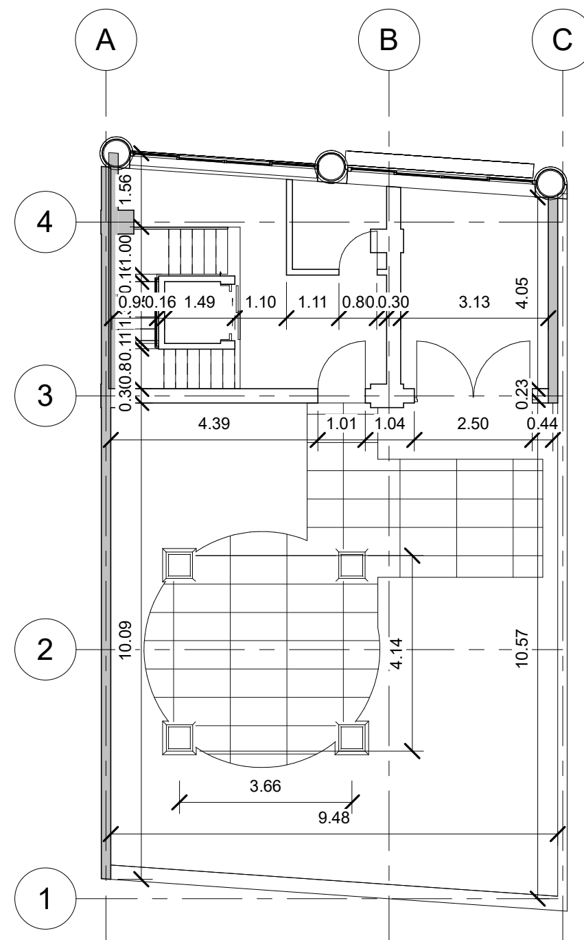
3 Level R Dim 1 : 100
