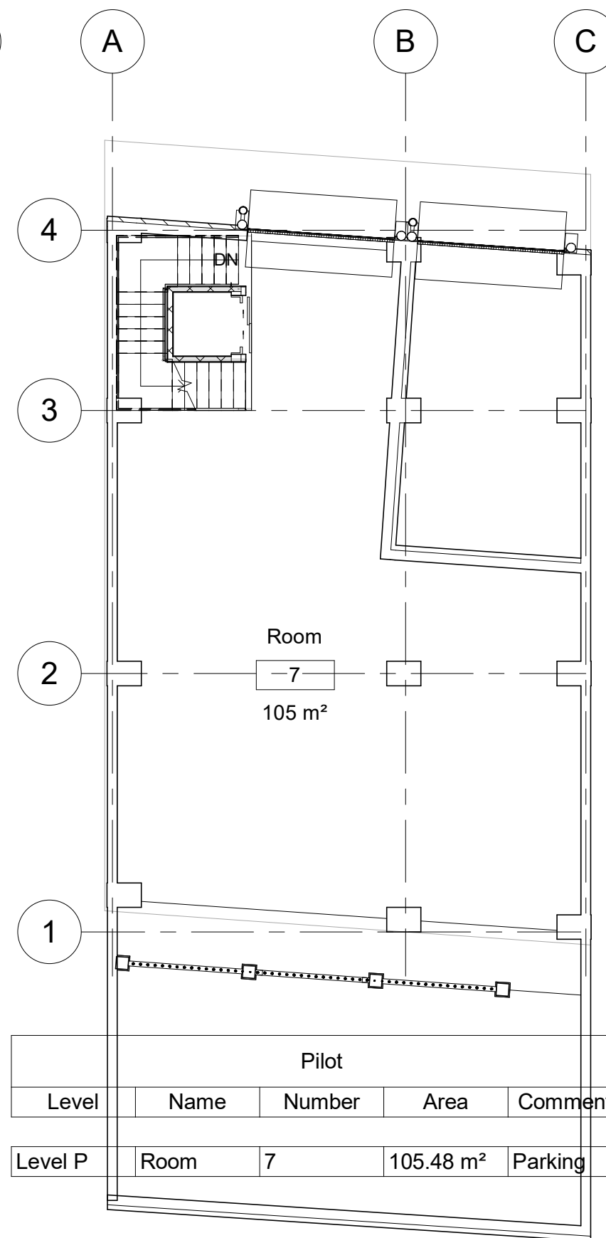
3 Level P Area 1 : 100
