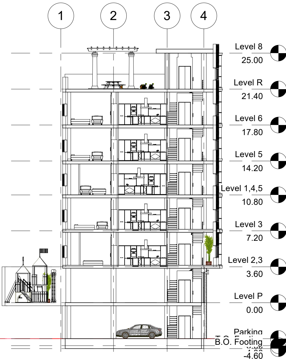
1 Section 1 1 : 200
