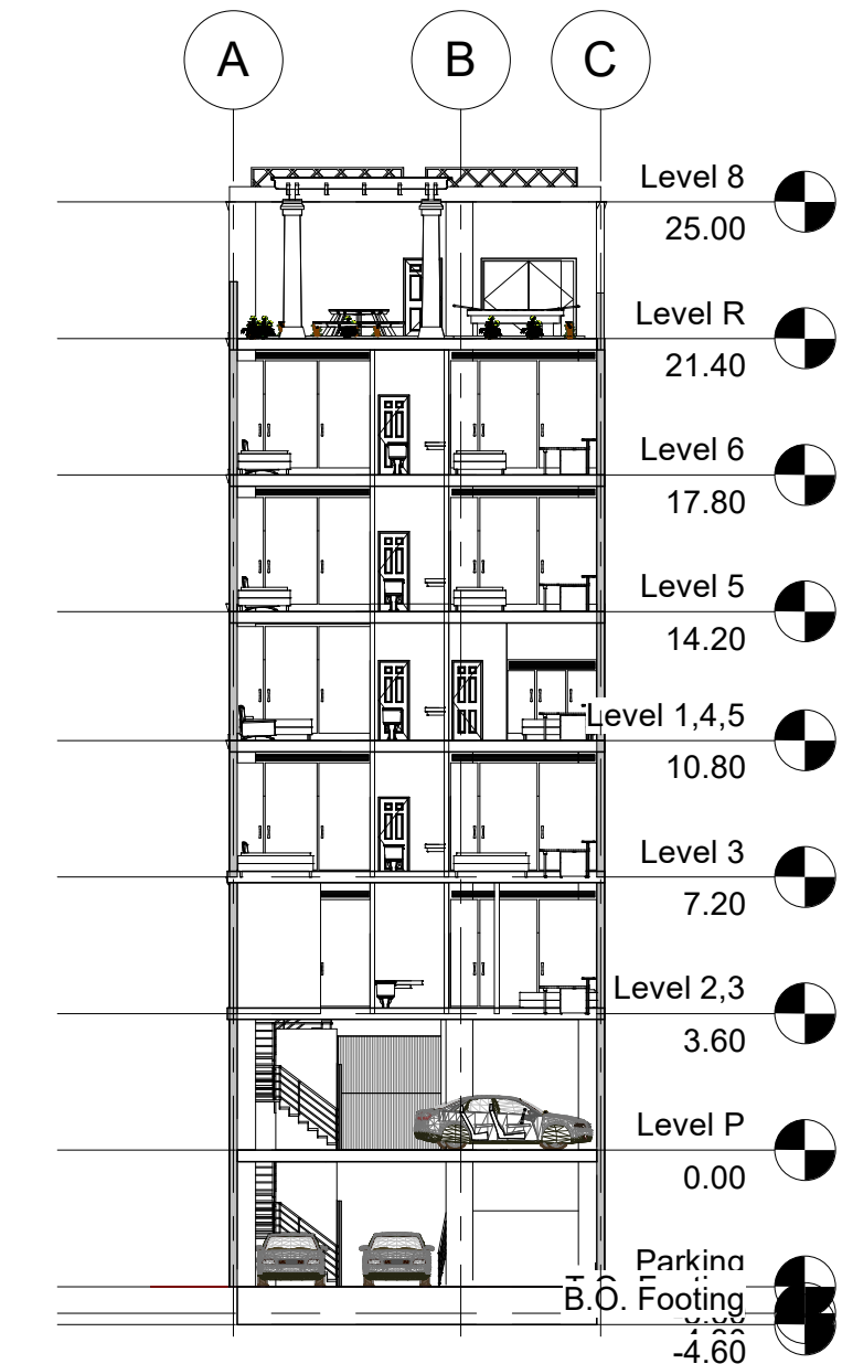
3 Section 3 1 : 200
