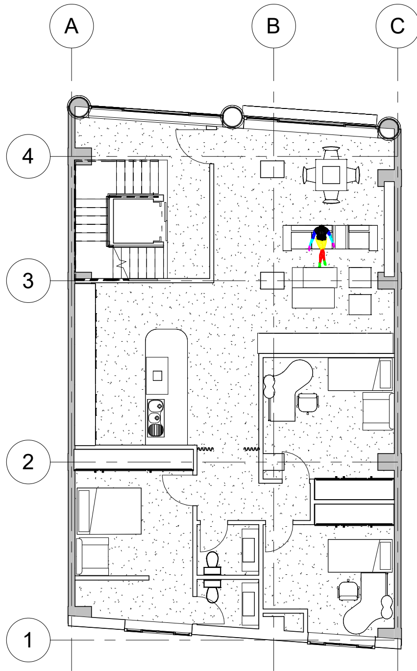
1 Level 1,4,5 1 : 100
