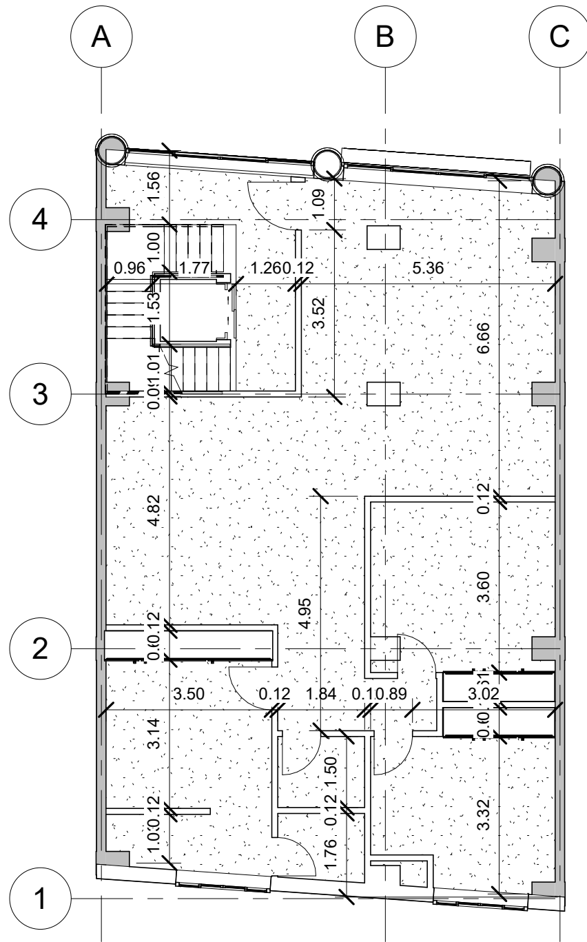
2 Level 1,4,5 Dim 1 : 100
