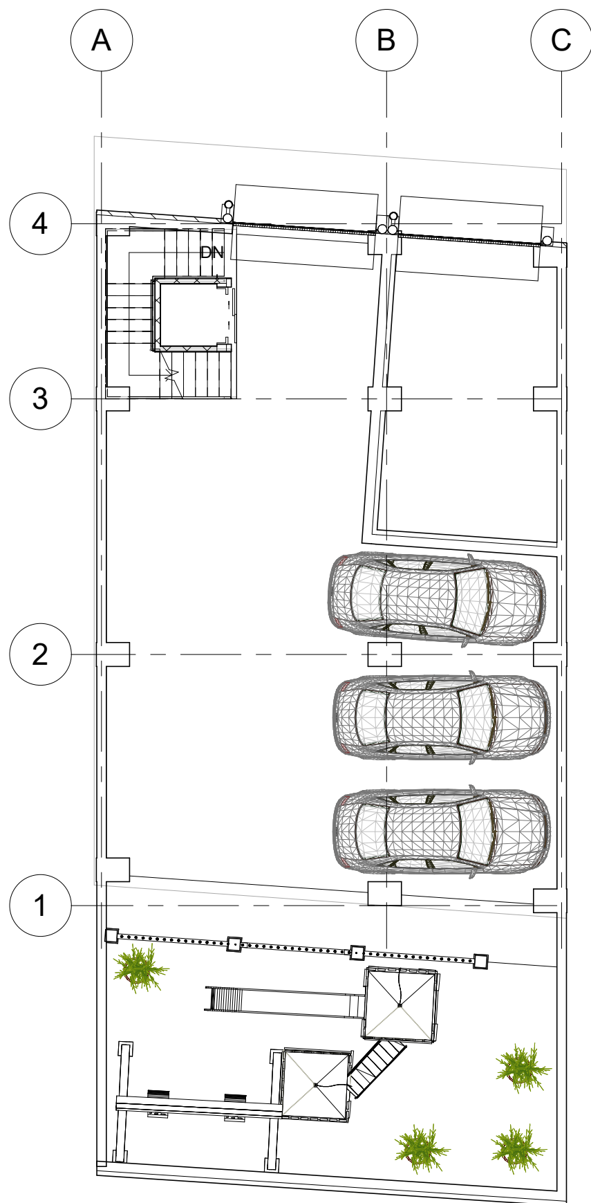
1 Level P 1 : 100
