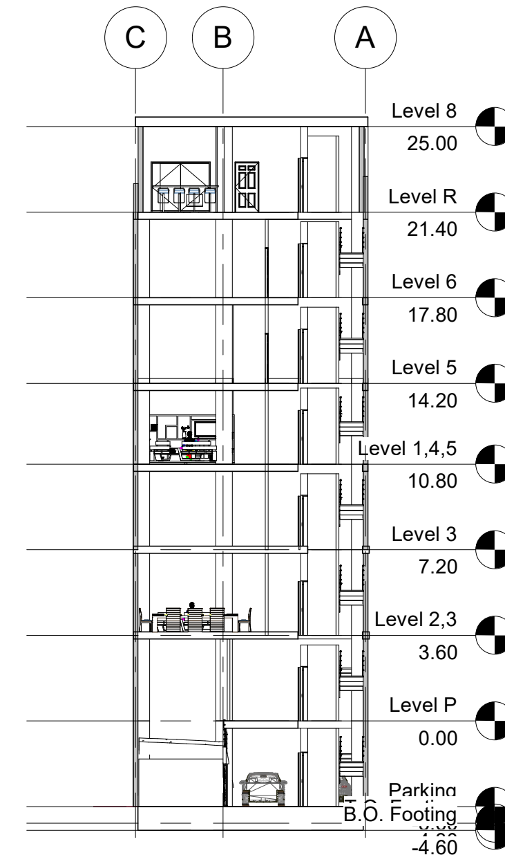
2 Section 2 1 : 200
