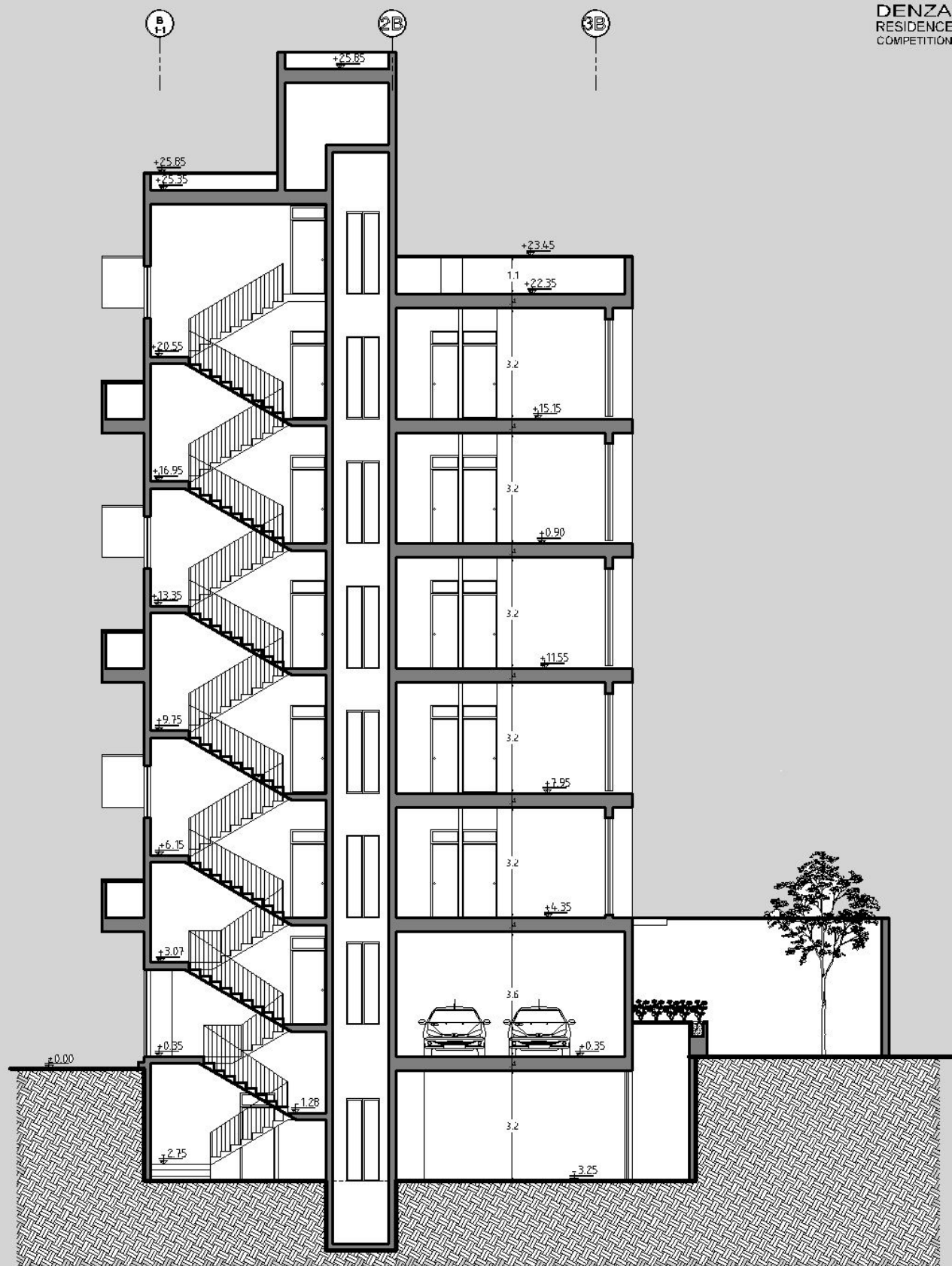
مقطع A-A
