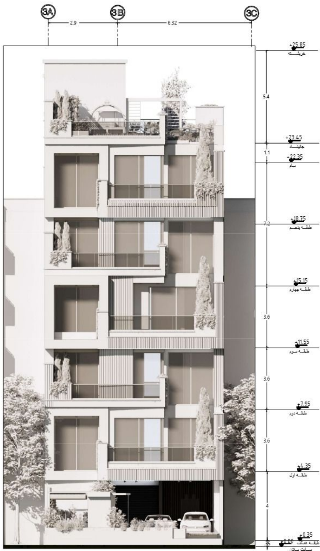
نمای جنوبی
