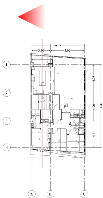
DIMENSION PLAN - L1,2,4,5
