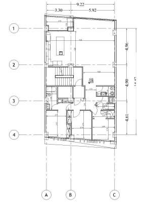
DIMENSION PLAN - L1,2,4,5
