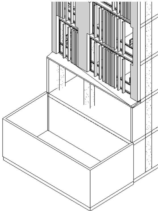
کاهش تراز حیاط تا زیر زمین جهت ارتقا کیفیت سالن اجتماعات با الهام از گودال باغچه ایرانی
