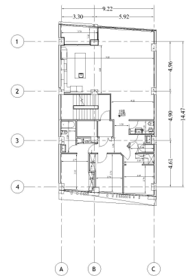
DIMENSION PLAN - L1,2,4,5
