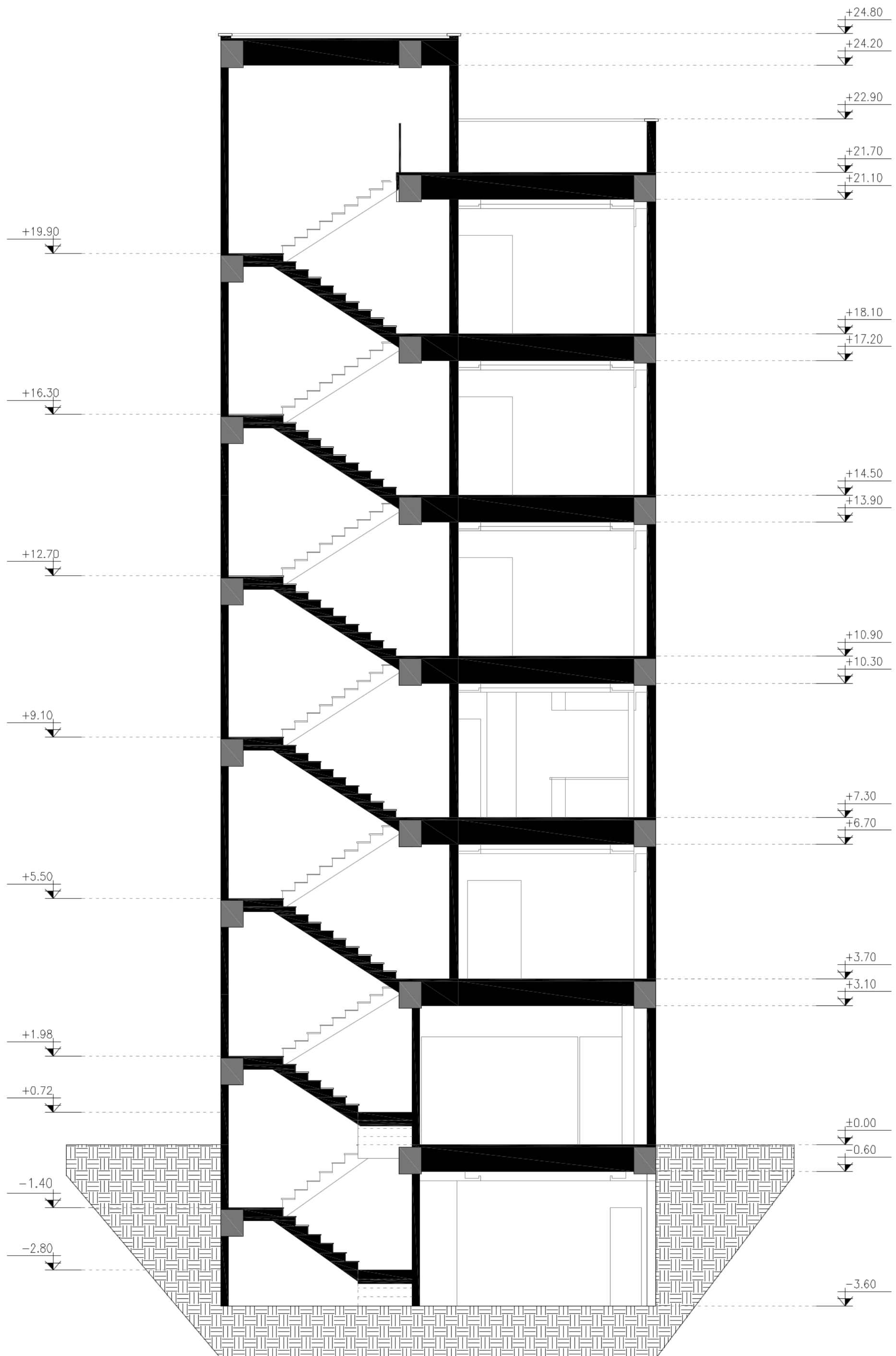
section a-a
