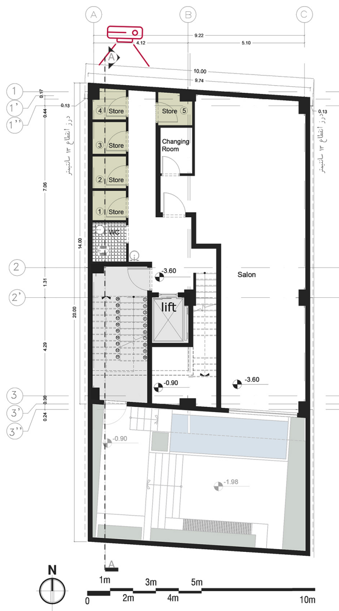
پلان مبلان زیرزمین -1
