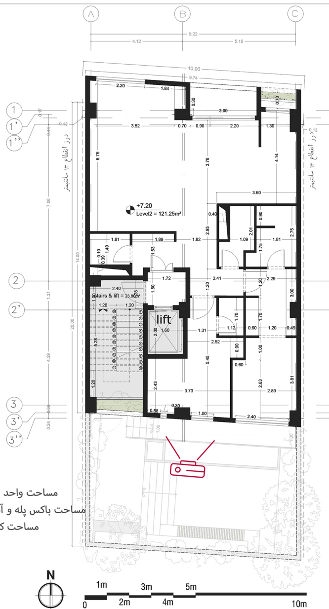
پلان اندازه گذاری طبقه ۲
