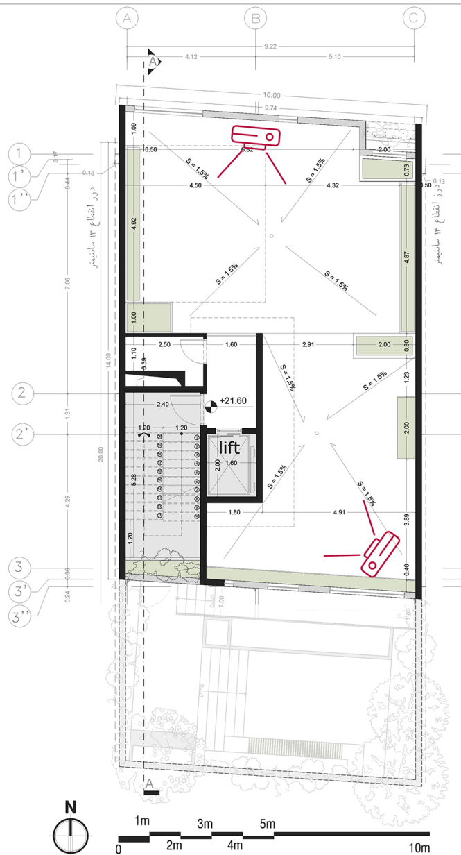
پلان اندازه گذاری بام
