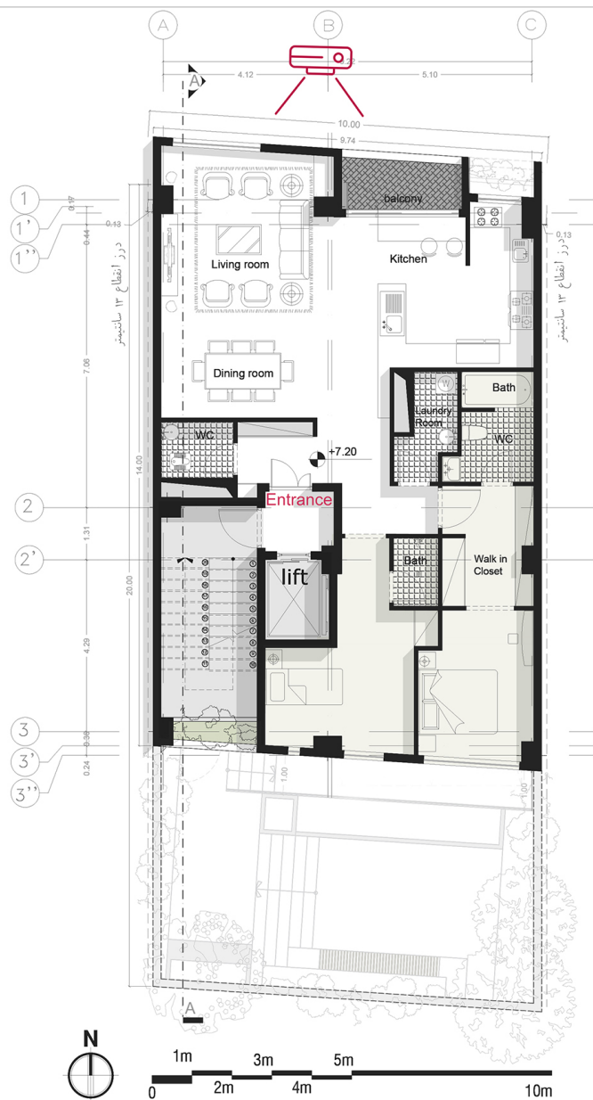
پلان مبلمان طبقه ۲
