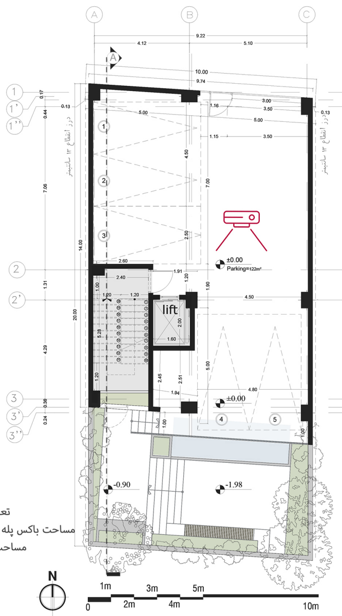
پلان اندازه گذاری همکف
