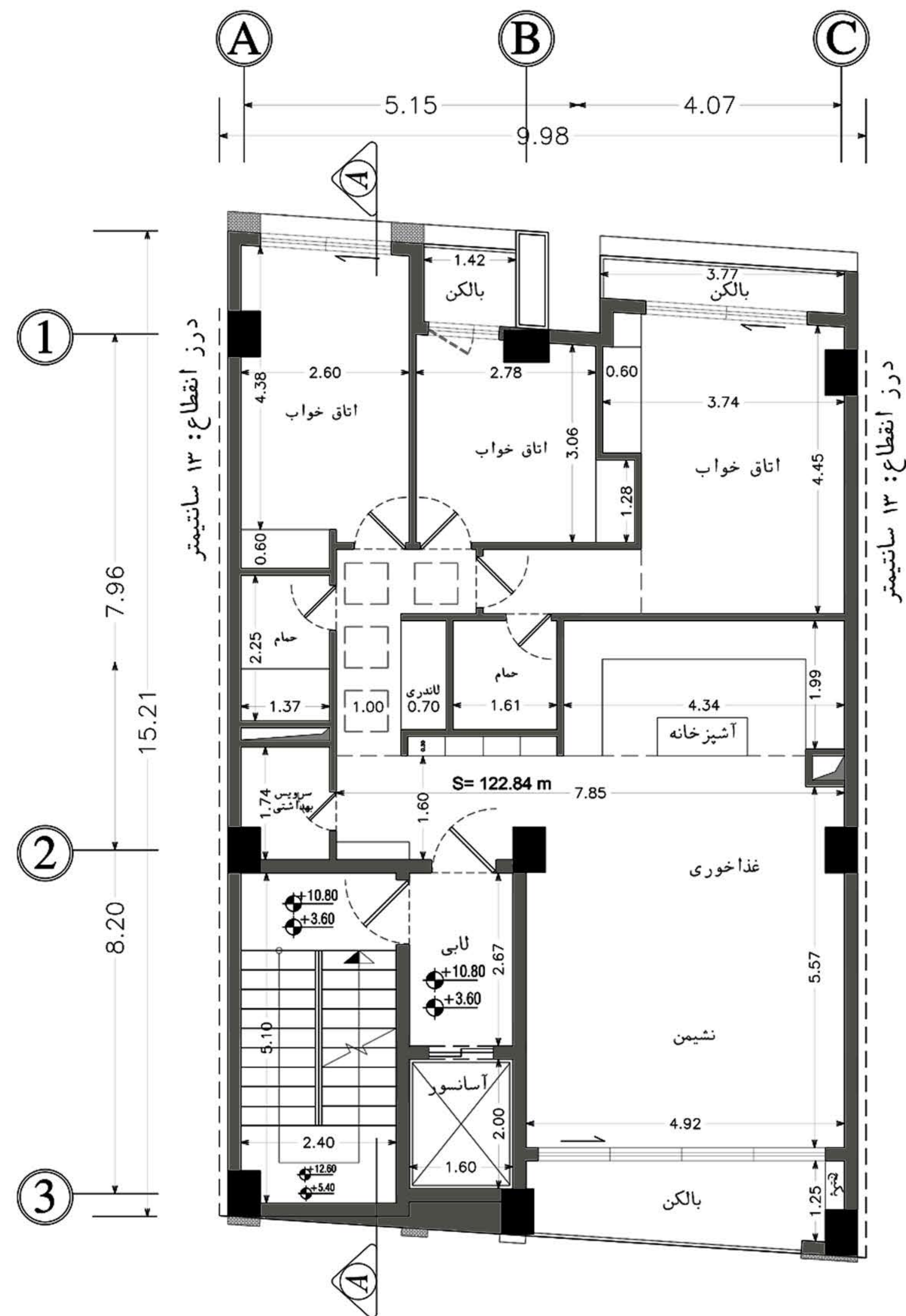
پلان اندازه گذاری طبقات اول و سوم
