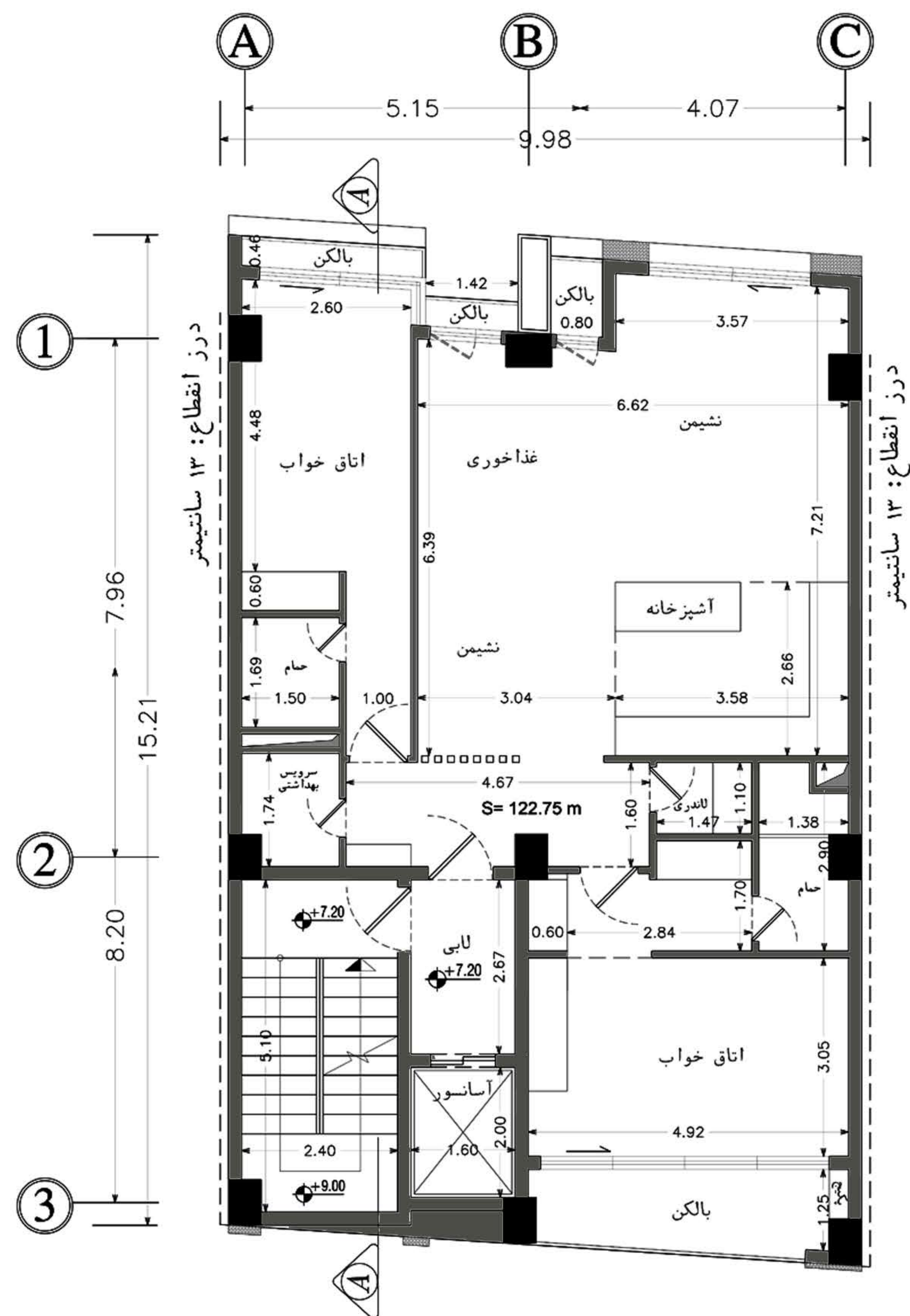
پلان اندازه گذاری طبقه دوم
