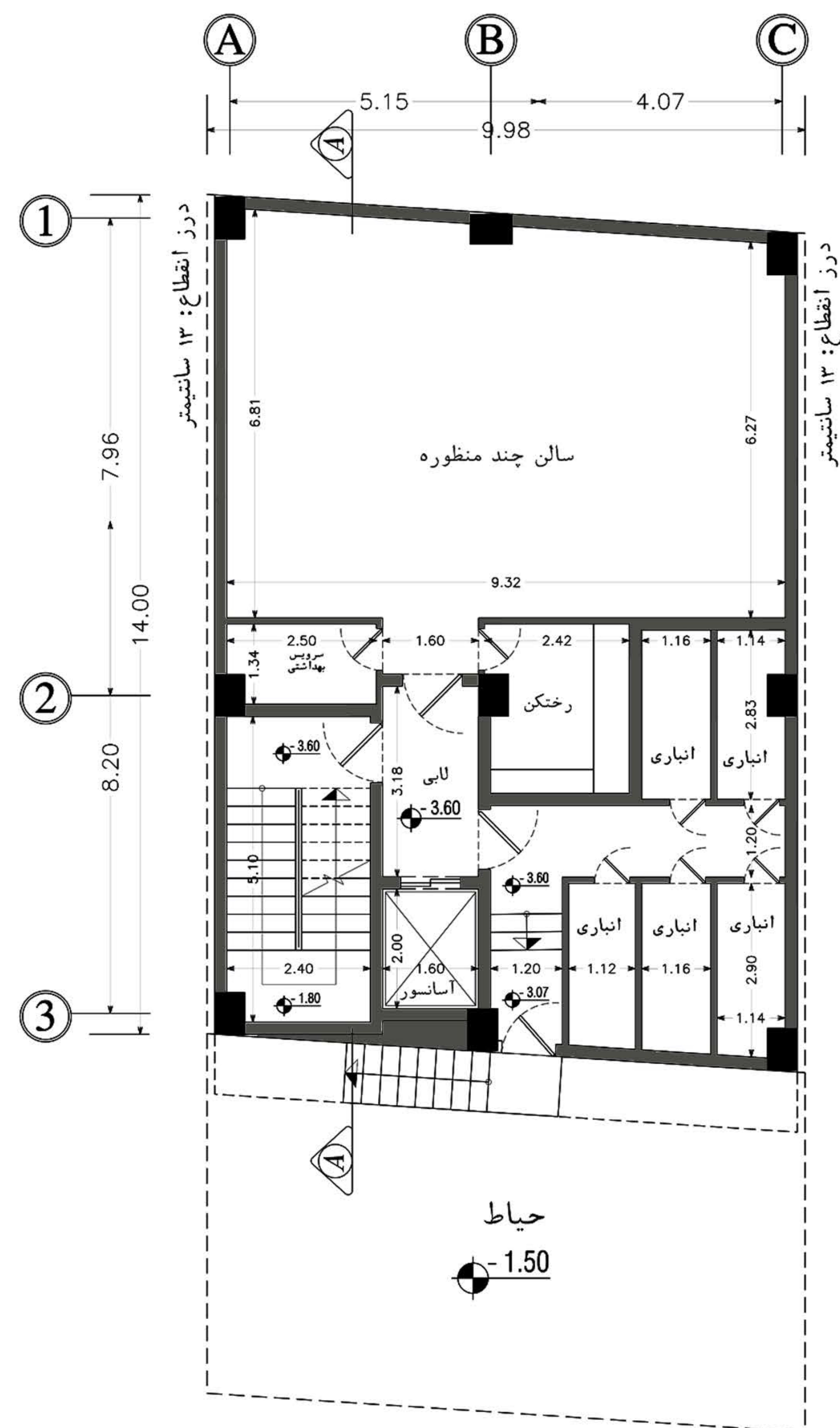
پلان اندازه گذاری زیرزمین
