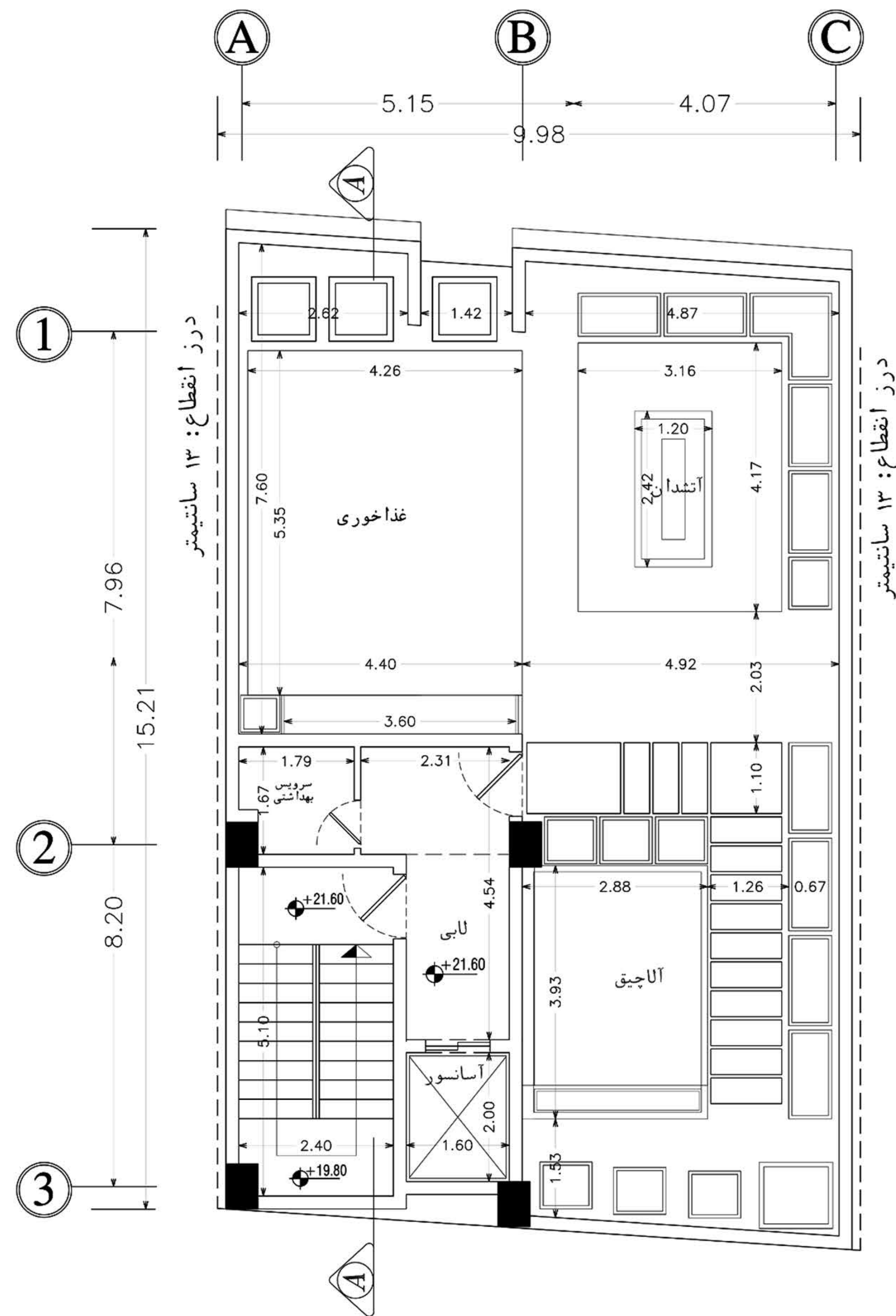
پلان اندازه گذاری روف گاردن
