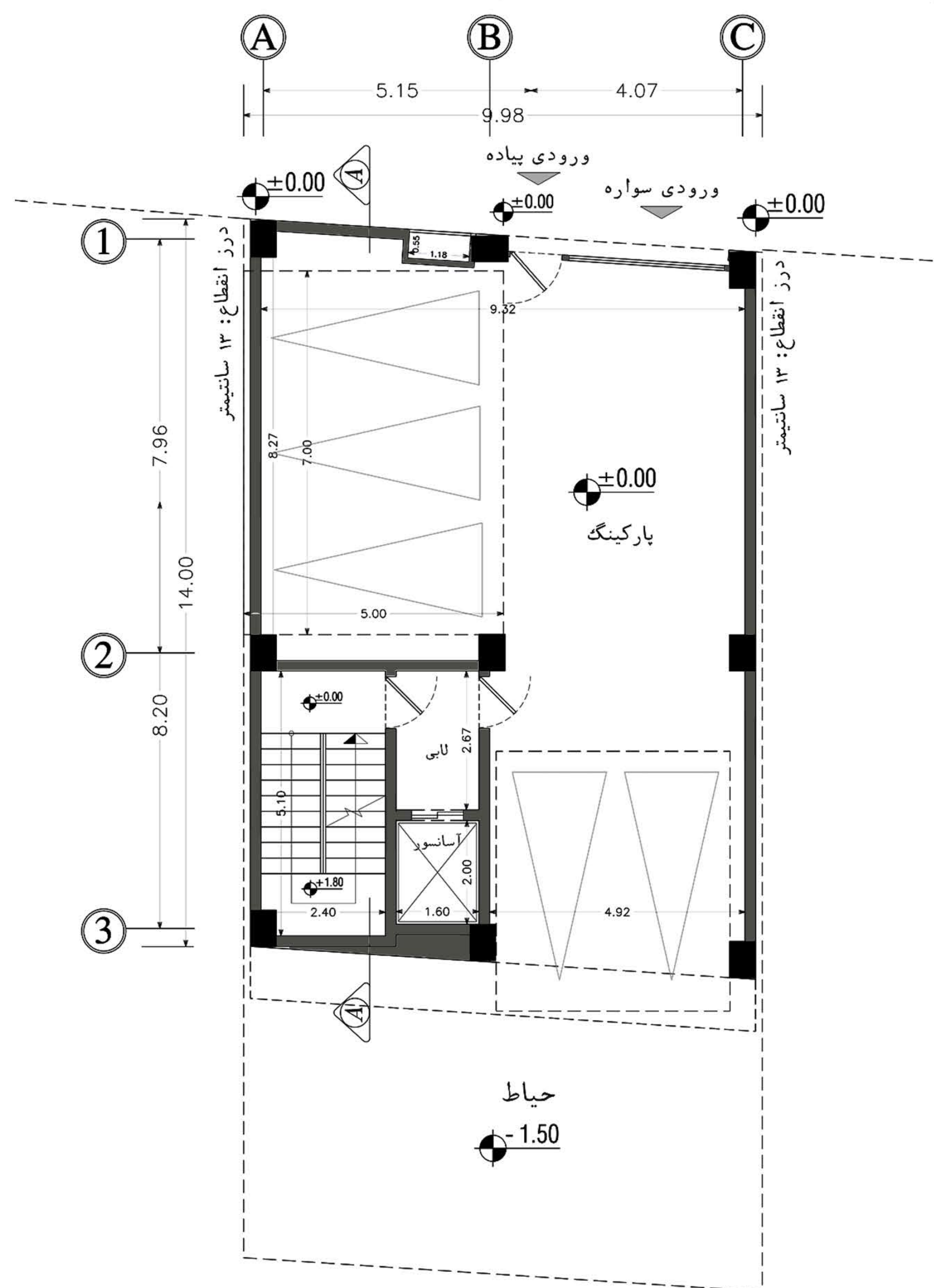
پلان اندازه گذاری طبقه همکف
