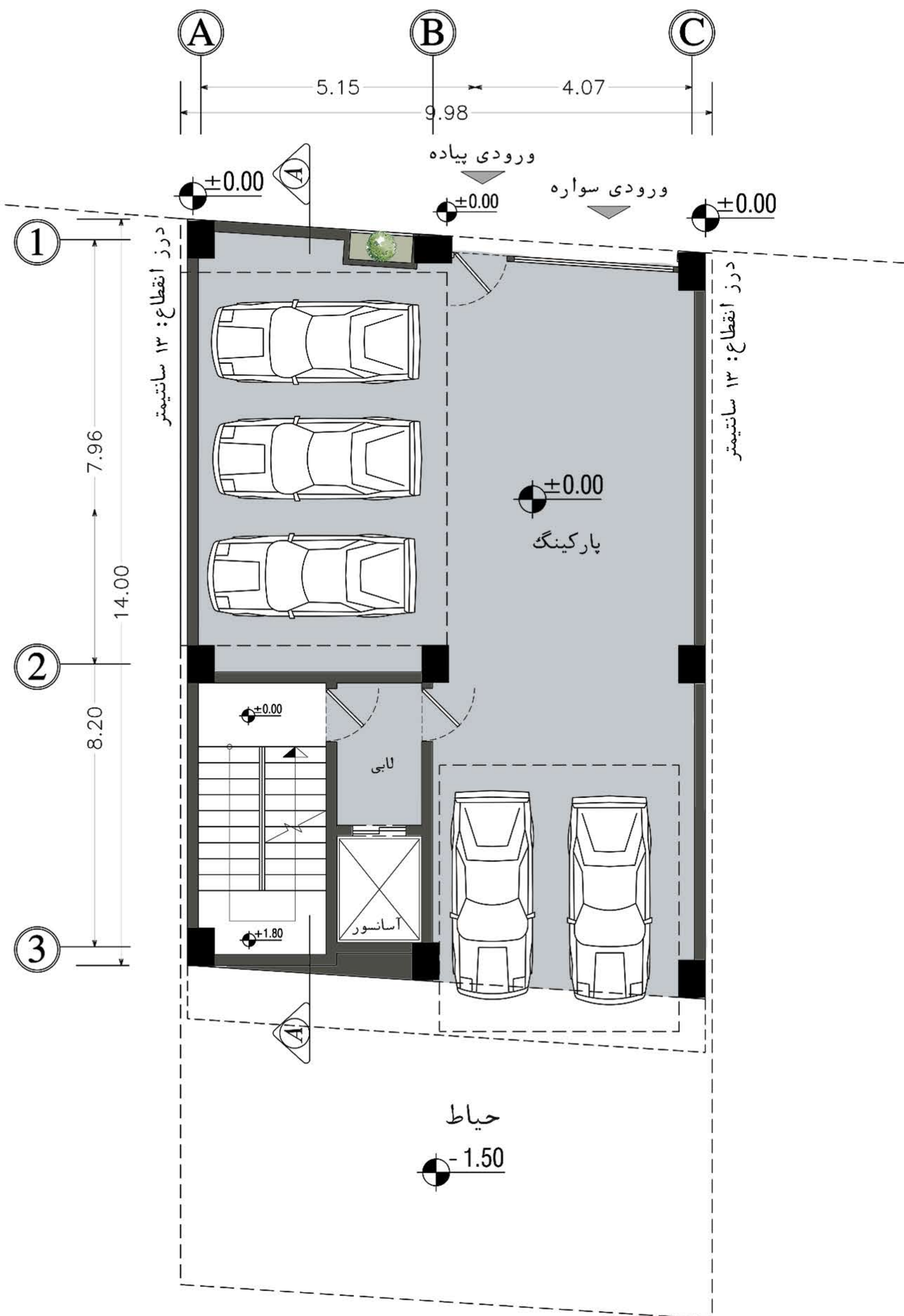
پلان مبلمان طبقه همکف
