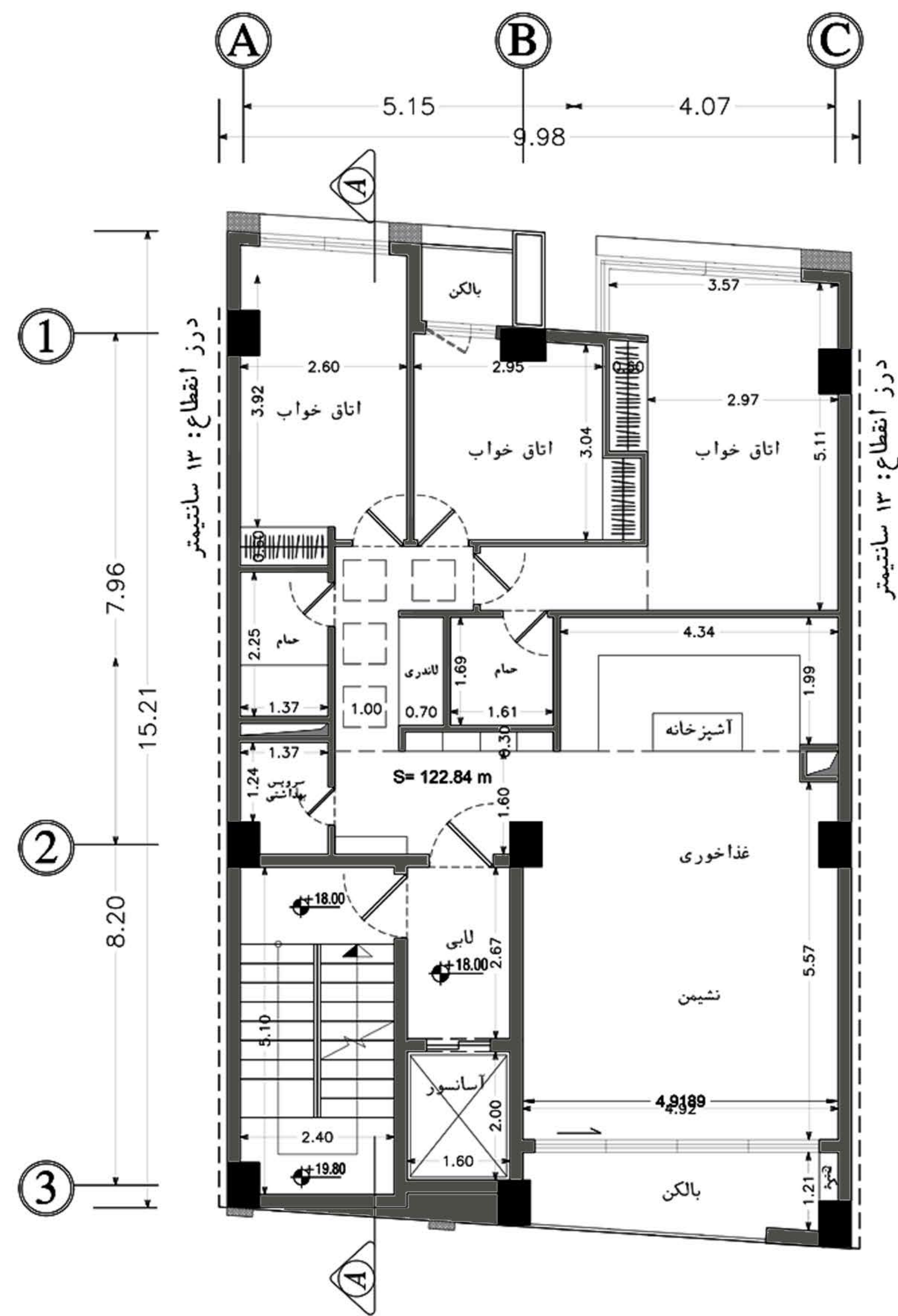
پلان اندازه گذاری طبقه پنجم
