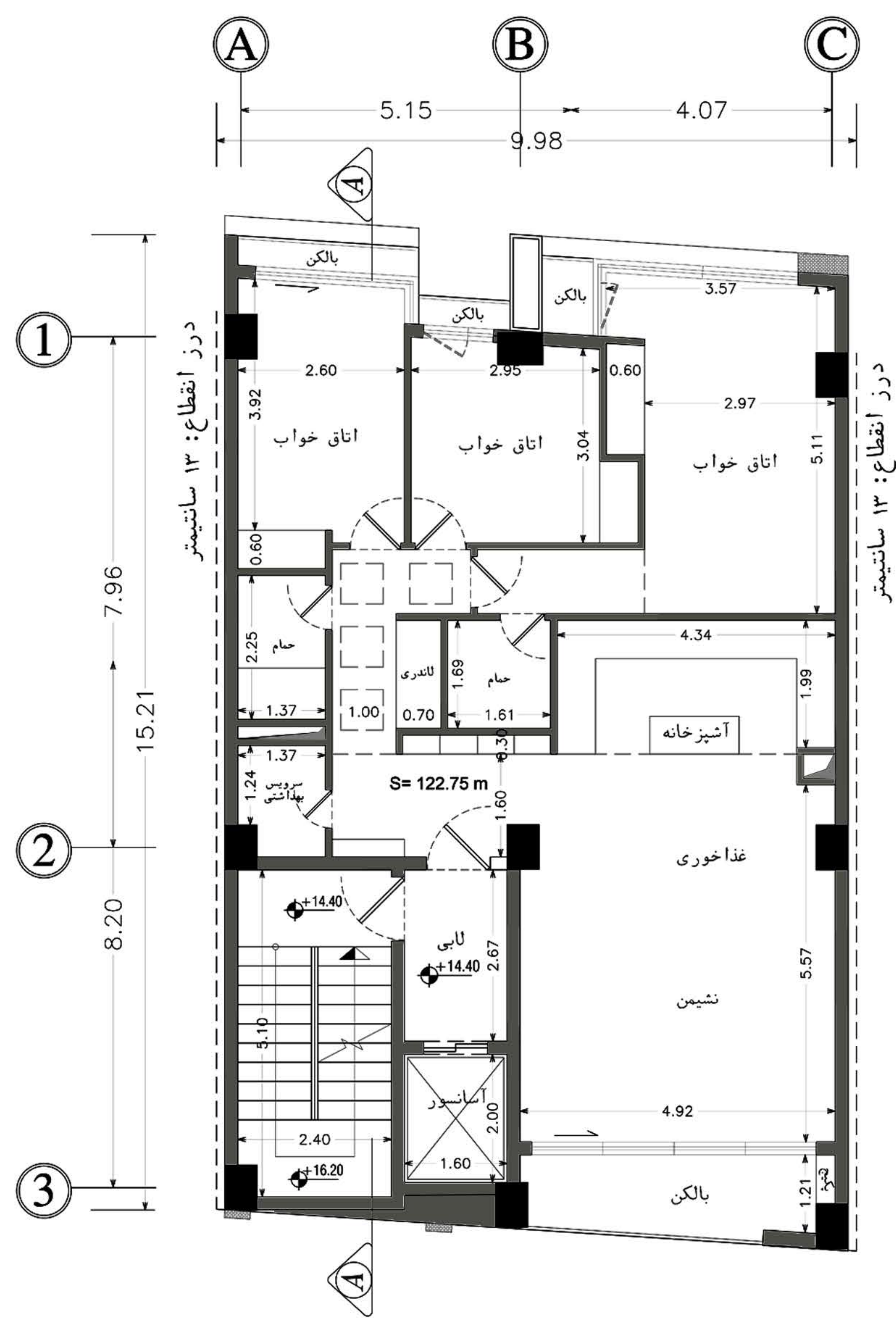
پلان اندازه گذاری طبقه چهارم
