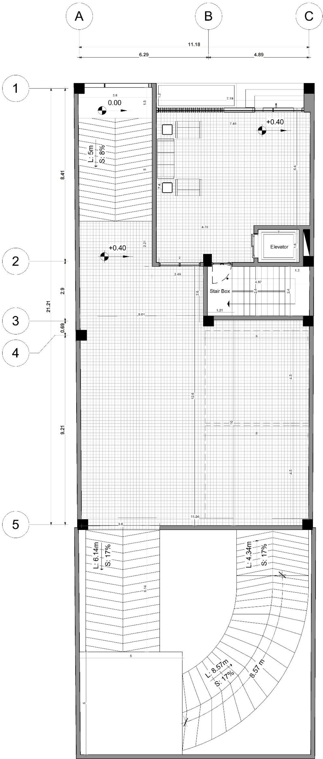
پلان اندازه گذاری طبقه همکف
