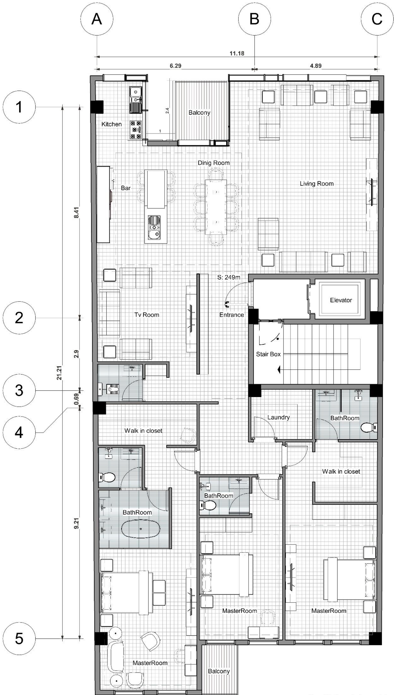
پلان مبلمان طبقات فرد
