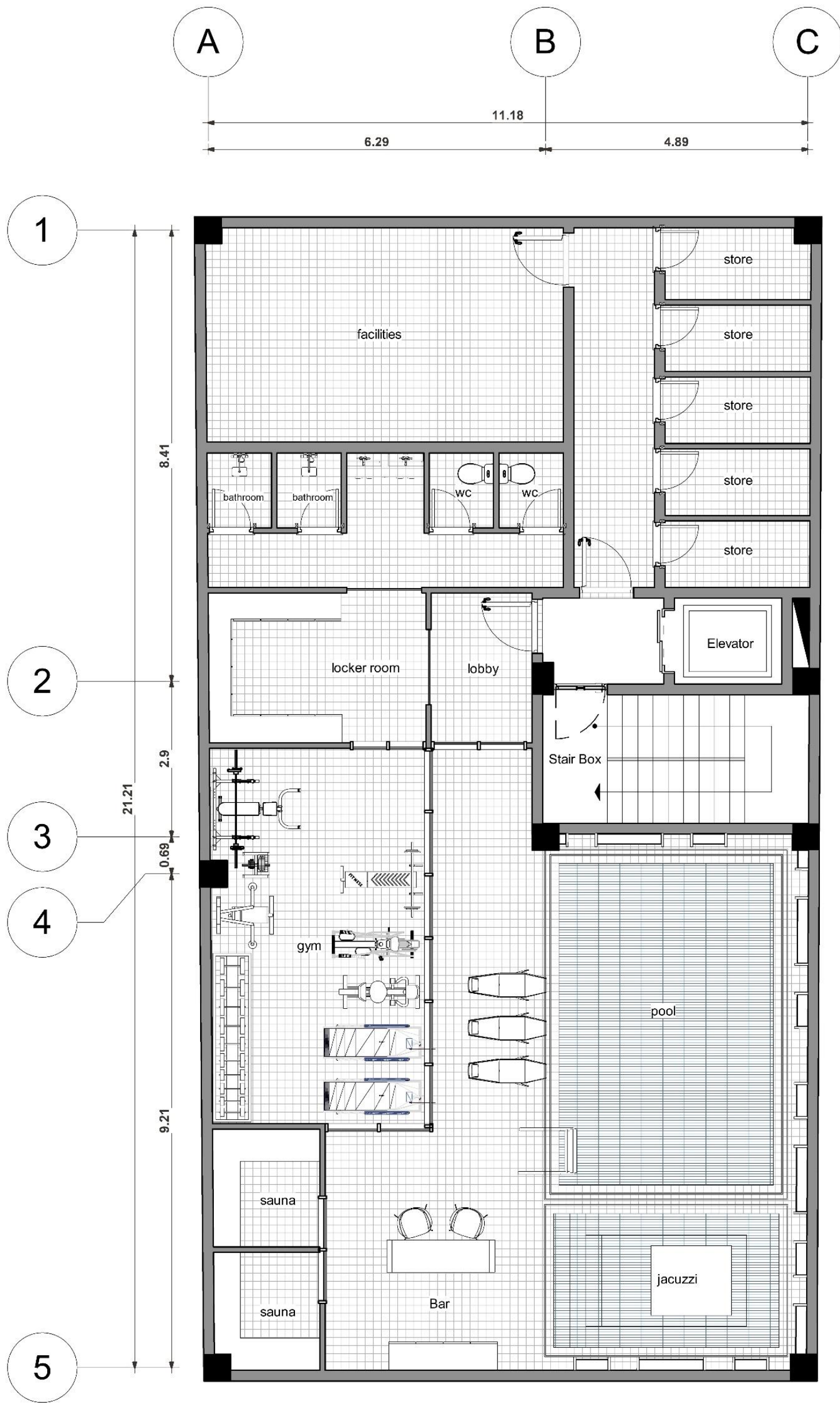
پلان مبلمان طبقه منفی دو
