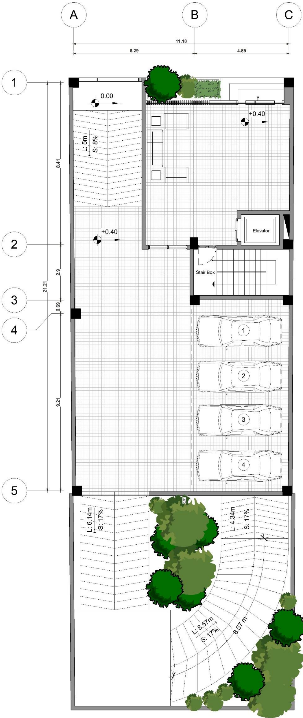
پلان مبلمان طبقه همکف
