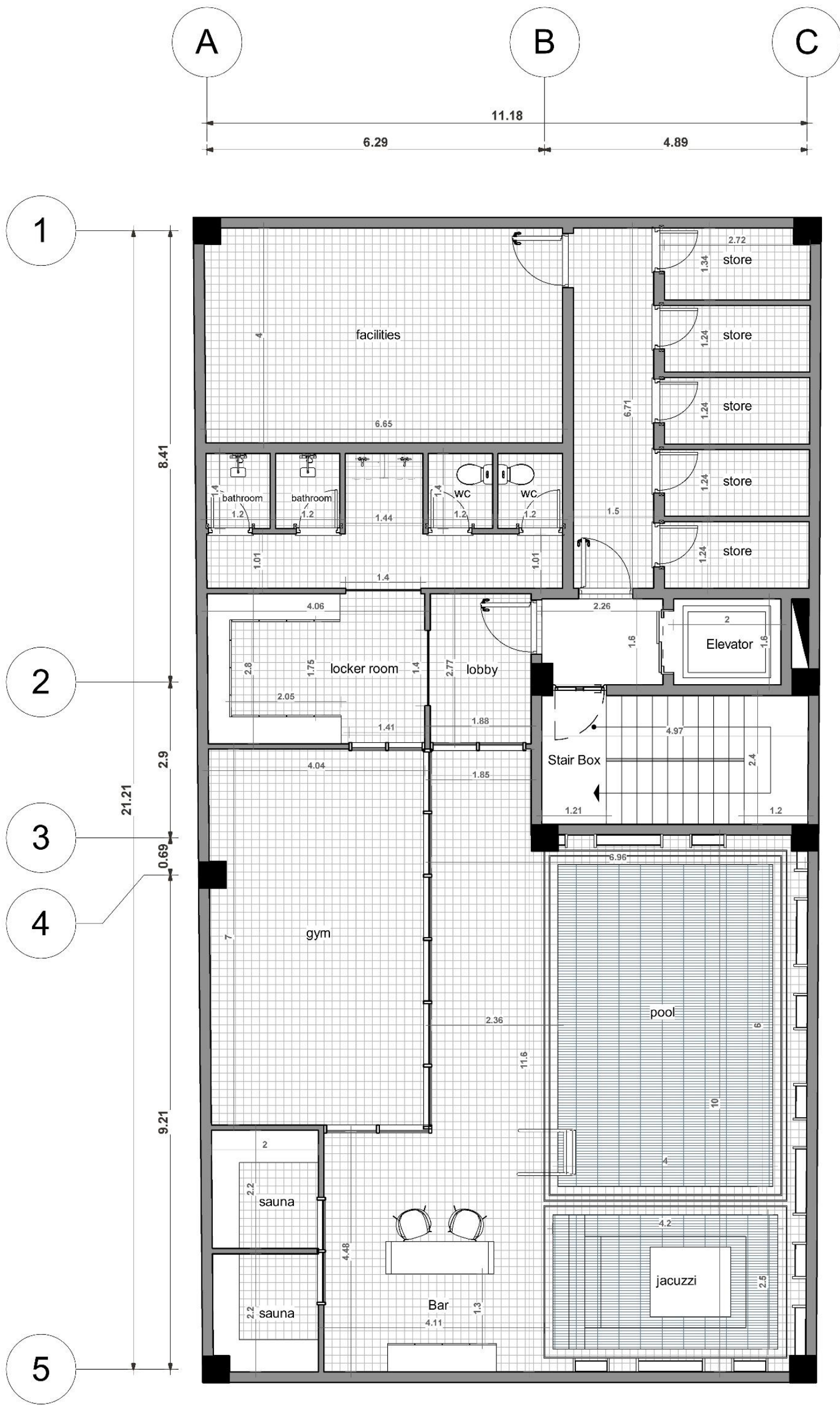
پلان اندازه گذاری طبقه منفی دو
