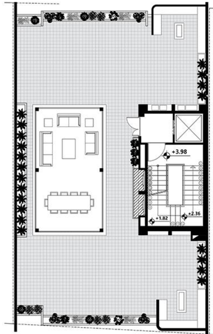
LEVEL : ROOF
