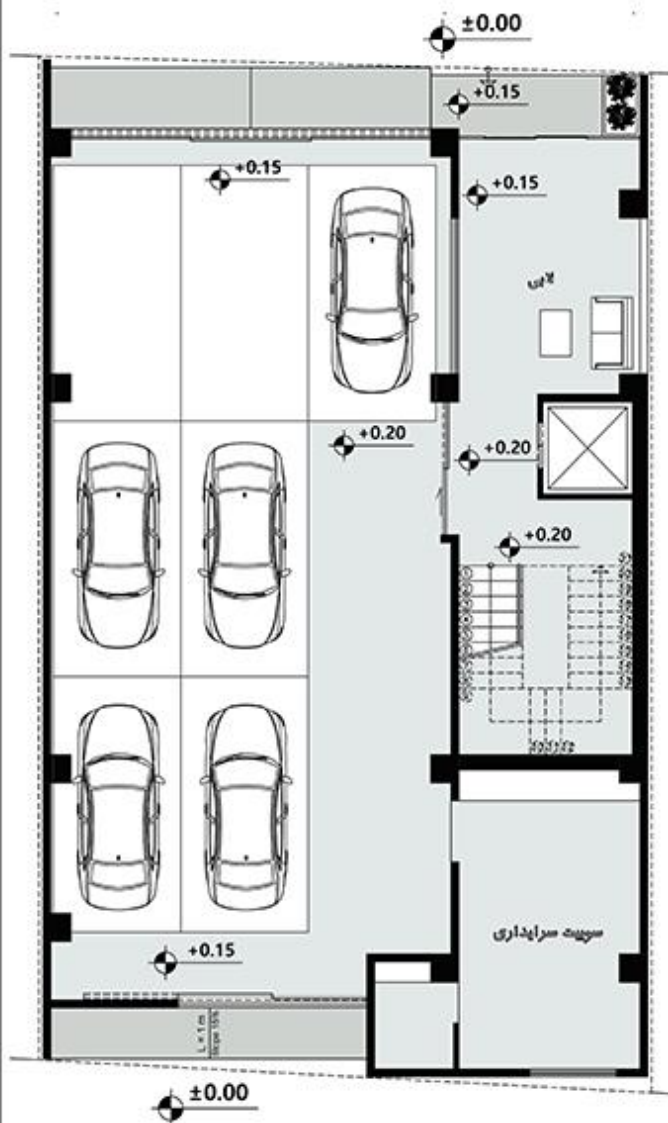
LEVEL : 0
