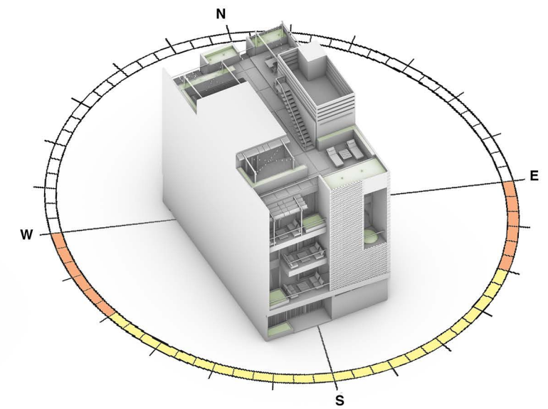
جهت گیری ساختمان نسبت تابش نور خورشید
