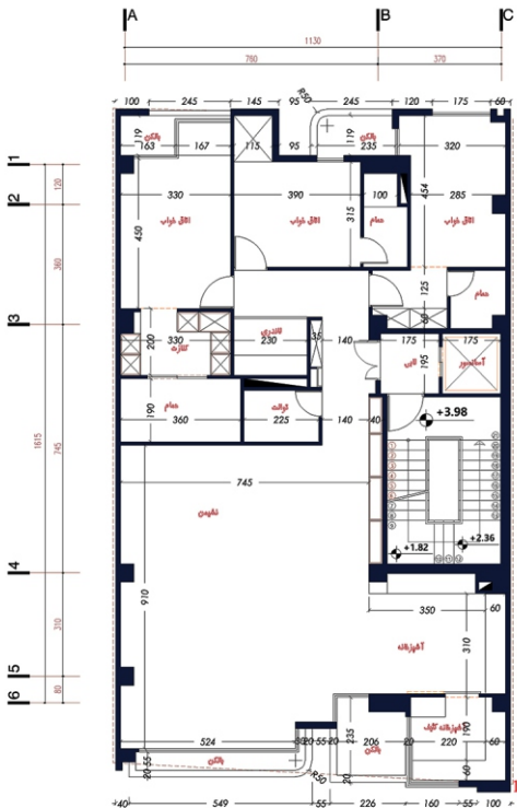
پلان طبقه اول
