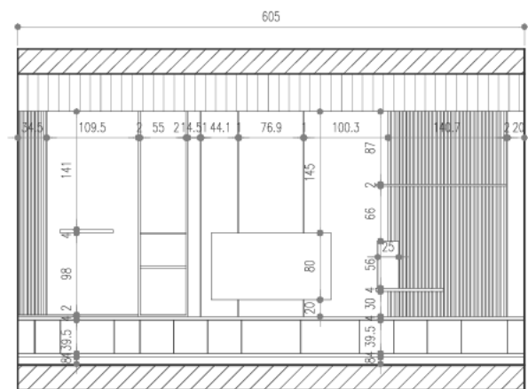
دیوار شمالی
