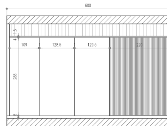
دیوار شرقی
