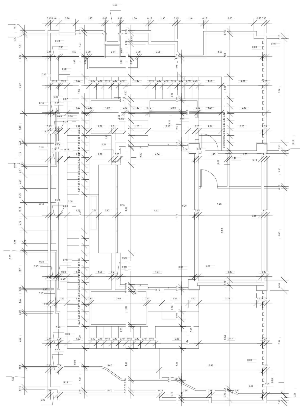
پلان اندازه گذاری بام
