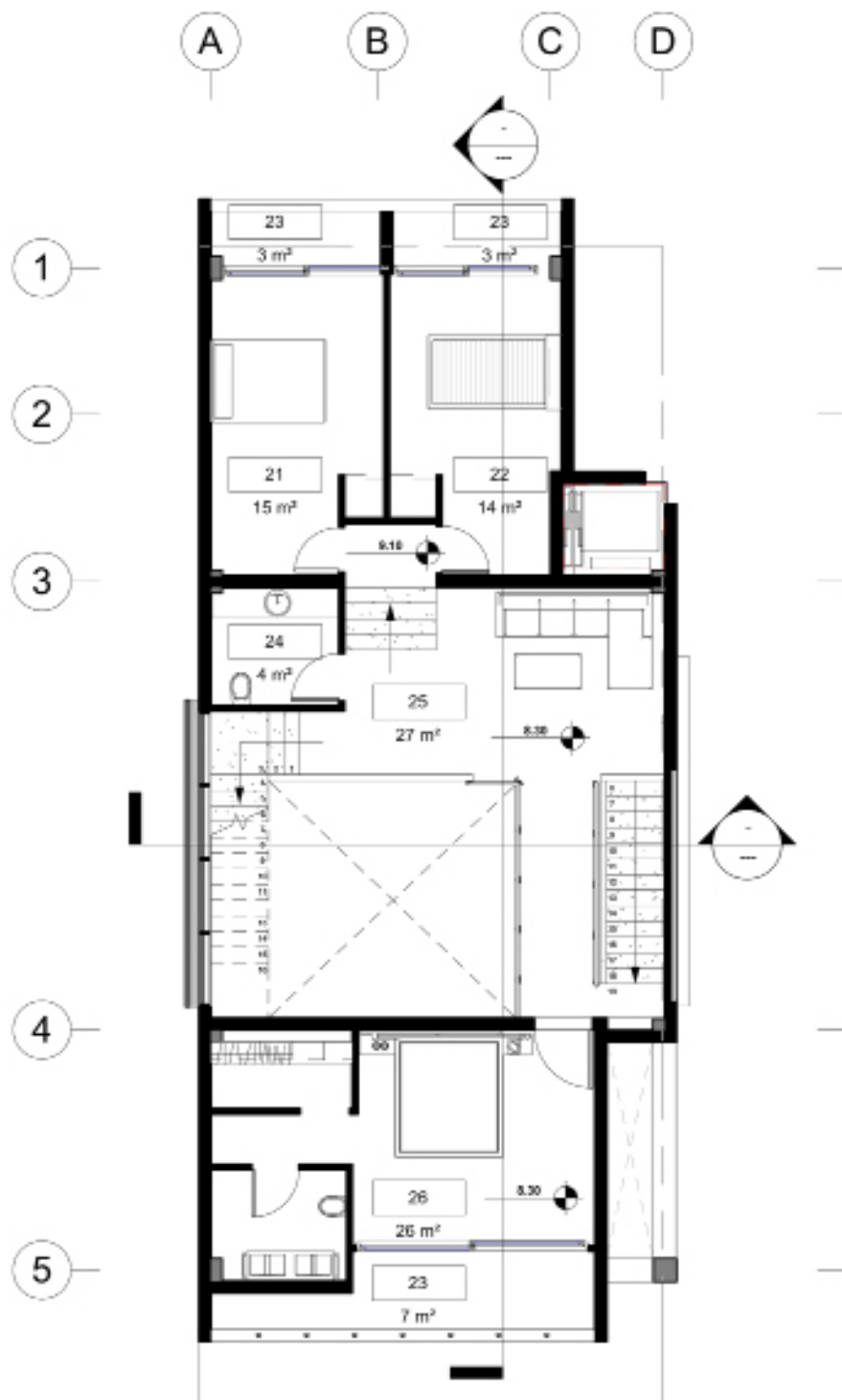
پلان مبلمان طبقه ی دوم
