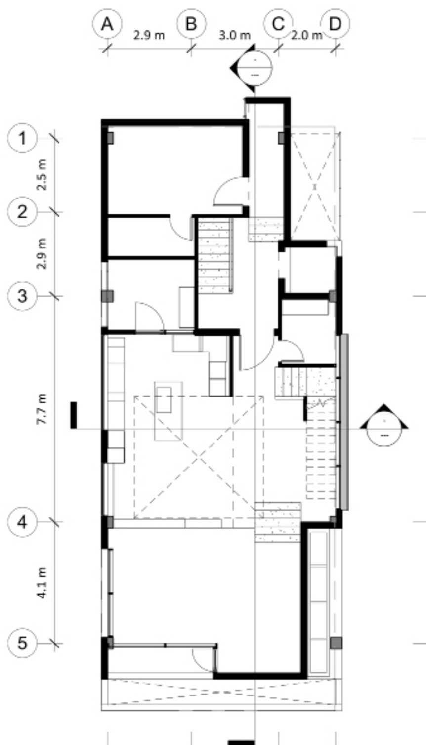
پلان اندازه گذاری طبقه ی اول
