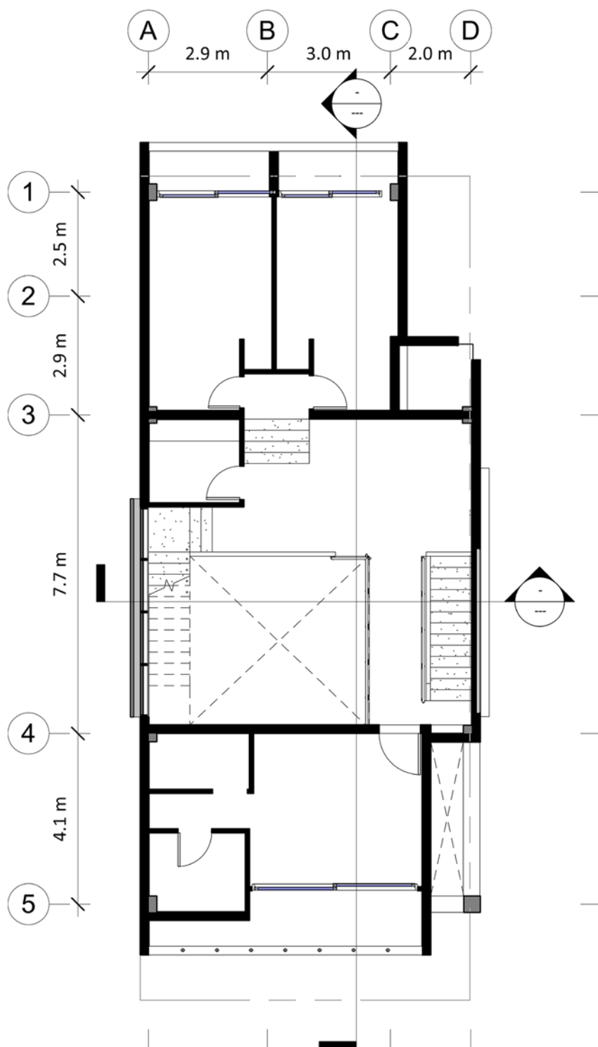
پلان اندازه گذاری طبقه ی دوم
