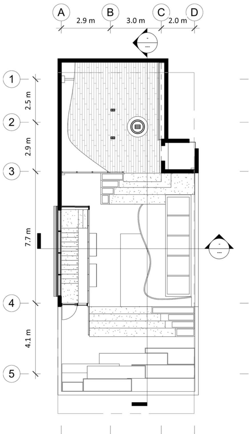
پلان اندازه گذاری روف گاردن
