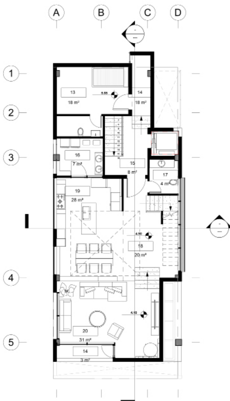
پلان مبلمان طبقه ی اول
