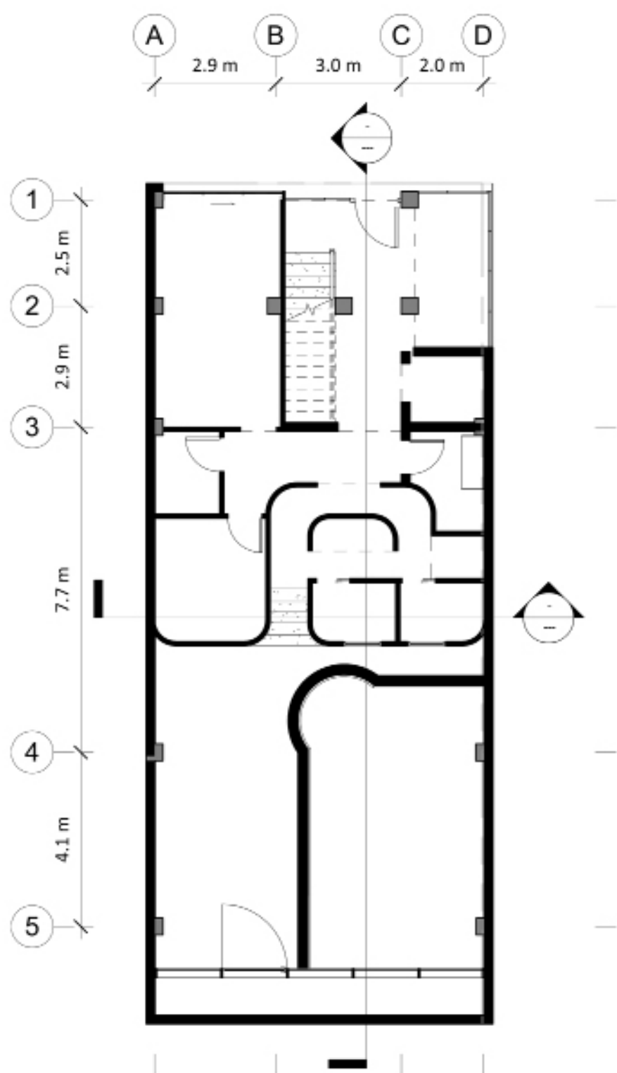
پلان اندازه گذاری طبقه ی همکف
