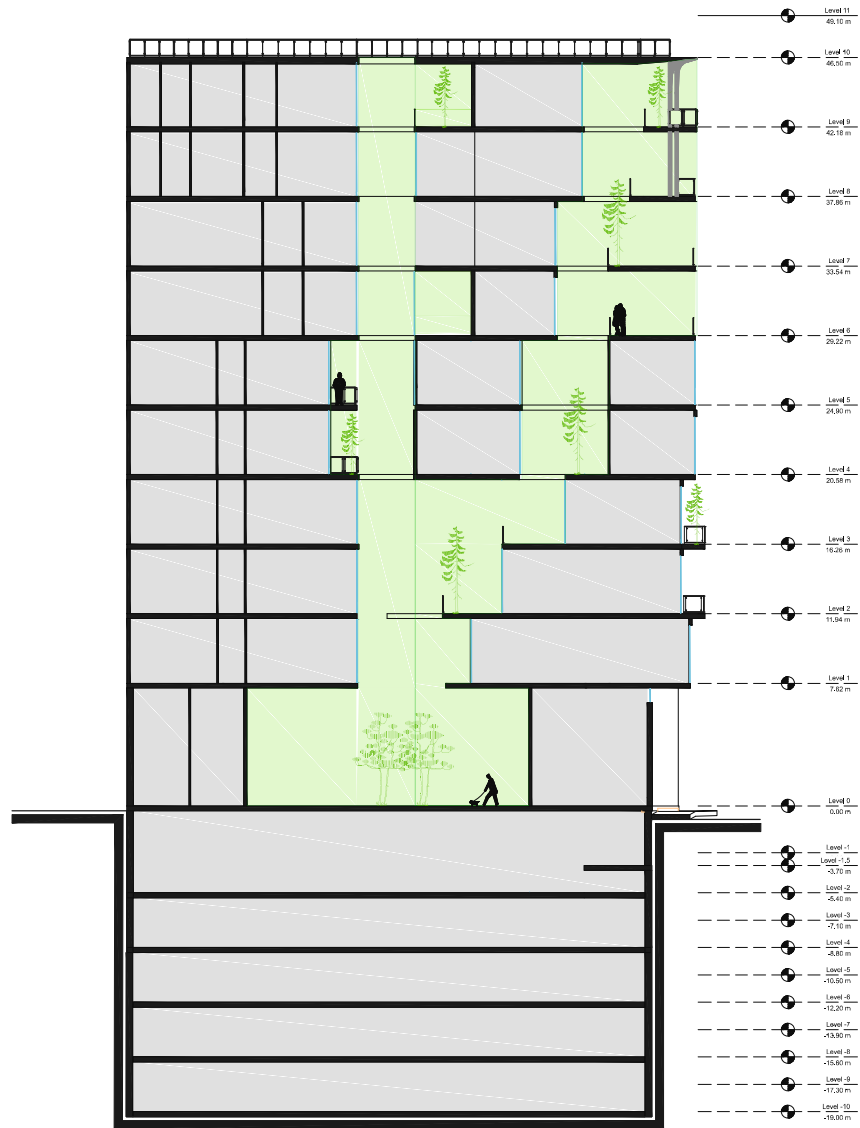
SECTION A-A & B-B
