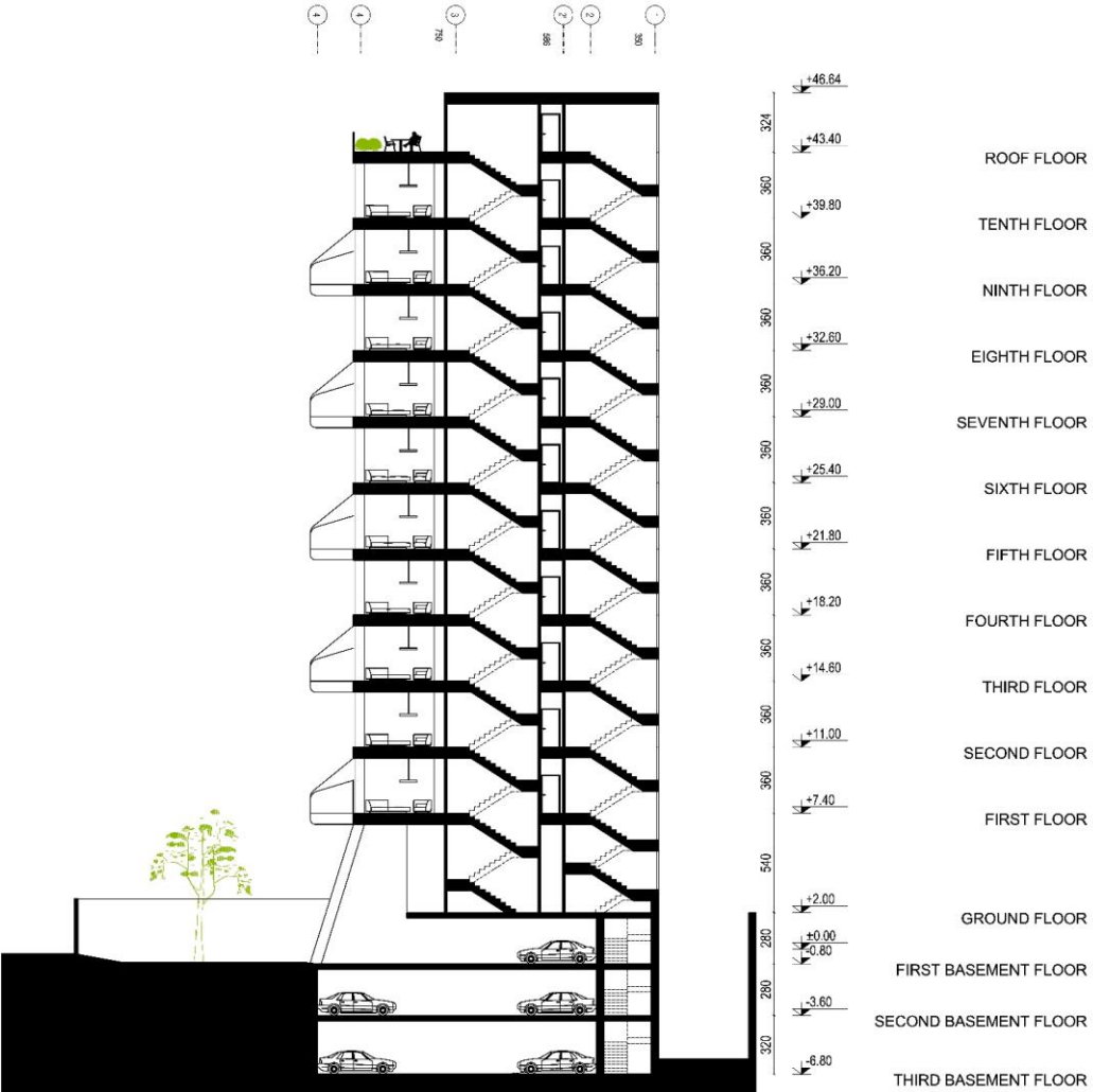
SECTION A-A 1 2 5 10
