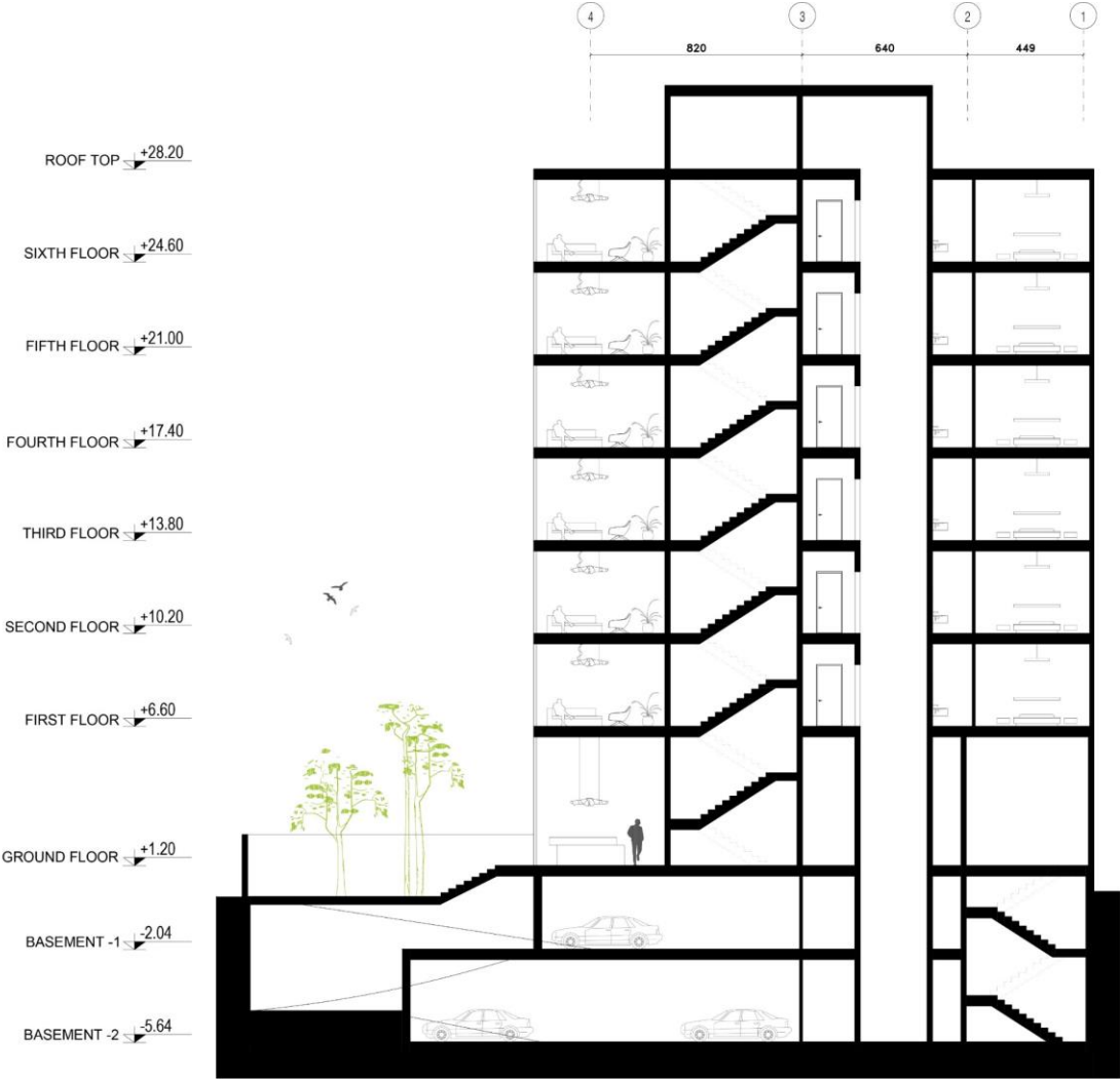
SECTION A-A
