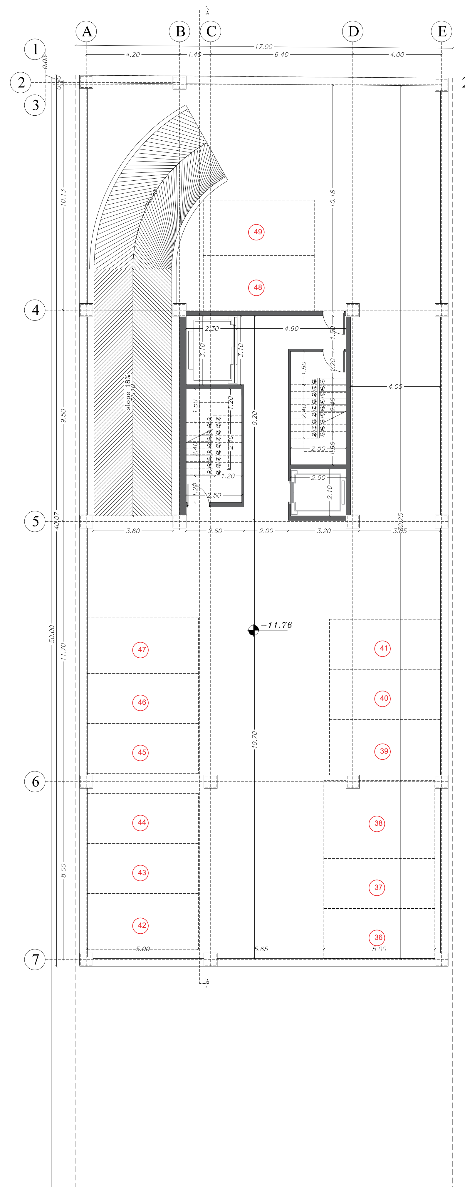
پلان اندازه گذاری ۴
