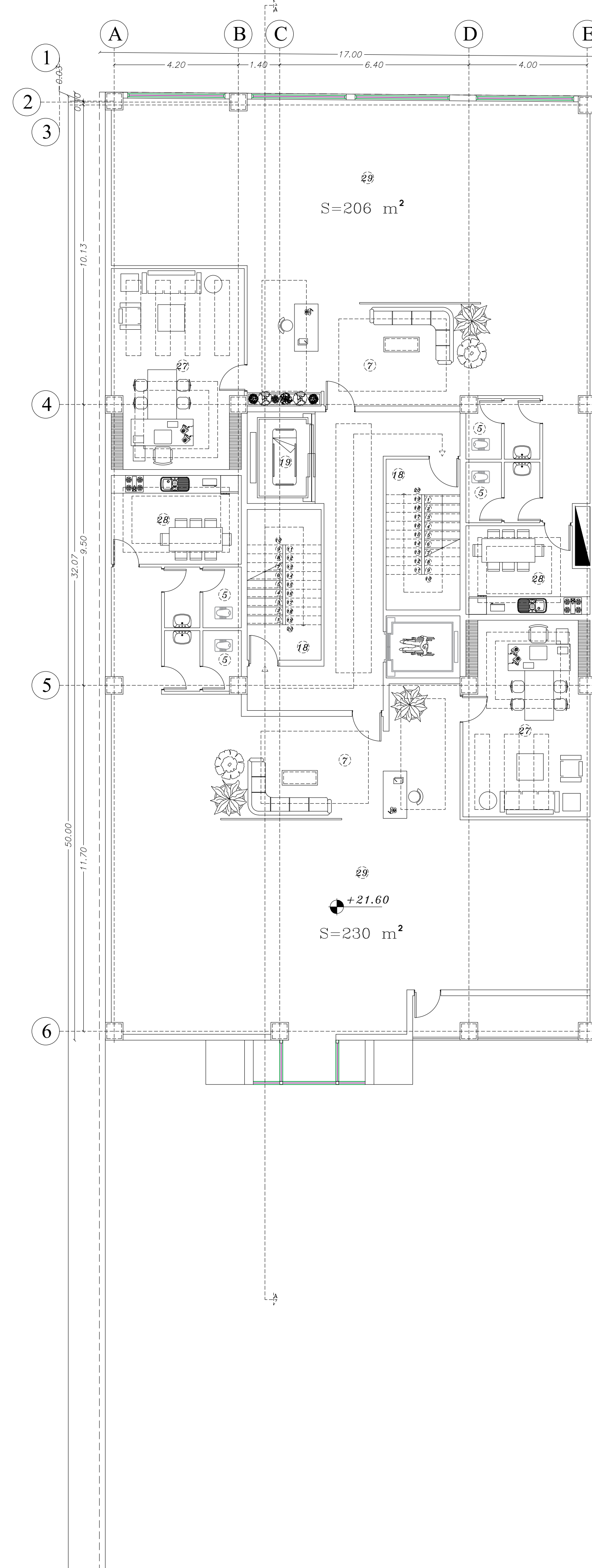
پلان مبلمان طبقه پنجم
