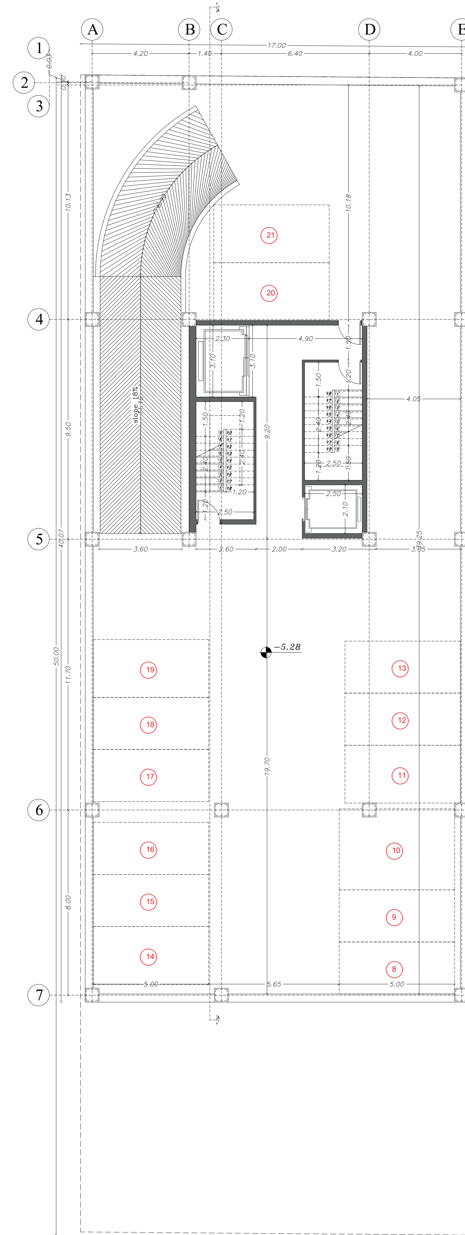
پلان اندازه گذاری ۲- Sc: 1:100
