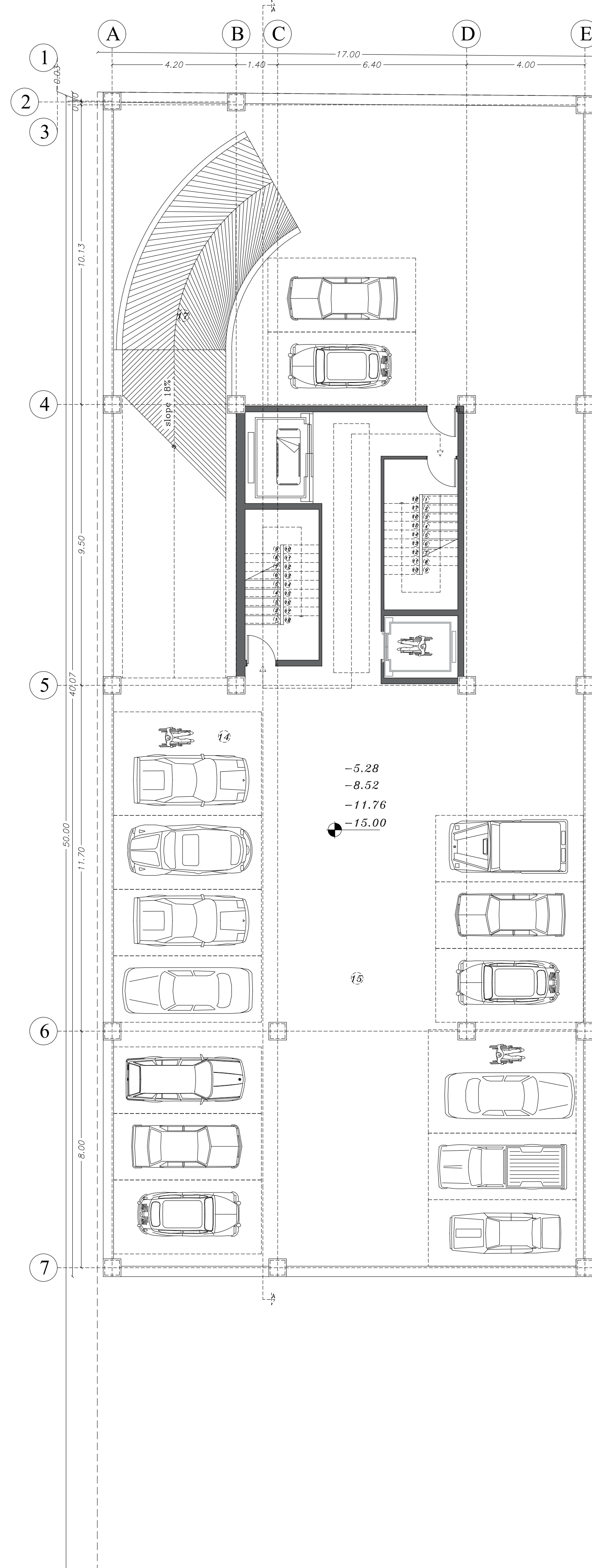
پلان مبلمان پارکینگ ۲- الی ۵-
