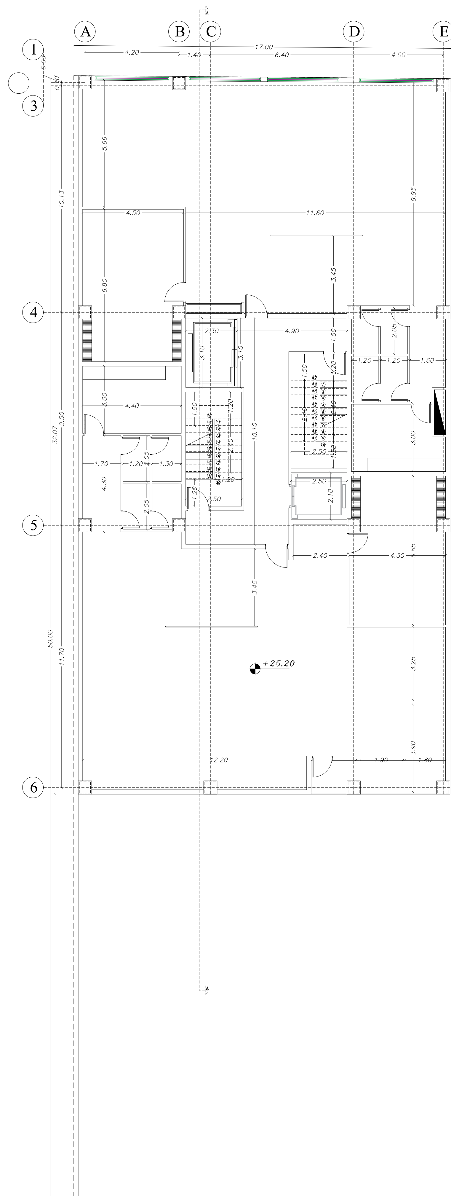
پلان اندازه گذاری طبقه ششم
