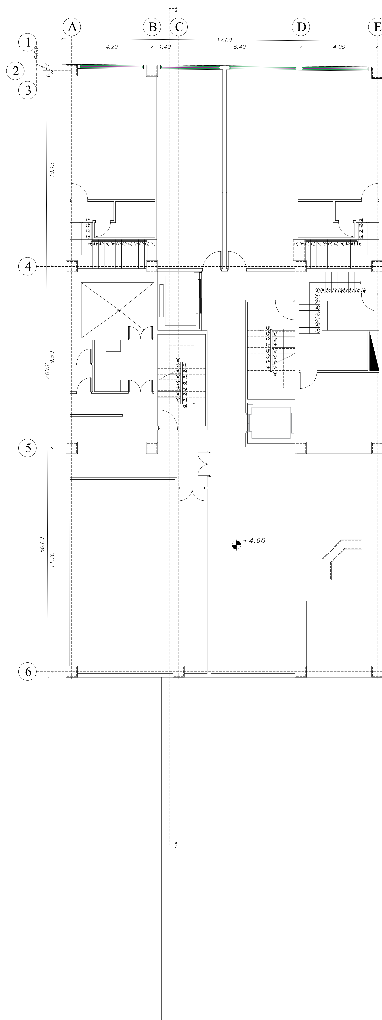
پلان اندازه گذاری دوبلکس
