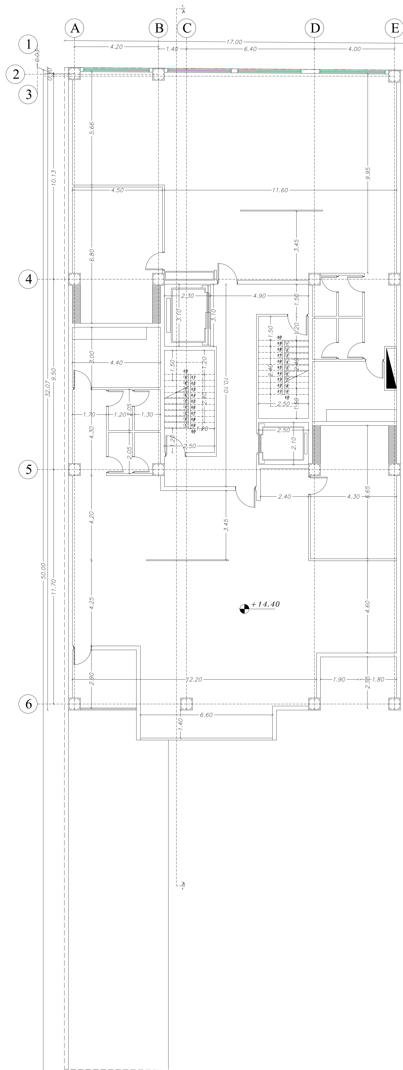
پلان اندازه گذاری طبقه سوم
