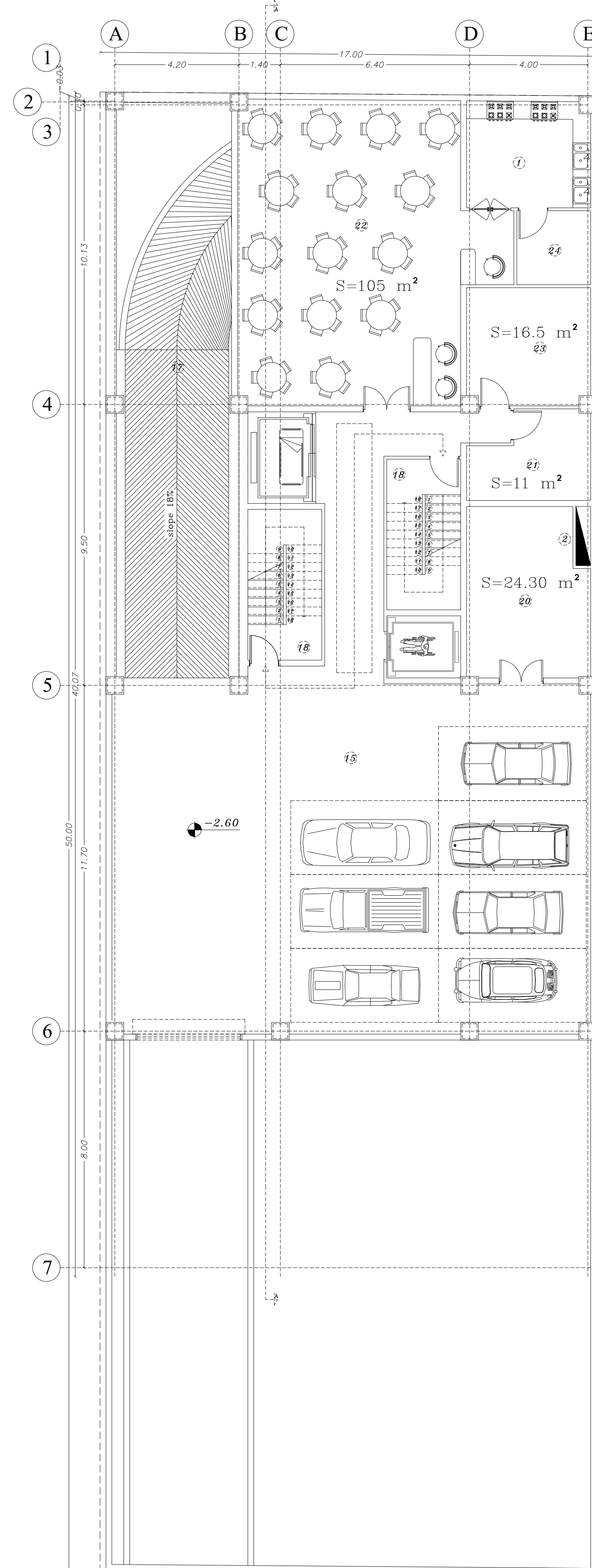
پلان مبلمان پارکینگ ۱-
