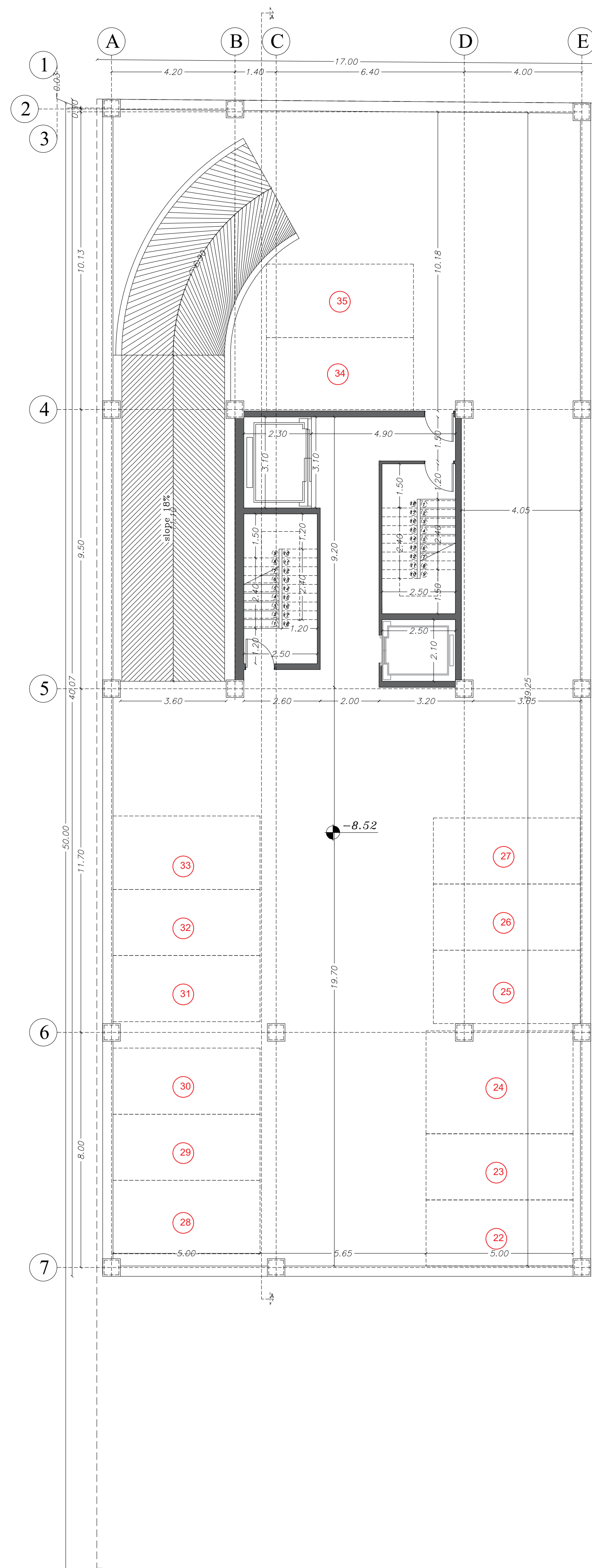
پلان اندازه گذاری ۳- Sc: 1:100
