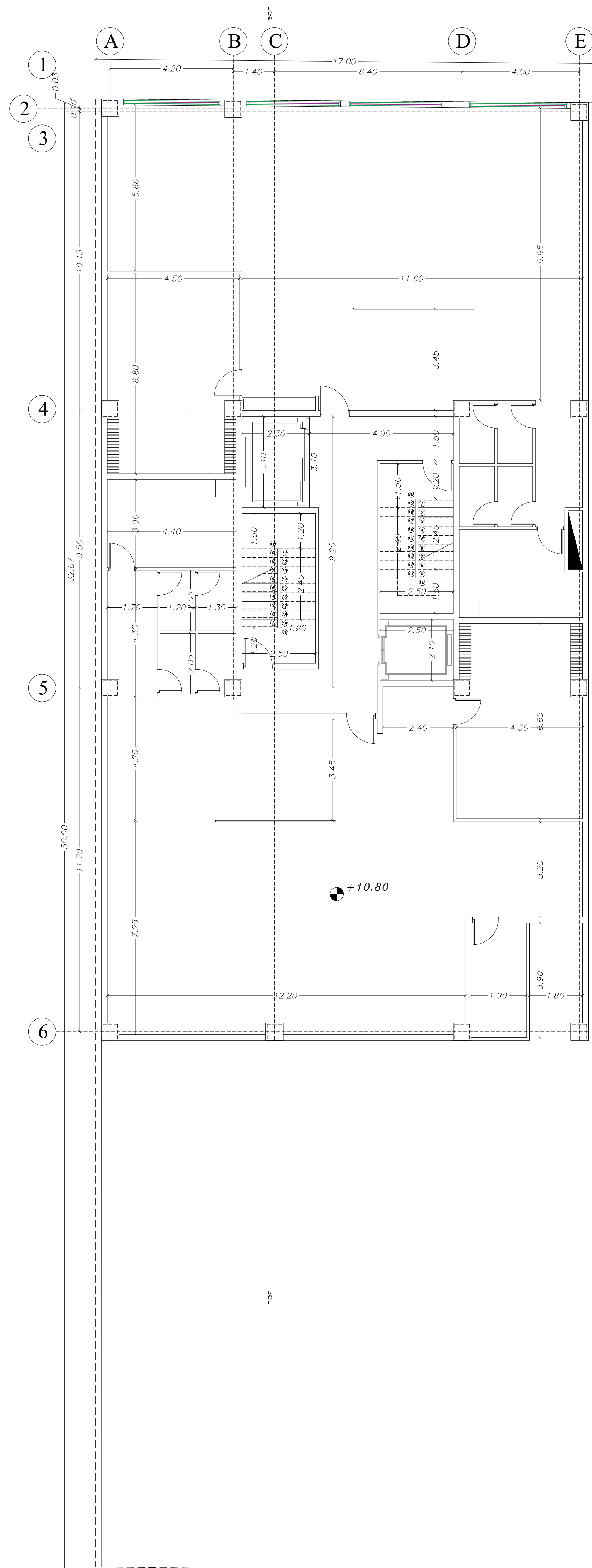
پلان اندازه گذاری طبقه دوم
