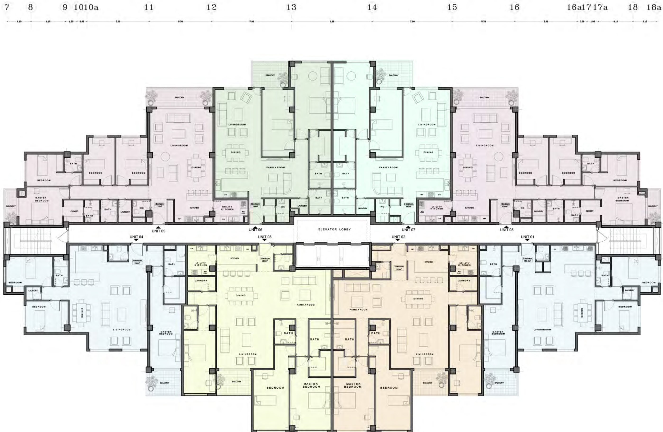
پلان مبلمان طبقه ی 8 واحدی
