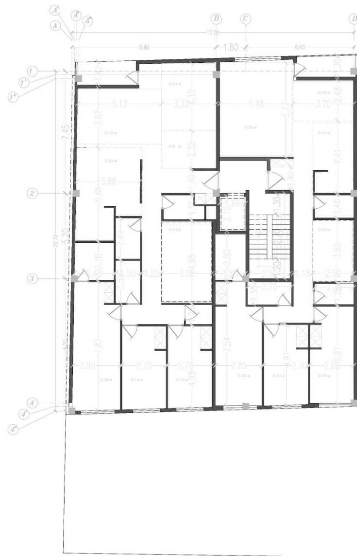
پلان طبقات
