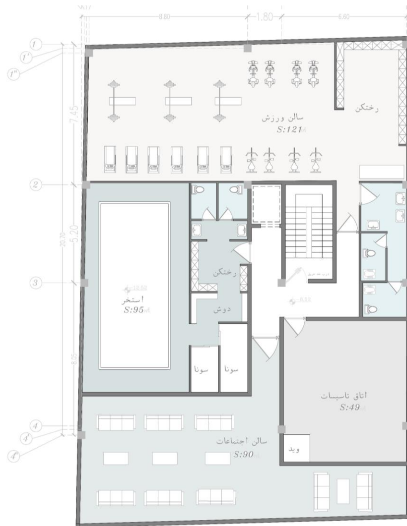
پلان زیرزمین 3-
