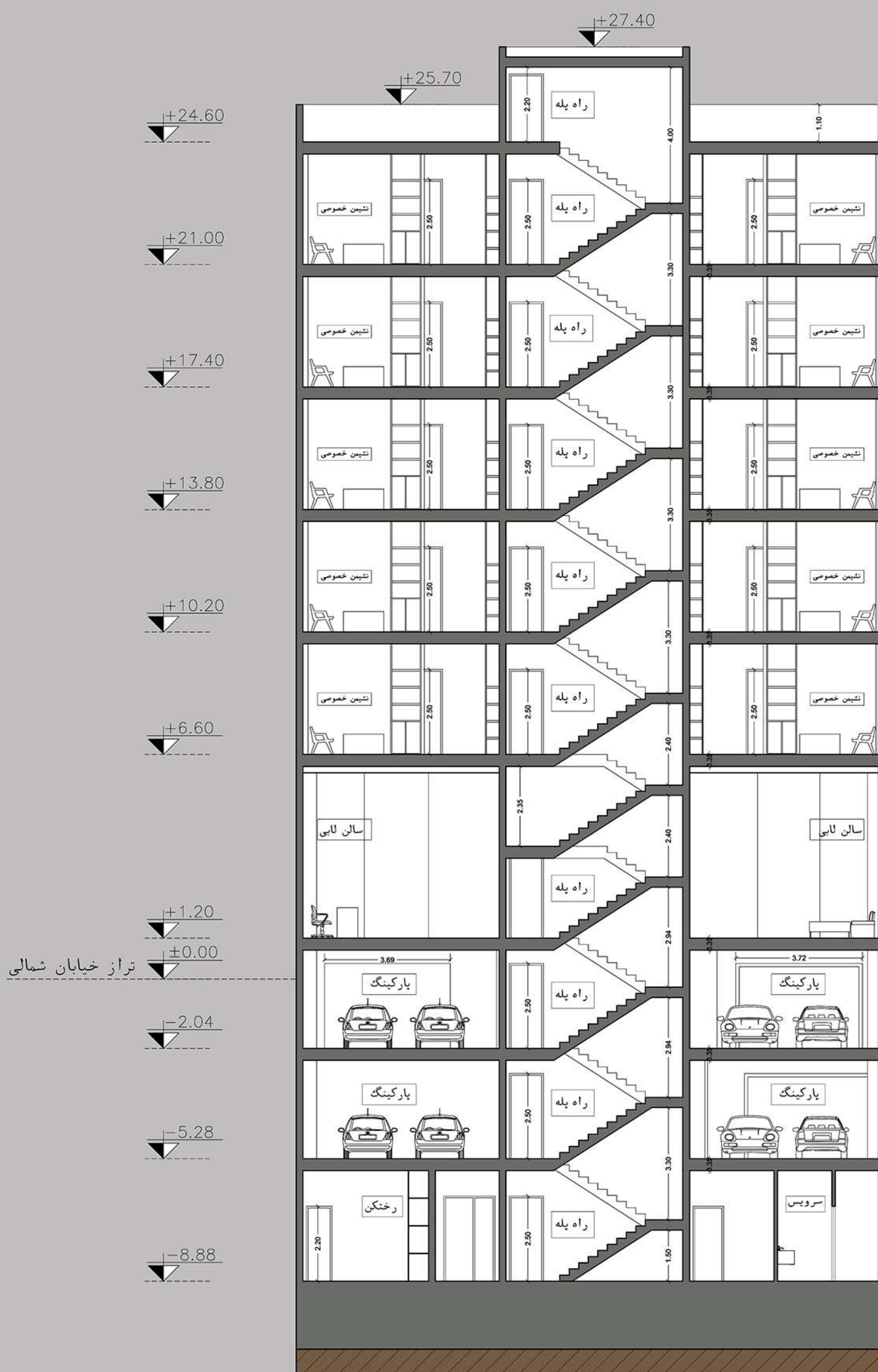
مقطع B_B
