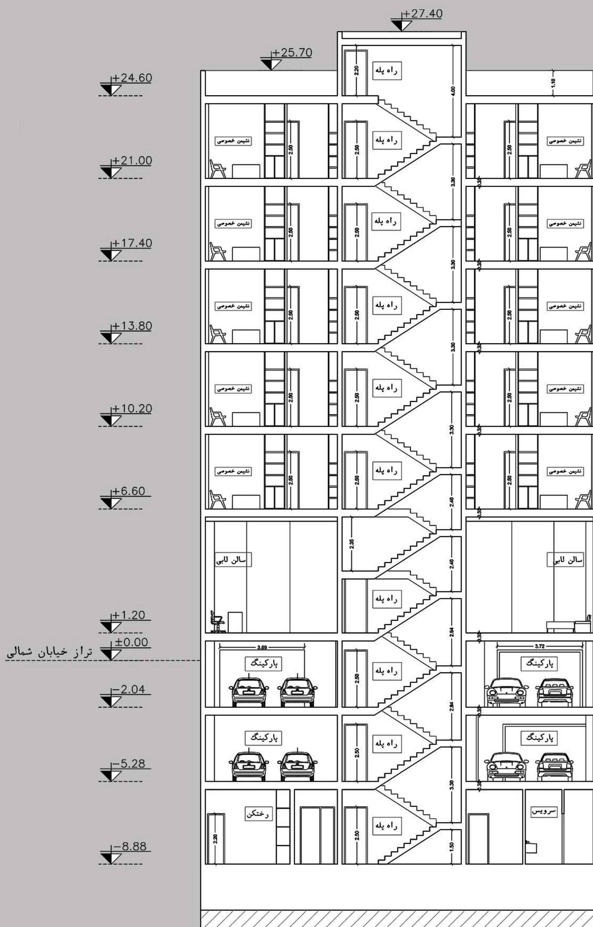
مقطع B_B
