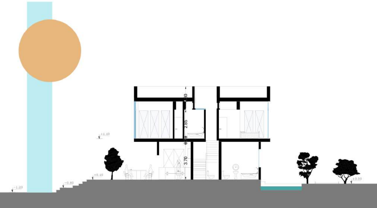
Section A-A
