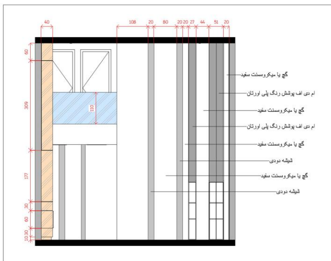
1 Wall 1 : 50
