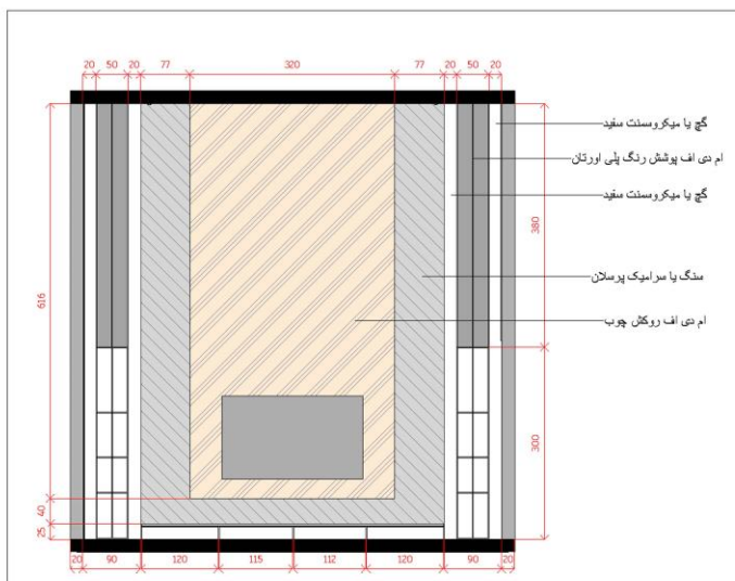
1 Tv wall 1 : 50
