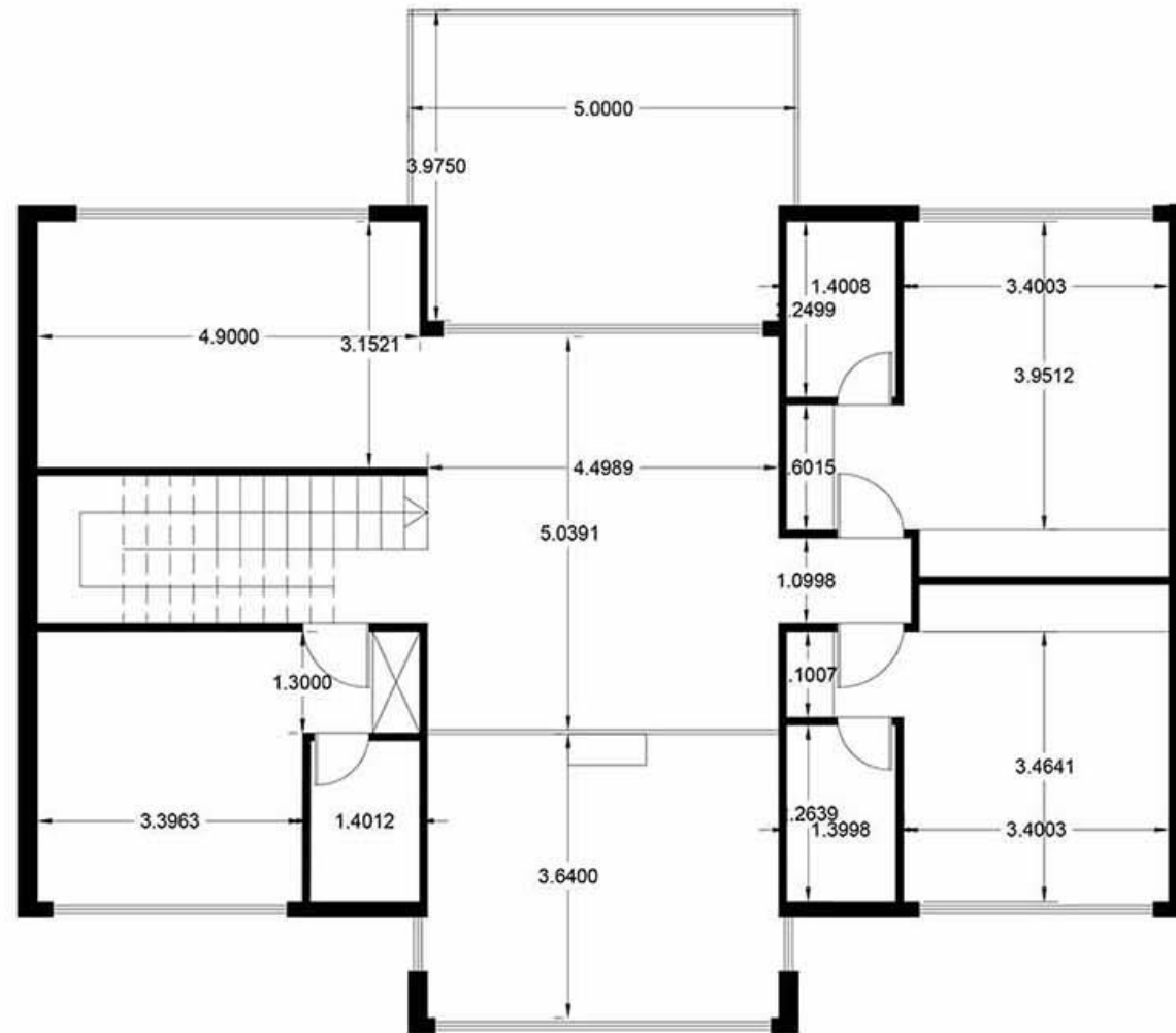
پلان اندازه گذاری طبقه اول
