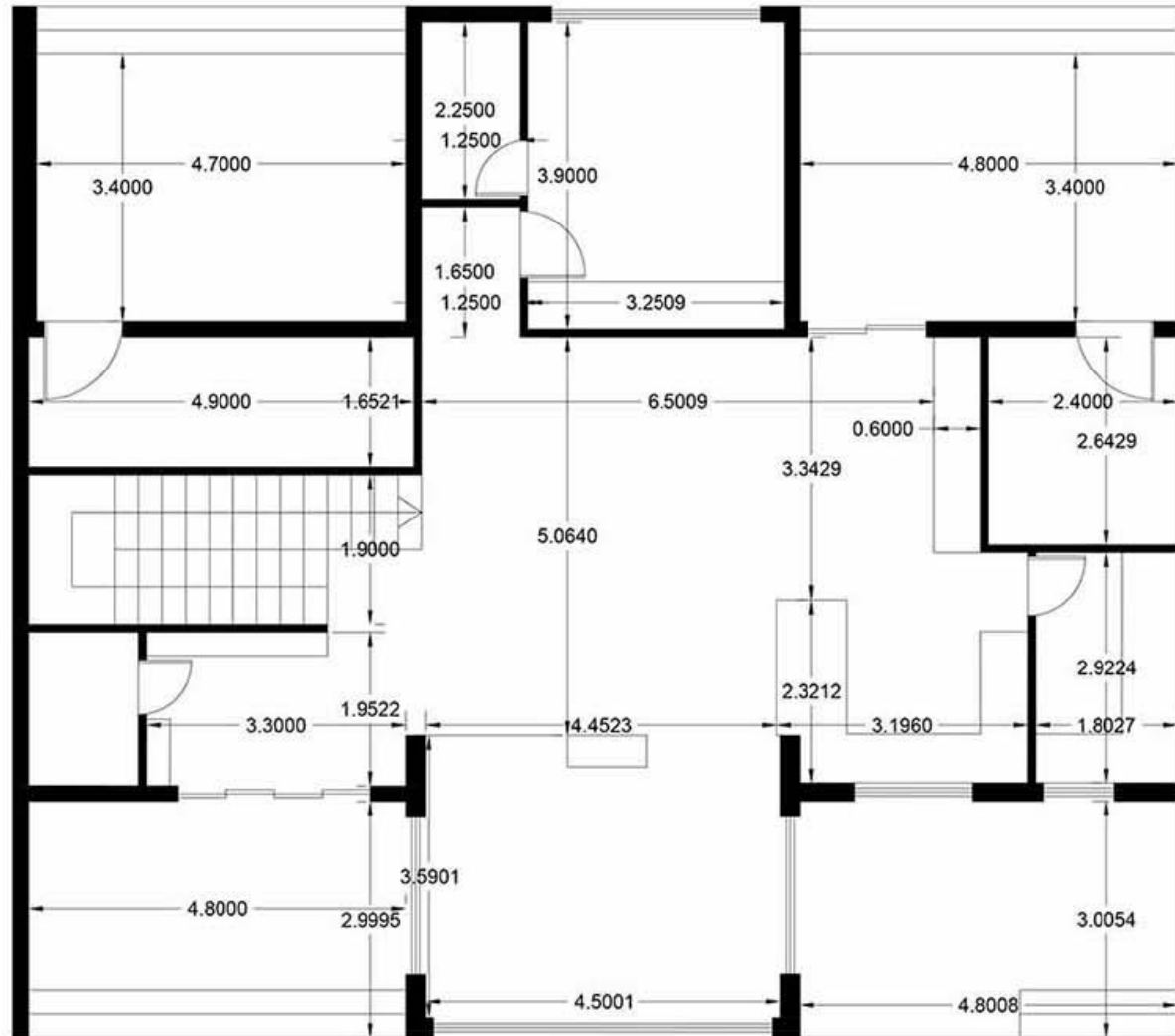
پلان اندازه گذاری طبقه همکف
