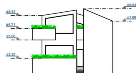
نمای غربی
