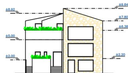
نمای شرقی
