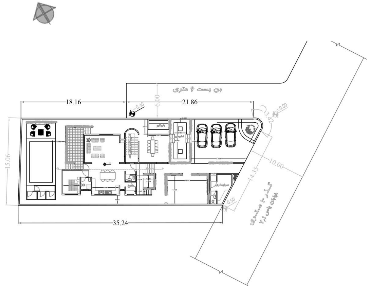
پلان همکف
