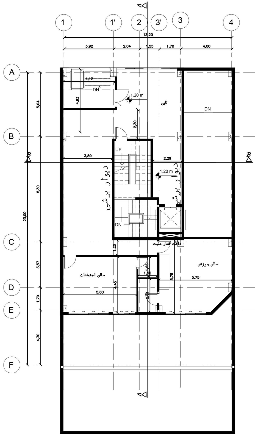
پلان طبقه همکف
