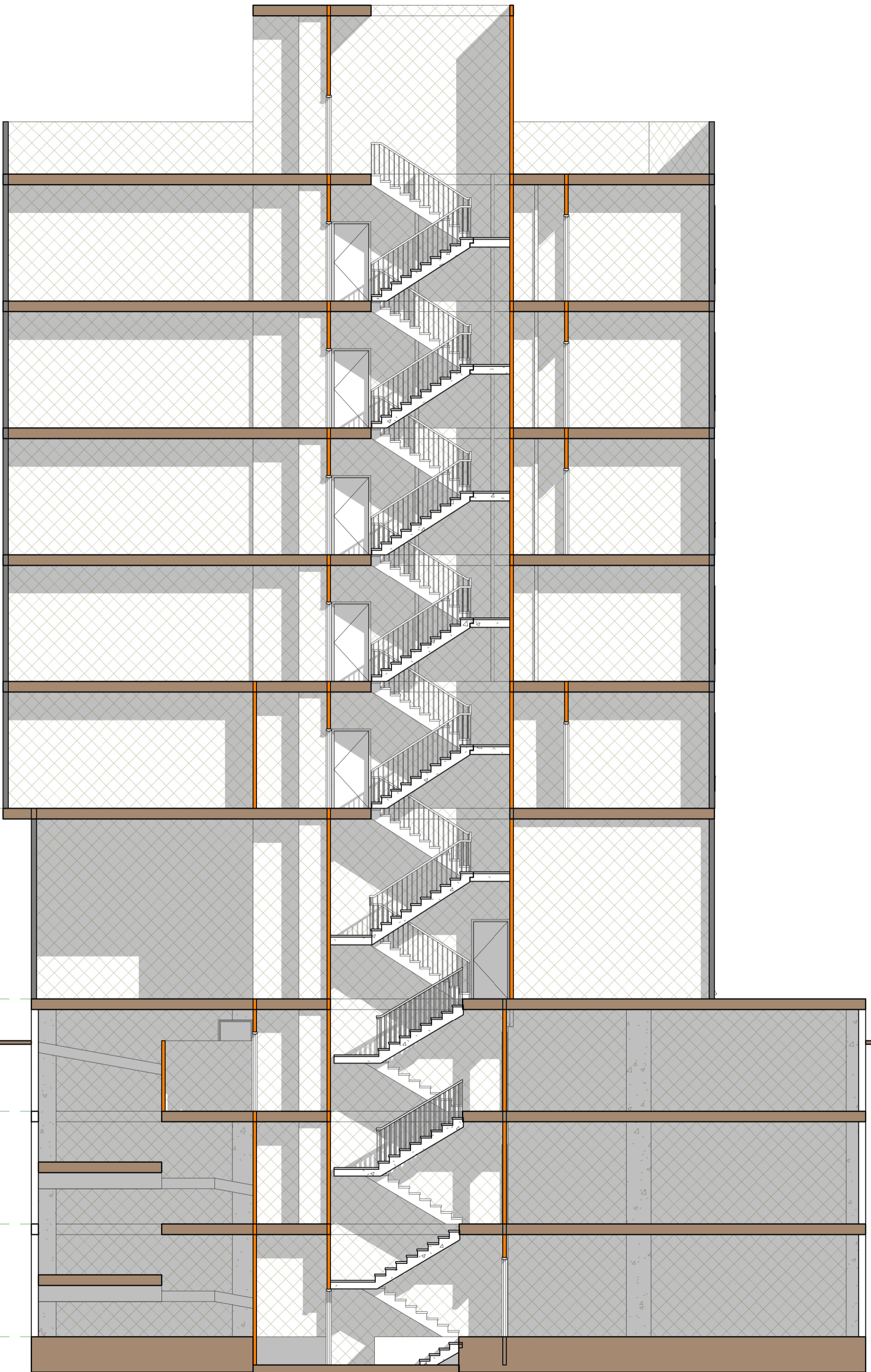
A-A Section Sc: 1/100
