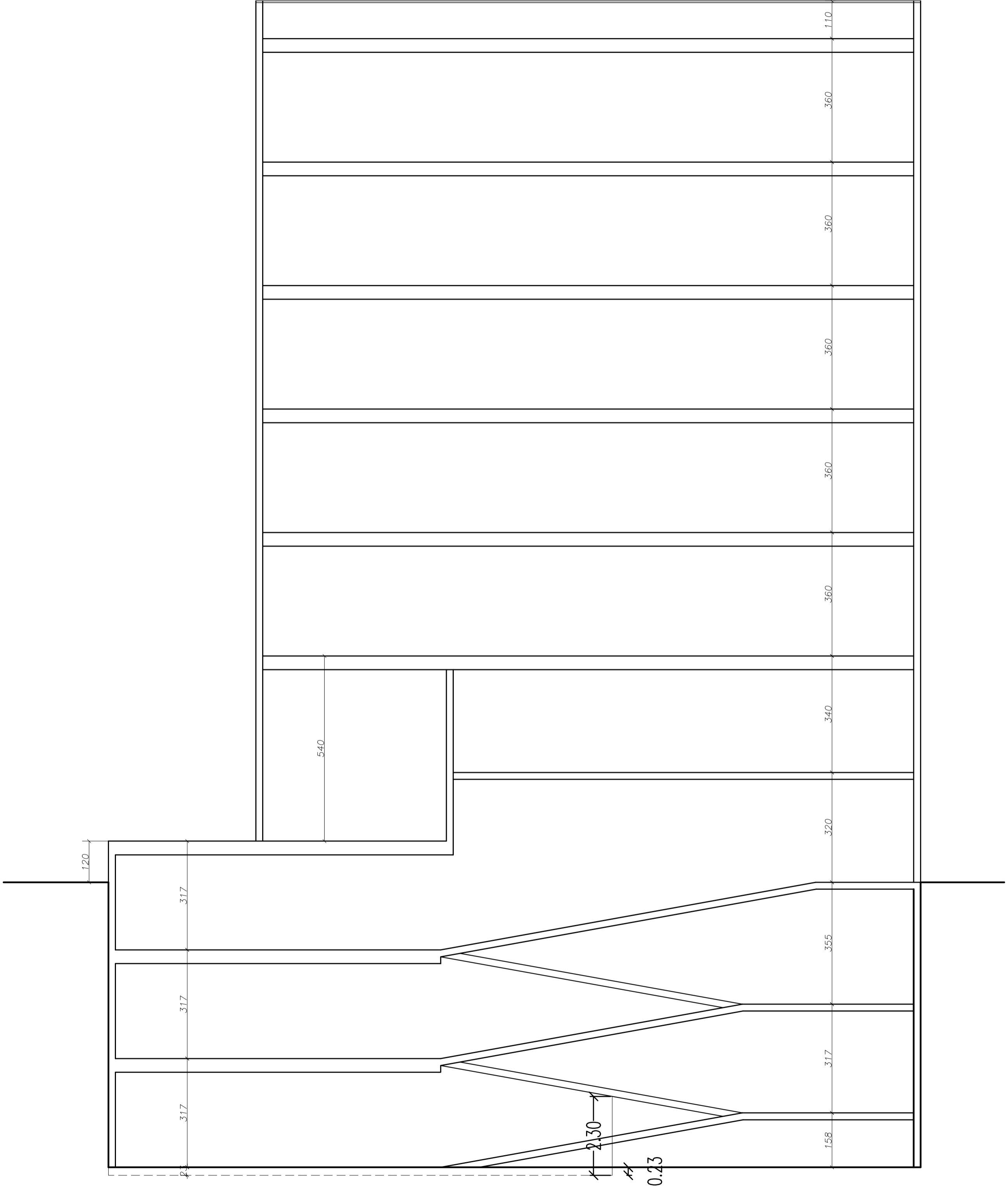
برش A-A SCALE 1:100
