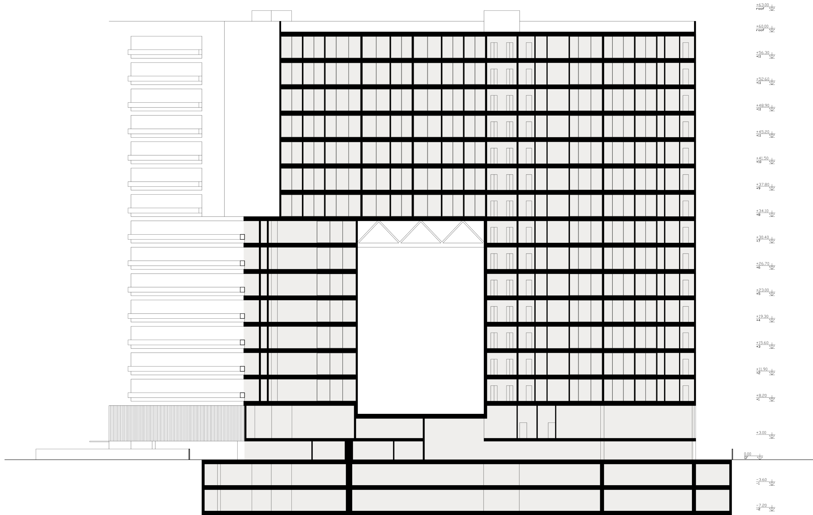
Section A-A
