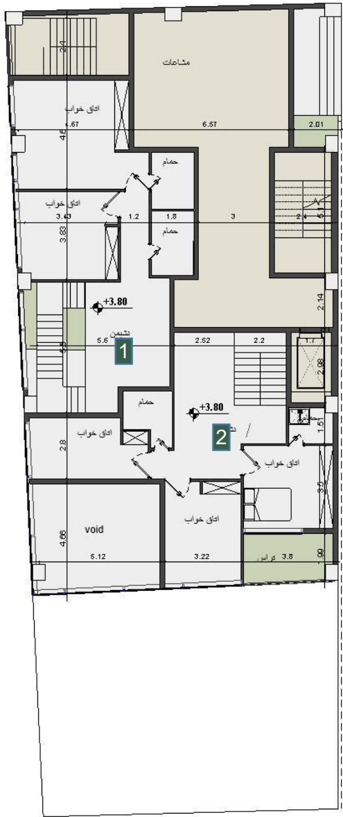
پلان اندازه گذاری نیم طبقه
