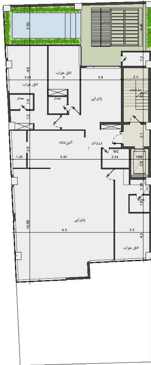
پلان اندازه گذاری طبقه ششم
