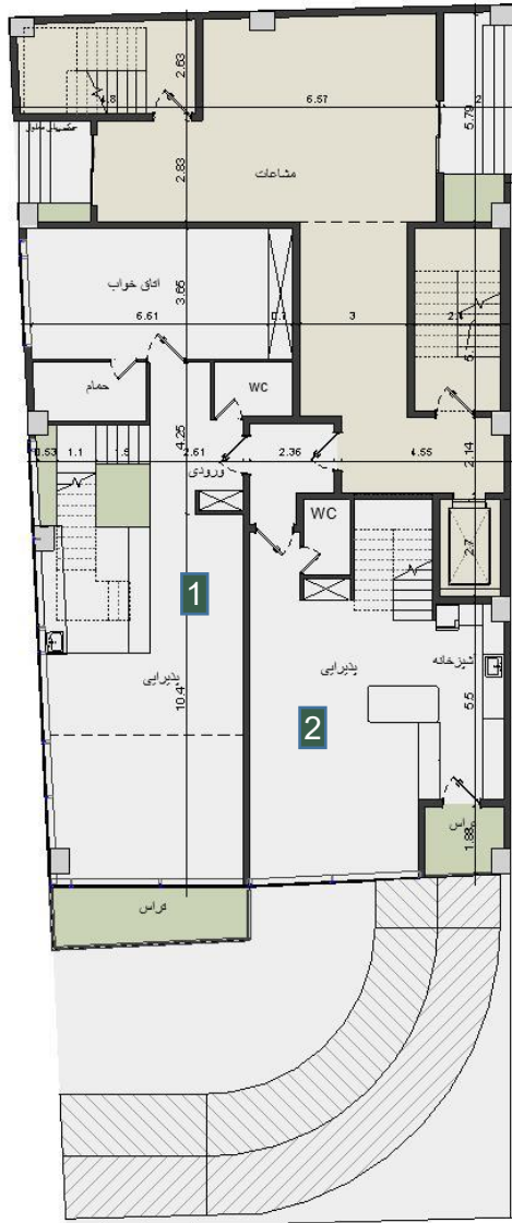
پلان اندازه گذاری همکف
