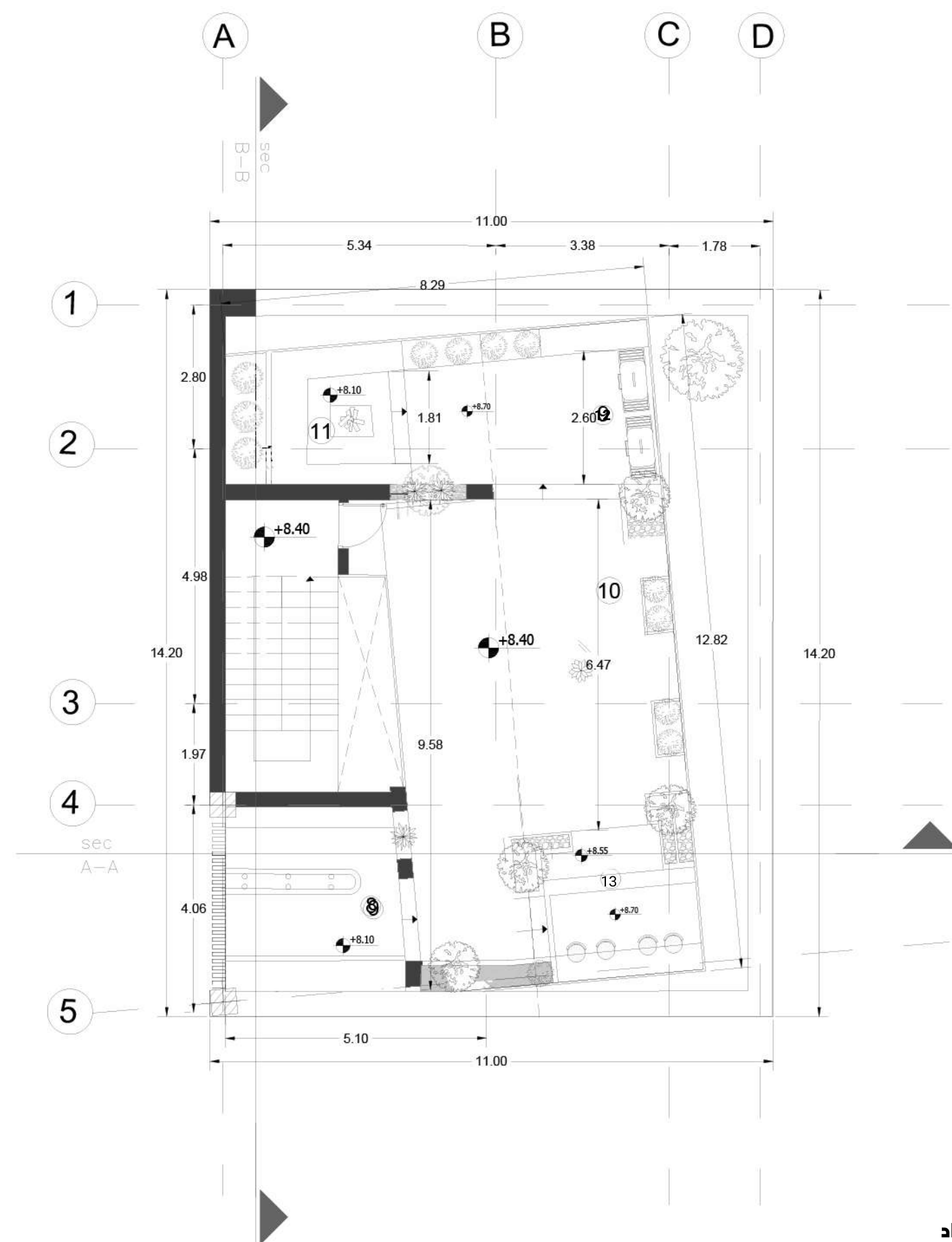
پلان اندازه گذاری روف گاردن
