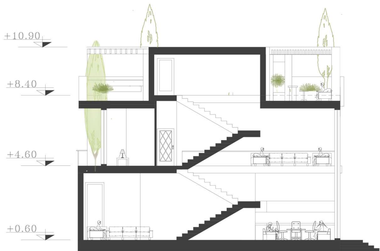
مقطع طولی B-B
