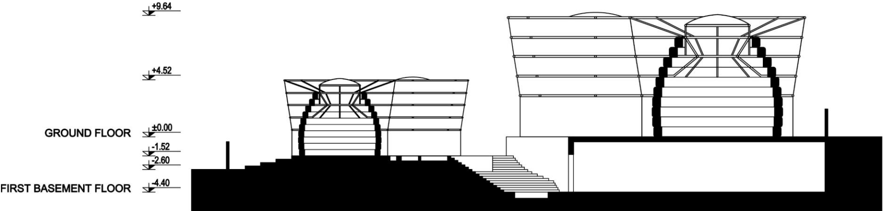
SECTION A-A
