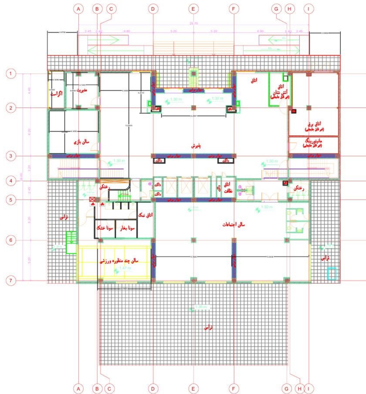
اندازه گذاری همکف
