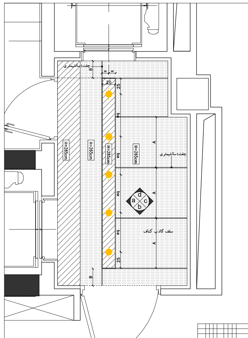
پلان سقف کاذب
