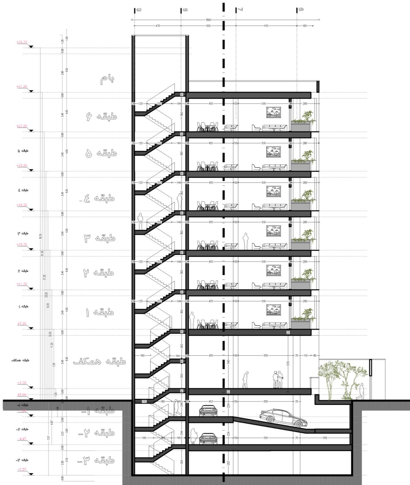
SECTION A-A
